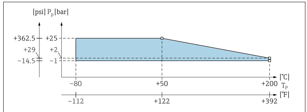
20 Diagrama de redução de pressão e temperatura para sondas de haste flexível sem comprimento inativo ou com comprimento inativo
