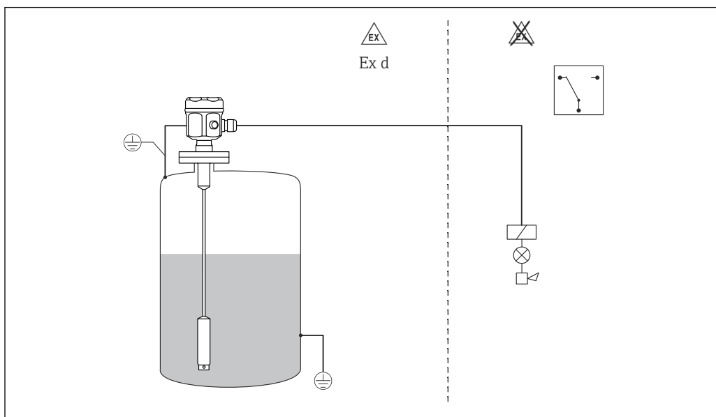
4 Sonda como interruptor de nivel puntual
