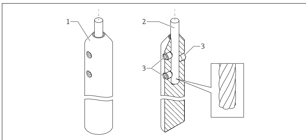
14 Visión general del contrapeso tensor
