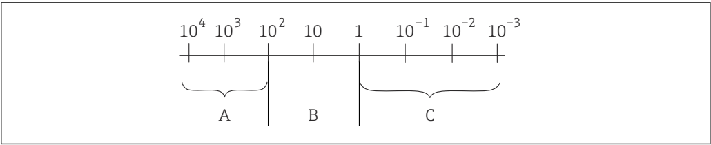
23 Rango operacional de la sonda. Unidad de medida: \mu S/cm
