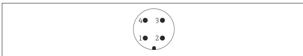
9 Conector M12 con módulo del sistema electrónico a 3 hilos FEI52, FEI53
