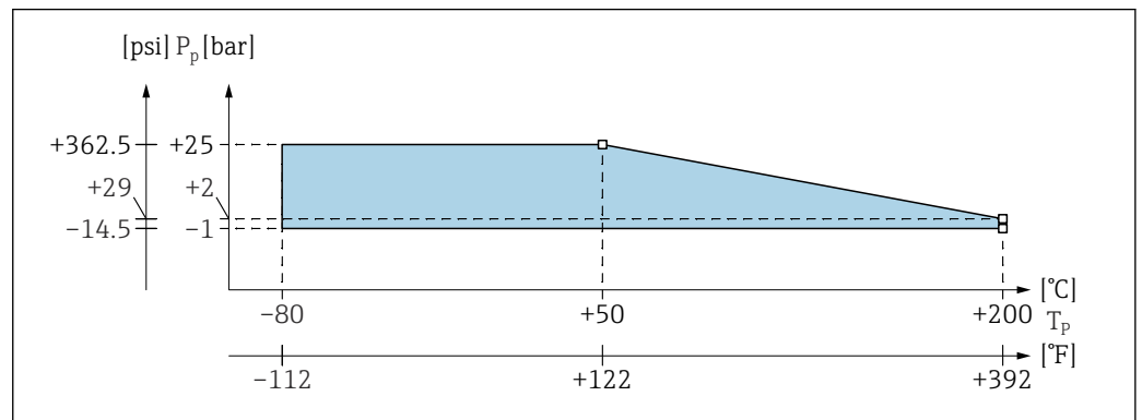
20 Diagrama de deriva de presión y temperatura para sondas de cable sin longitud inactiva o con longitud inactiva
