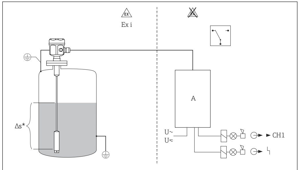
\Delta s Nur mit FEI53 A Messumformerspeisegerät
