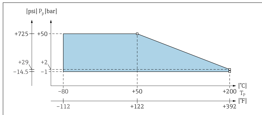
22 Grafik zum Druck- und Temperatur-Derating für vollisolierte Seilsonden mit inaktiver Länge
