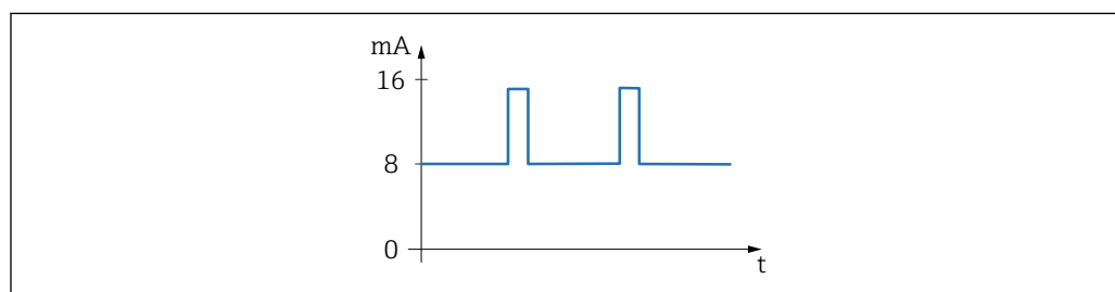
図 24 周波数 17~185 Hz の場合の PFM 信号
