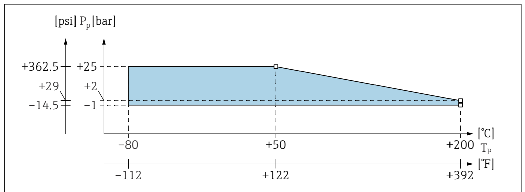
20 不感帯なし/不感帯付きローブプローブの圧力および温度ディレーティング図
