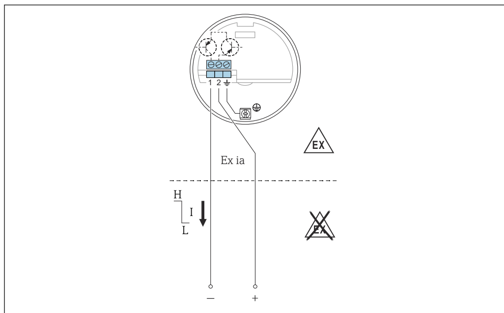
図 25 端子は、IEC 60947-5-6 (NAMUR) に準拠した変換器（絶縁アンプ）に接続してください
