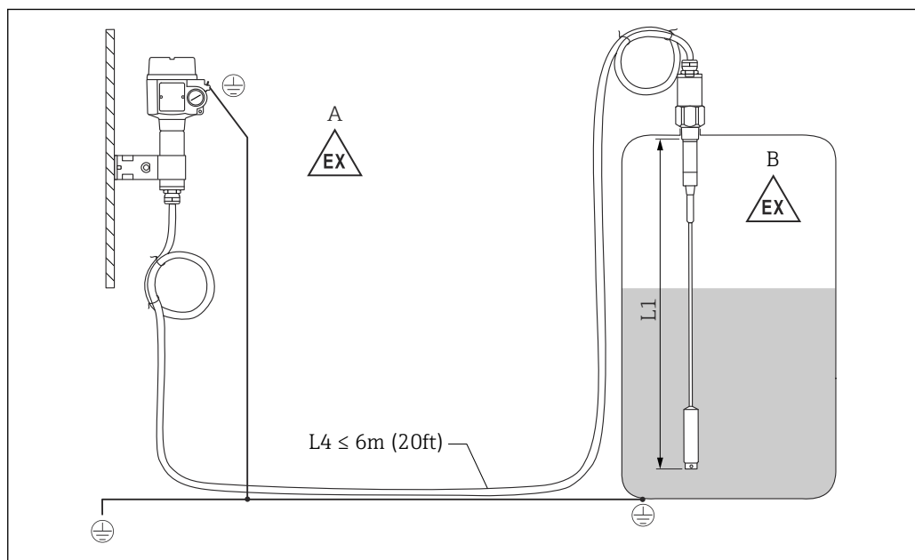
☑ 15 プローブと分離型ハウジングの接続。測定単位 mm (in)
