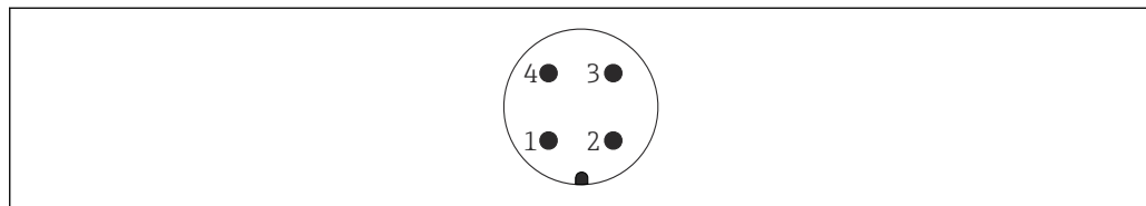
図 8 M12 コネクタ : 2 線式エレクトロニックインサート FEI55、FEI57、FEI58、FEI57C
