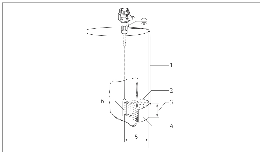
図 13 樹脂タンクへのプローブの取付け
