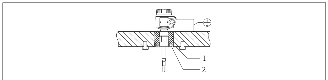
☑ 12 コンクリート製のサイロ壁への取付け：結露が発生する場合
