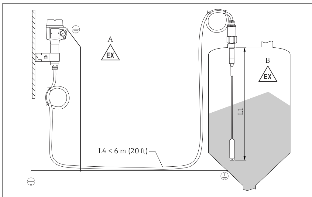
図 15 プローブと分離型ハウジングの接続
