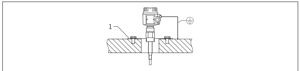
☑ 11 コンクリート製のサイロ壁への取付け
