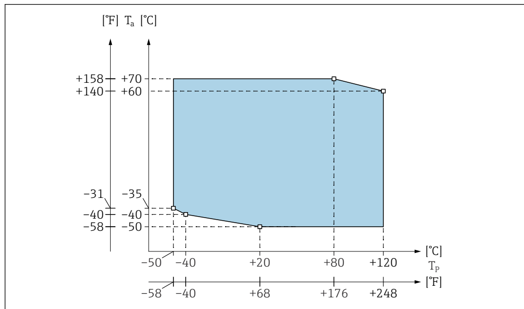
図 19 プロセス温度範囲図：完全絶縁プローブ
