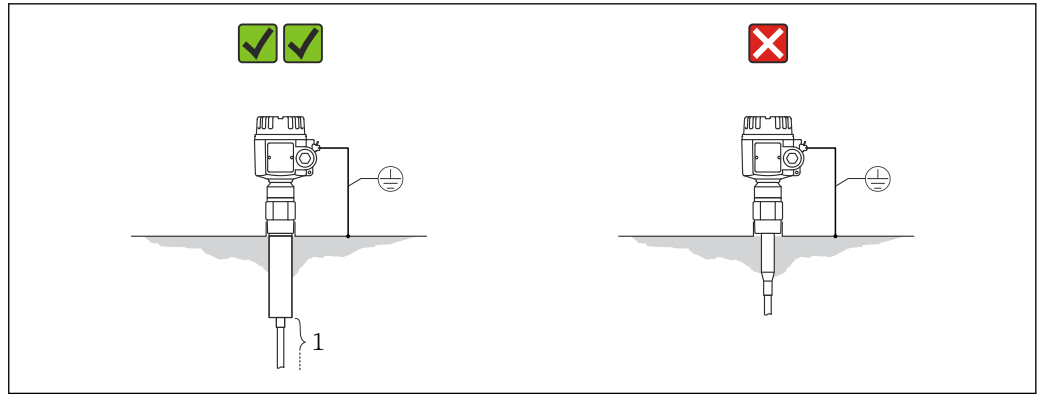
☑ 10 サイロの壁に導電性がある場合
