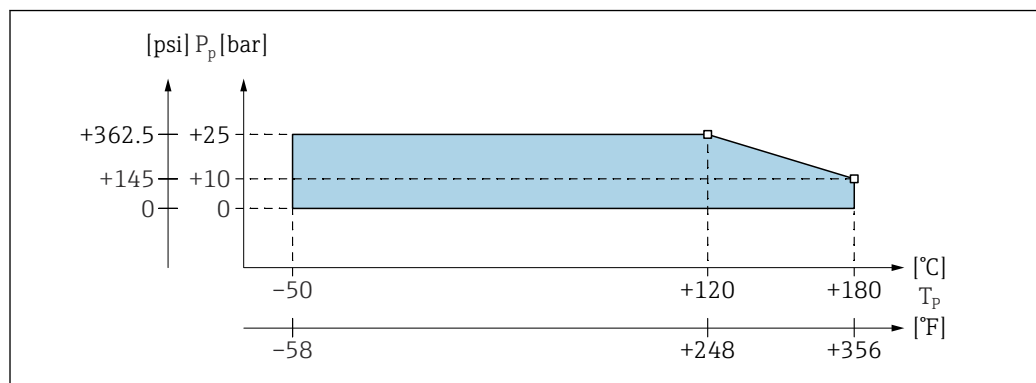
図 20 プロセス圧力と温度ディレーティングの図：部分絶縁プローブ
