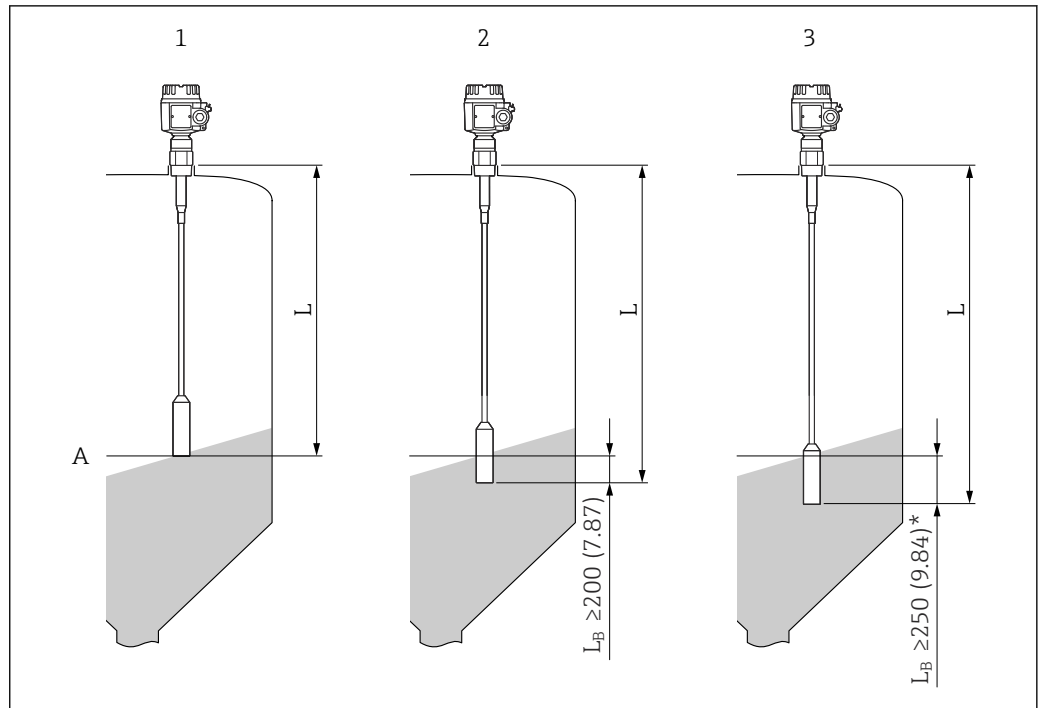
図 14 ロープ長と測定物の相関関係。測定単位 mm (in)
