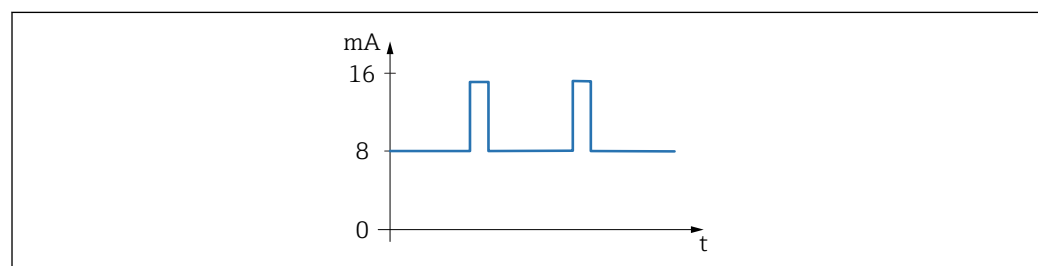
図 23 周波数 17~185 Hz の場合の PFM 信号
