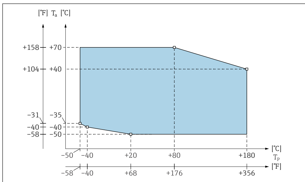
図 18 プロセス温度範囲図：部分絶縁プローブ
