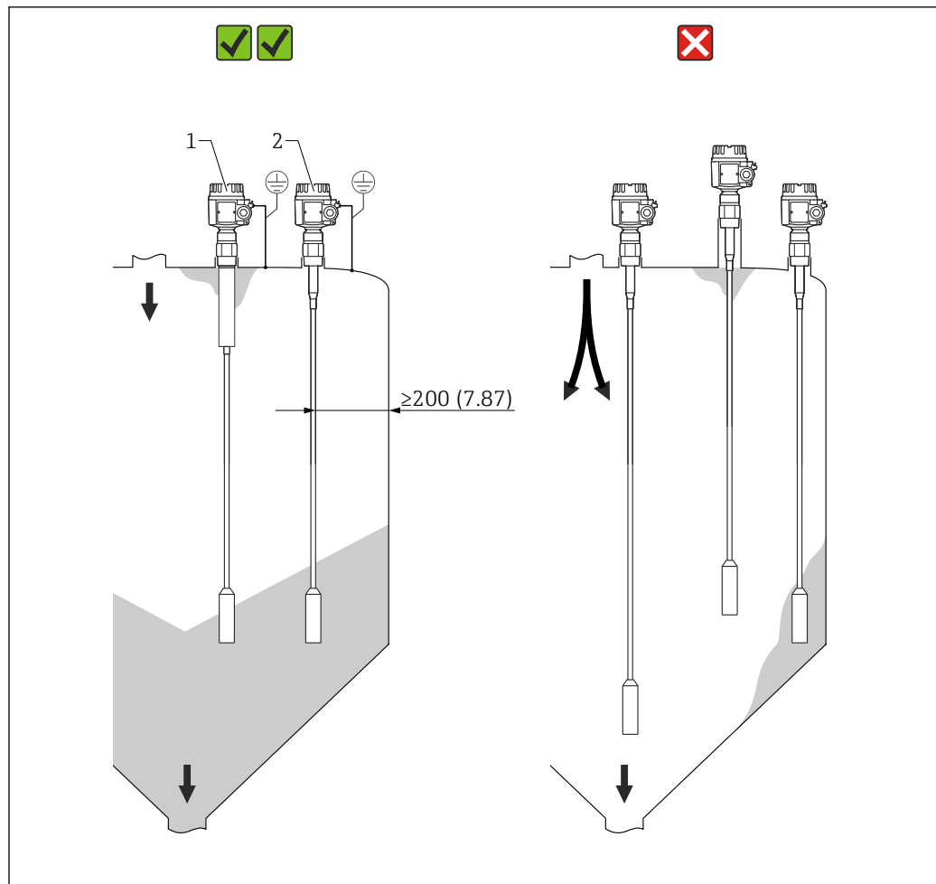
図 9 取付例。測定単位 mm (in)
