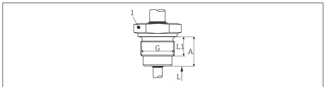
図 13 ISO 228 準拠ネジ、溶接アダプタ Liquiphant 用
