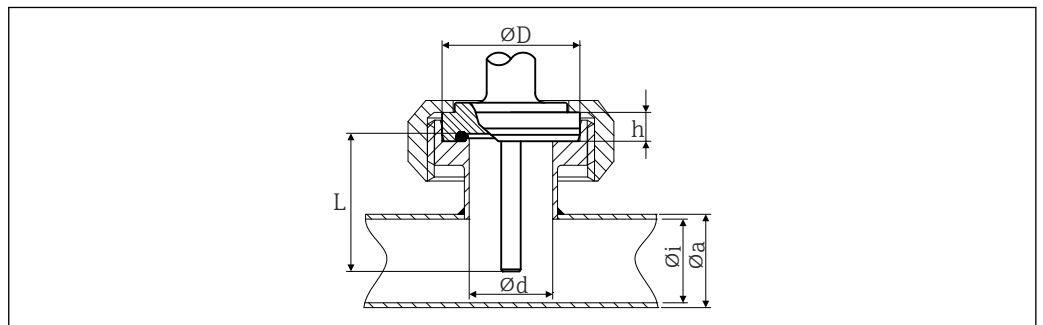
10 無菌配管接続 (DIN 11864-1 フォーム A 準拠)
