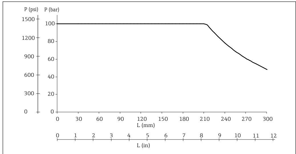
図 5 許容最大プロセス圧力
