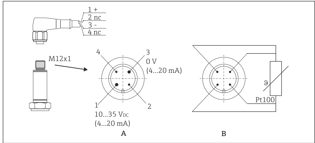
図2 機器プラグのピンの割当て
