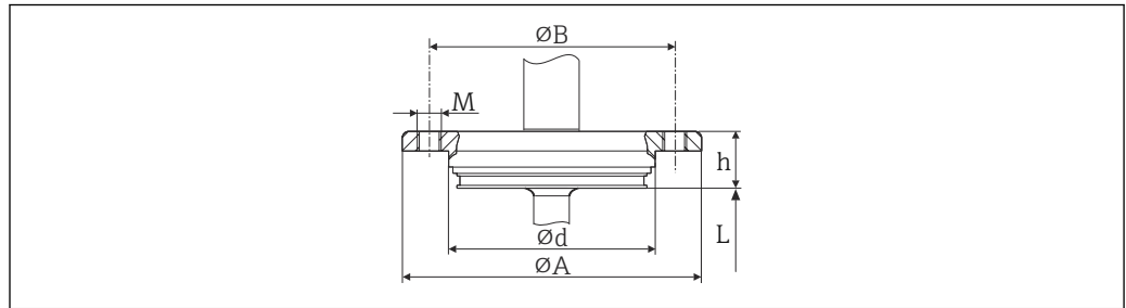
図 14 APV インライン
