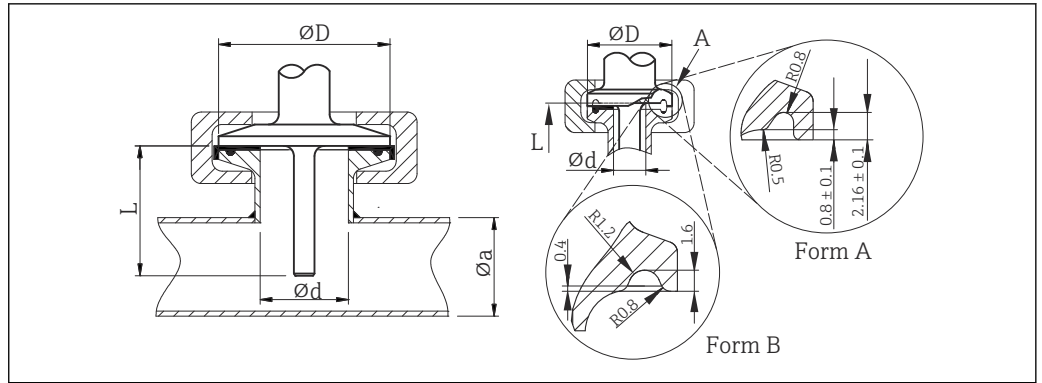
図 12 ISO 2852 準拠クランプ
