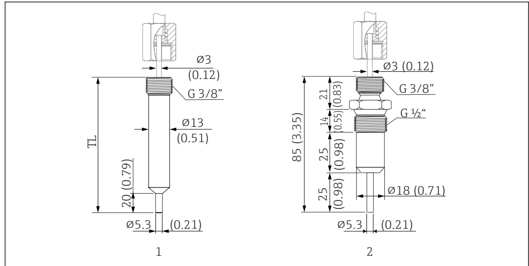
図 16 コンパクト温度計に接続するサーモウェル、バネ荷重袋ナットおよび G3/8" ネジ付き。寸法単位：mm (in)
