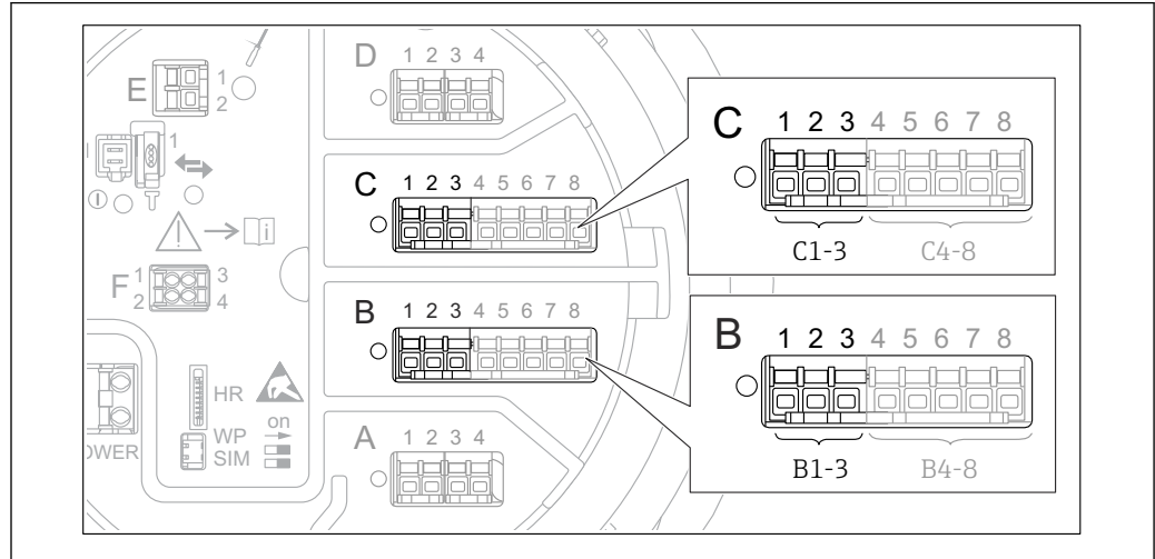
10 Klemmen für das Untermenü "Analog I/O" (→ 126) ("B1-3" bzw. "C1-3")
