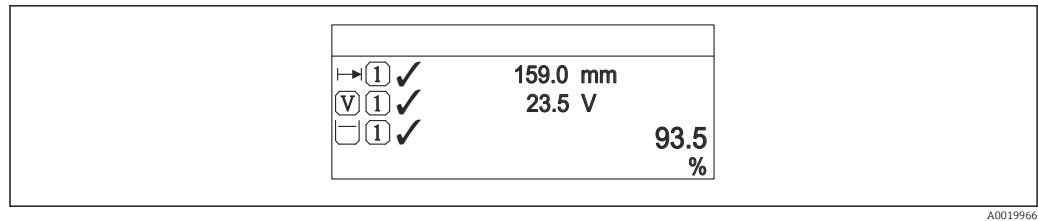
4 "Format Anzeige" = "1 Wert groß + 2 Werte"
