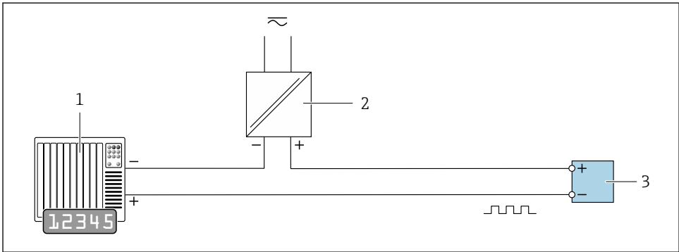
10 Ejemplo de conexión para salida de pulsos/frecuencia (pasiva)
