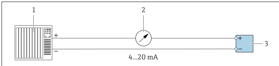
▣ 5 Пример подключения для токового выхода 4–20 мА (активного)
