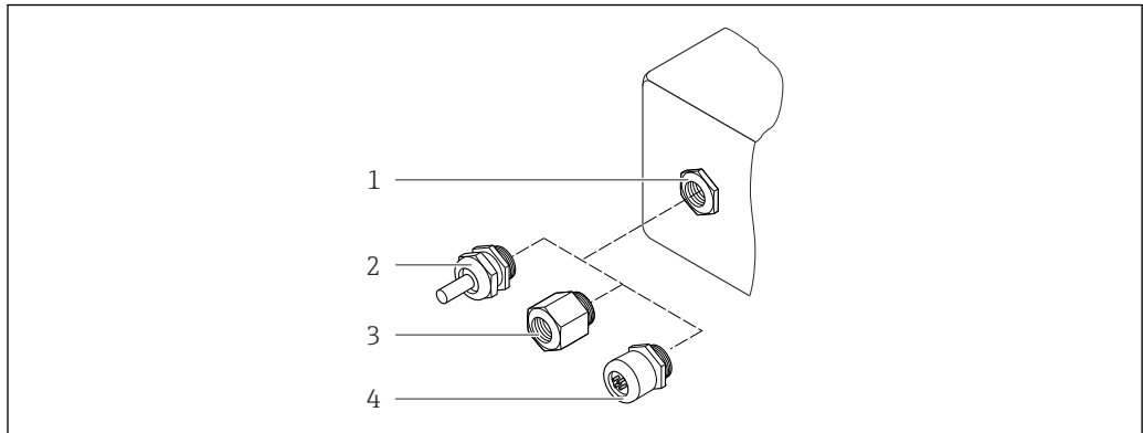
31 Possíveis entradas para cabo/prensa-cabos
