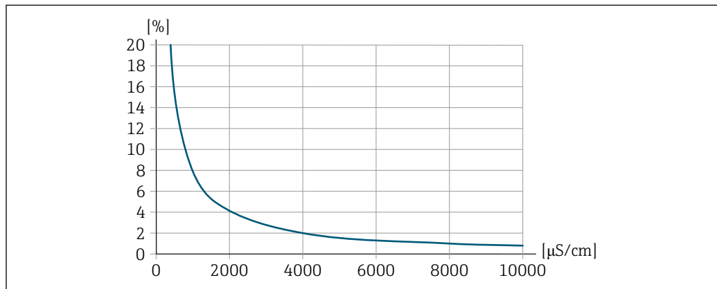
30 Repetibilidade em % do valor medido - condutividade elétrica [µS/cm]
