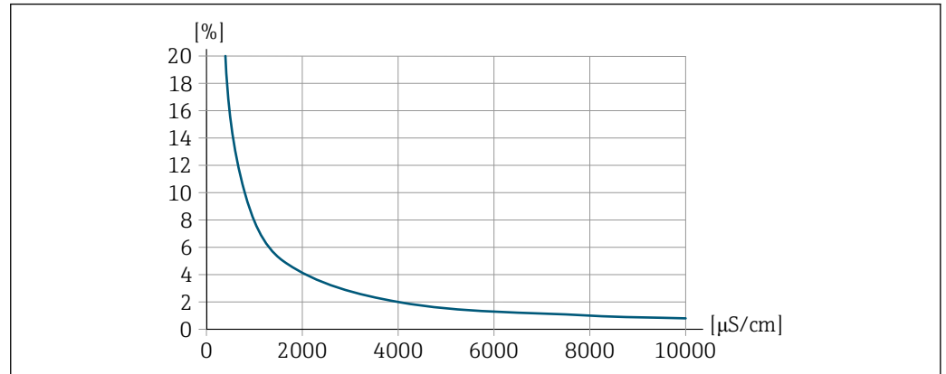
图 35 重复性 (测量值百分比) - 电导率 [μS/cm]
