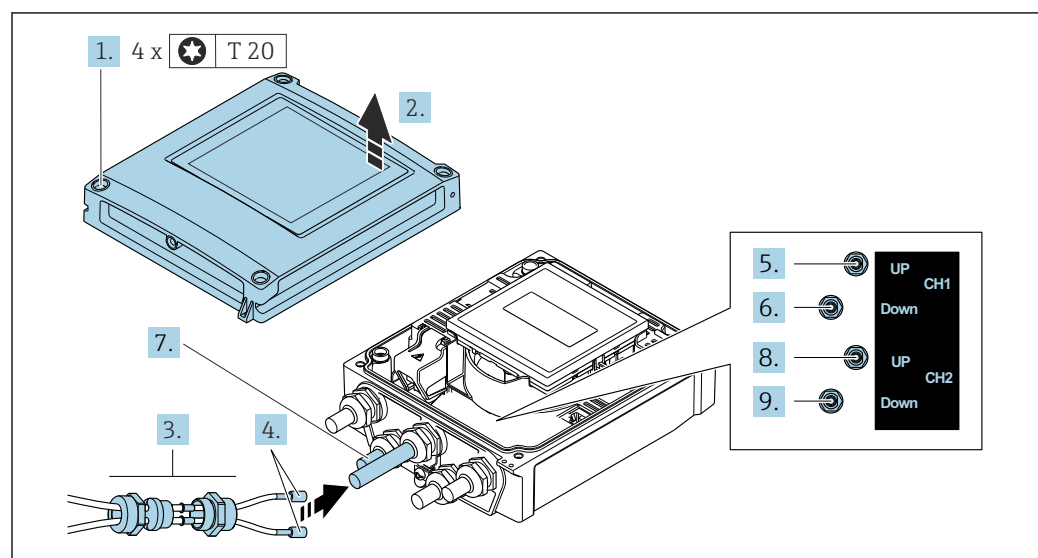
12 Messumformer: Hauptelektronikmodul mit Anschlussklemmen
