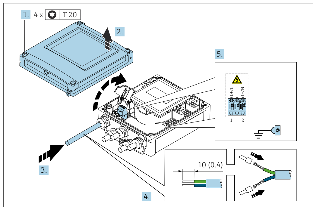
13 Anschluss Versorgungsspannung und 0-20 mA/4-20 mA HART mit weiteren Aus- und Eingängen
