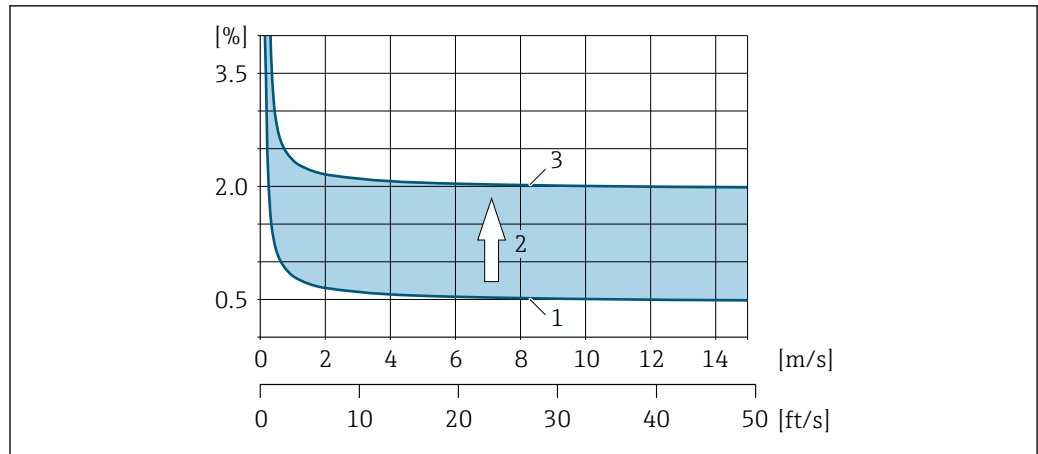
30 Beispiel für die Messabweichung in einer Rohrleitung mit Nennweite DN > 200 (8")
