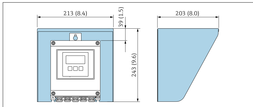
8 Wetterschutzhaube; Maßeinheit mm (in)
