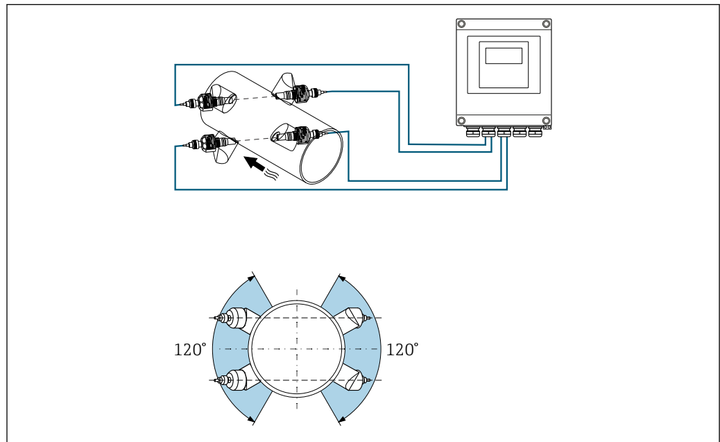
7 Zweipfad-Messung: Beispiel für die horizontale Anordnung der Sensorsets an einer Messstelle
