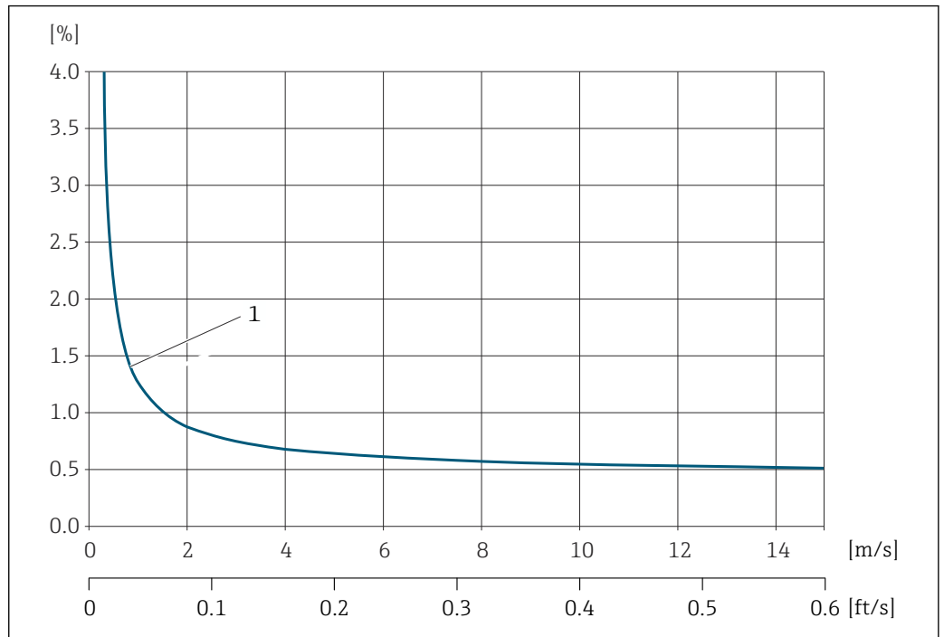
31 Beispiel maximale Messabweichung (Volumenfluss) in % v.M.
