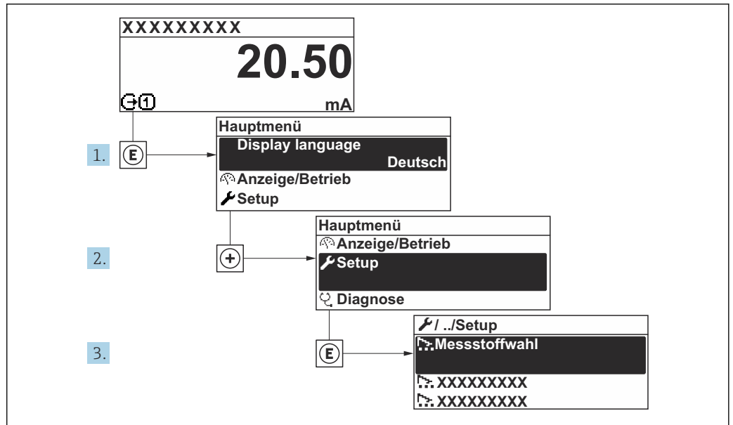
23 Navigation zum Menü "Setup" am Beispiel der Vor-Ort-Anzeige
