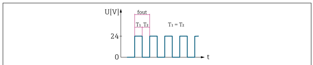
7 Durchflussproportionaler Frequenzgang
