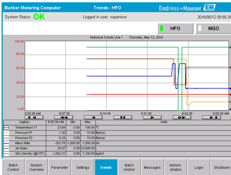
14 Окно «Trends»
