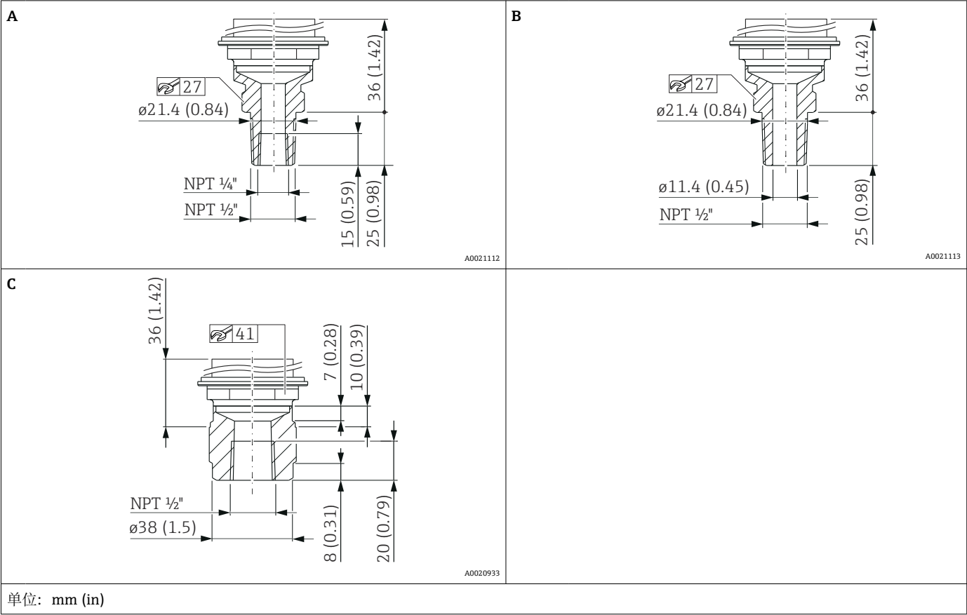
ASME B1.20.1 螺纹过程连接，内置膜片（不带隔膜密封系统的标准型仪表）
