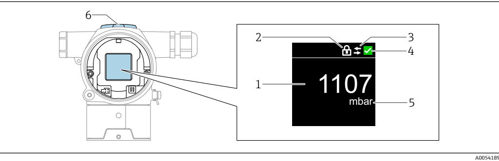
图 2 彩色显示单元 1 测量值（最多 5 位） 2 锁定（仪表锁定时显示此图标） 3 HART 通信状态（HART 通信开启时显示此图标） 4 状态图标，符合 NAMUR 标准 5 电流输出测量值（百分比单位） 6 磁性按钮（零点和量程）
