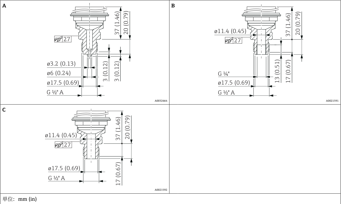
ISO 228 G 螺纹过程连接，内置膜片（不带隔膜密封系统的标准型仪表）
