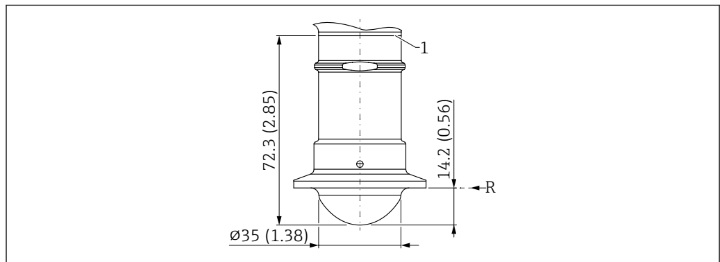
图 20 外形尺寸示意图; Tri-Clamp NA Connect ISO2852 DN25-38 (1½)过程连接, 工作频率 80 GHz; PTFE
