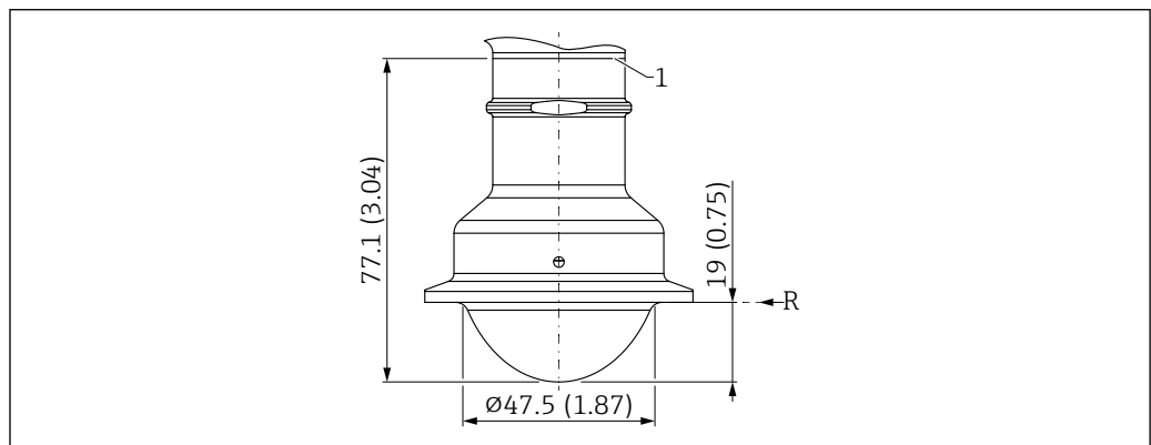
图 21 外形尺寸示意图; Tri-Clamp NA Connect ISO2852 DN40-51 (2)过程连接, 工作频率 80 GHz; PTFE
