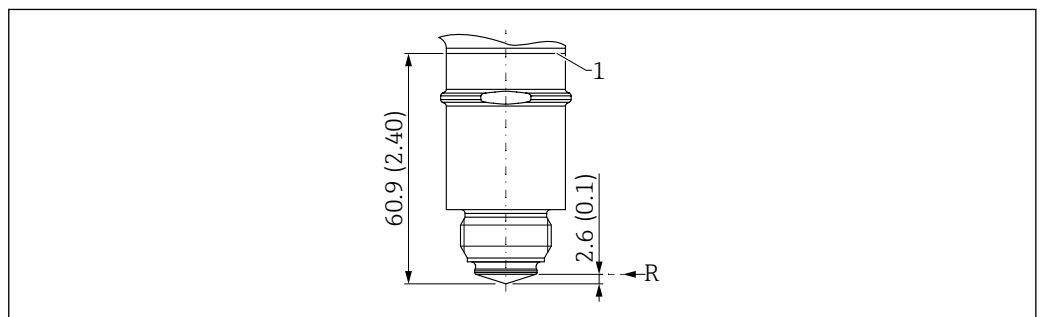
18 外形尺寸示意图; M24 过程连接, 工作频率 80 GHz; PEEK
