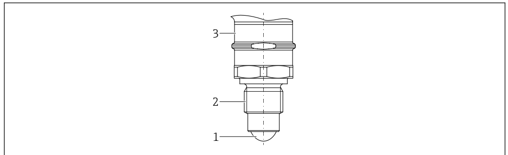
☐ 26 材质组成; G½过程连接, 工作频率 180 GHz; PTFE
