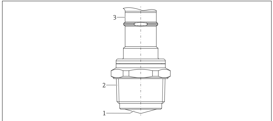
☐ 25 材质组成; MNPT1½过程连接, 工作频率 80 GHz; PEEK
