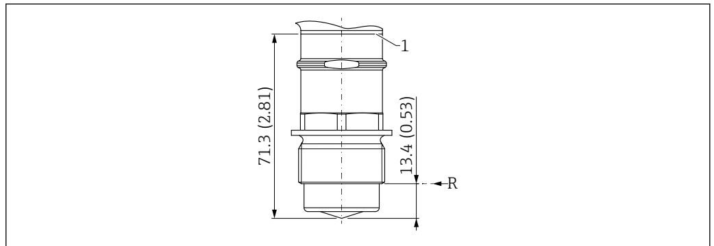
16 外形尺寸示意图; G 1 过程连接, 工作频率 80 GHz; PEEK
