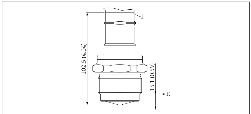
17 外形尺寸示意图; G 1½ 过程连接, 工作频率 80 GHz; PEEK
