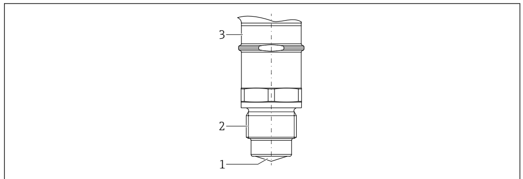
☐ 27 材质组成; G¾过程连接, 工作频率 80 GHz; PEEK
