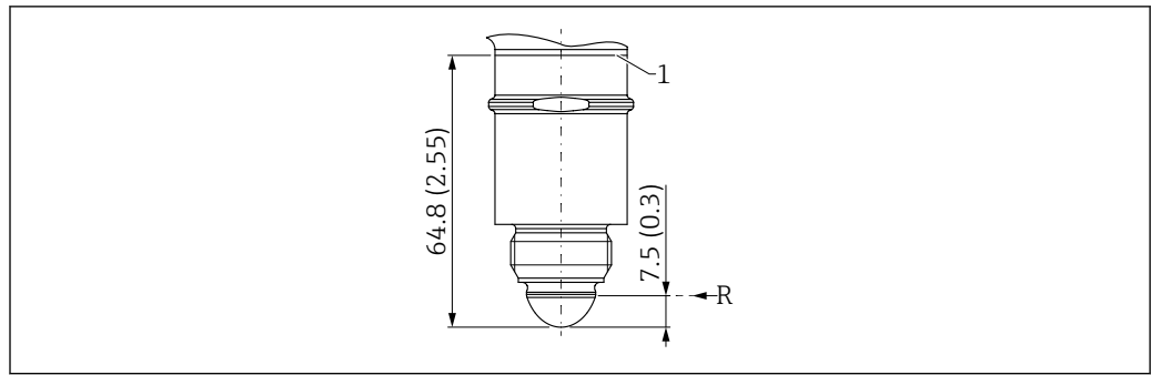
图 19 外形尺寸示意图; M24 过程连接, 工作频率 180 GHz; PTFE
