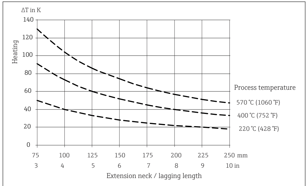
12 Erwärmung des Anschlusskopfes in Abhängigkeit von der Prozesstemperatur. Temperatur im Anschlusskopf = Umgebungstemperatur 20 °C (68 °F)+ ΔT
