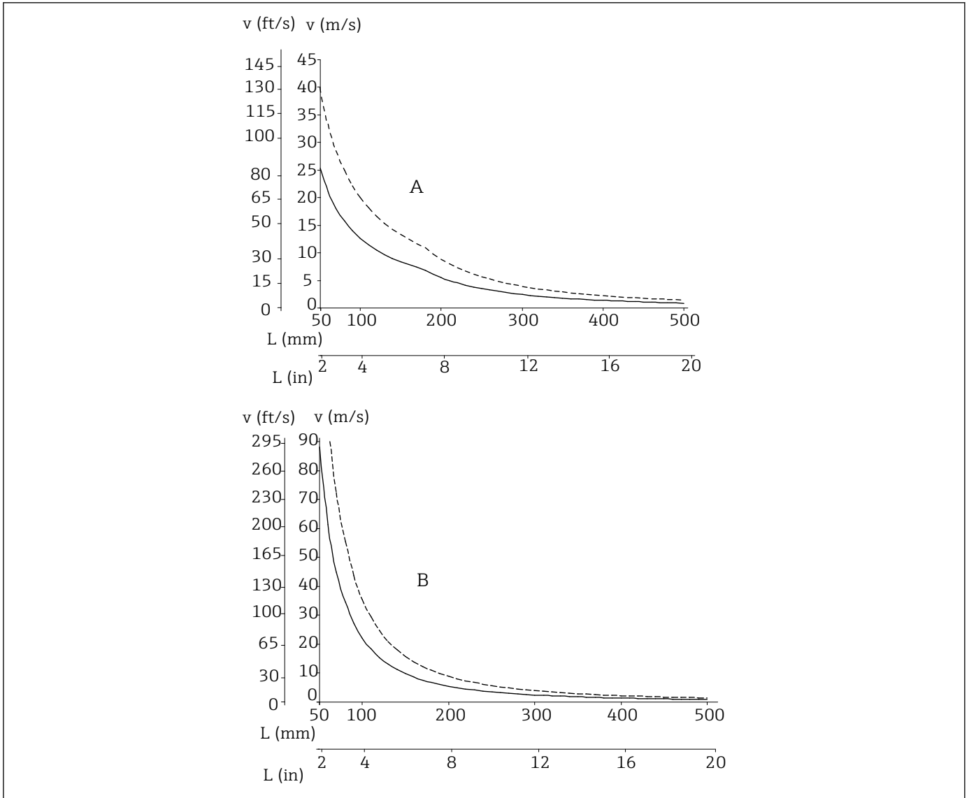
9 Maximale Anströmgeschwindigkeit bei Schutzrohrdurchmesser 9 mm (0,35 in) (——) oder 12 mm (0,47 in) (----)
