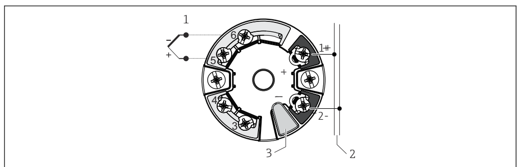
11 Im Anschlusskopf montierter Transmitter TMT7x (ein Sensoreingang)
