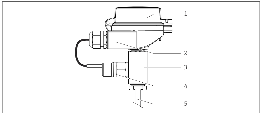
30 Halsrohr mit zweiter Prozessbarriere
