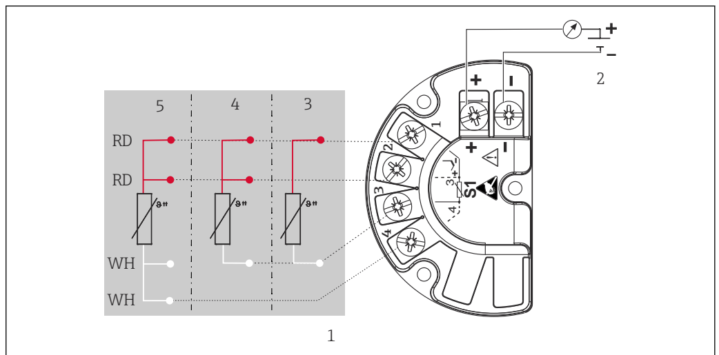
8 TMT142B (ein Sensoreingang)
