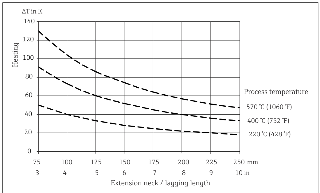
29 Erwärmung des Anschlusskopfes in Abhängigkeit von der Prozesstemperatur. Temperatur im Anschlusskopf = Umgebungstemperatur 20 °C (68 °F) + ΔT
