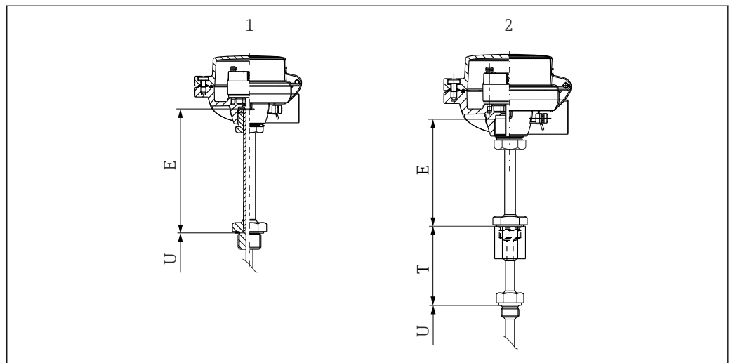
1 Abnehmbares Halsrohr - Thermometer ohne Schutzrohr
