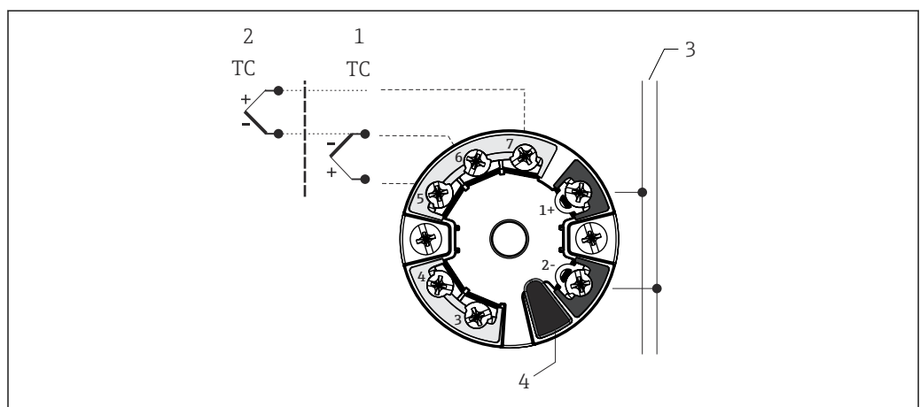
10 Im Anschlusskopf montierter Transmitter TMT8x (doppelter Sensoreingang)
