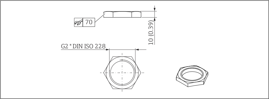
32 Medidas de la tuerca de seguridad. Unidad de medida mm (in)
