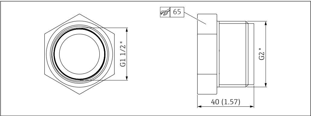
33 Medidas del adaptador Uni
