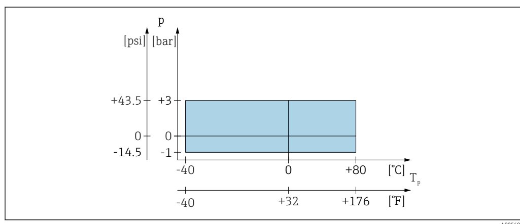
20 Rango admisible para la temperatura y la presión de proceso
