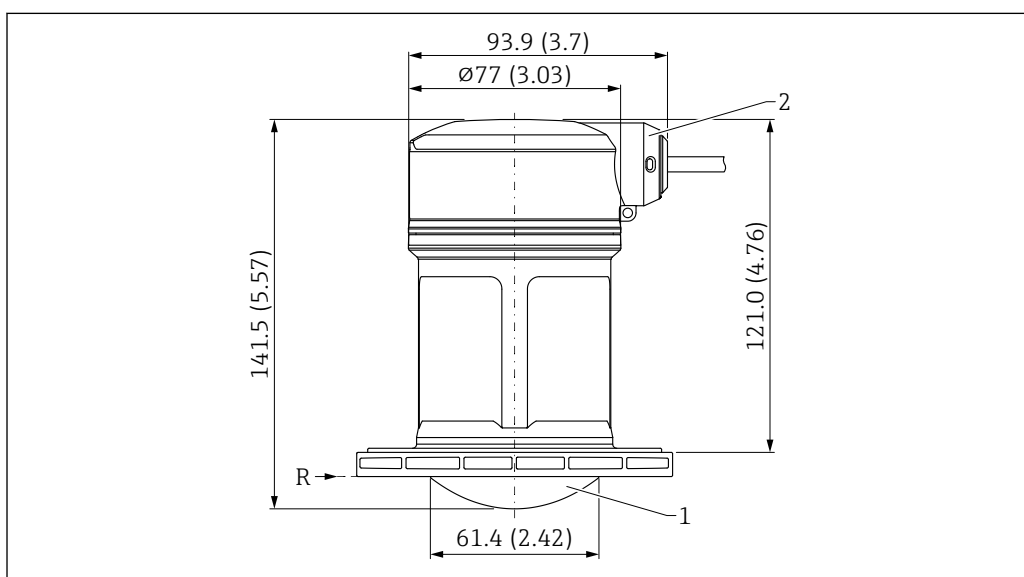
24 Medidas; antena de 80 mm (3 in) con entrada de cable en el costado
