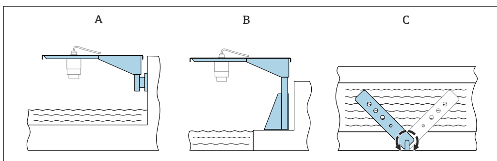
18 Instalación del soporte voladizo, con pivote
