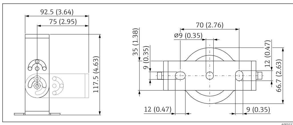
38 Dimensiones del soporte de montaje. Unidad de medida mm (in)
