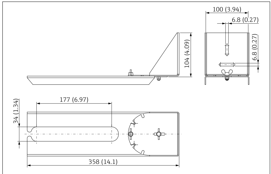
51 Dimensiones del soporte de montaje pivotante. Unidad de medida mm (in)
