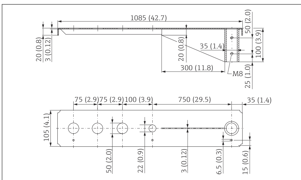
47 Medidas del soporte voladizo de 1 000 mm con pivote, para conexión a proceso de extremo de antena de sensor G 1½". Unidad de medida mm (in)
