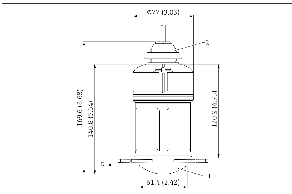
23 Medidas; antena de 80 mm (3 in) con entrada de cable desde arriba. Unidad de medida mm (in)
