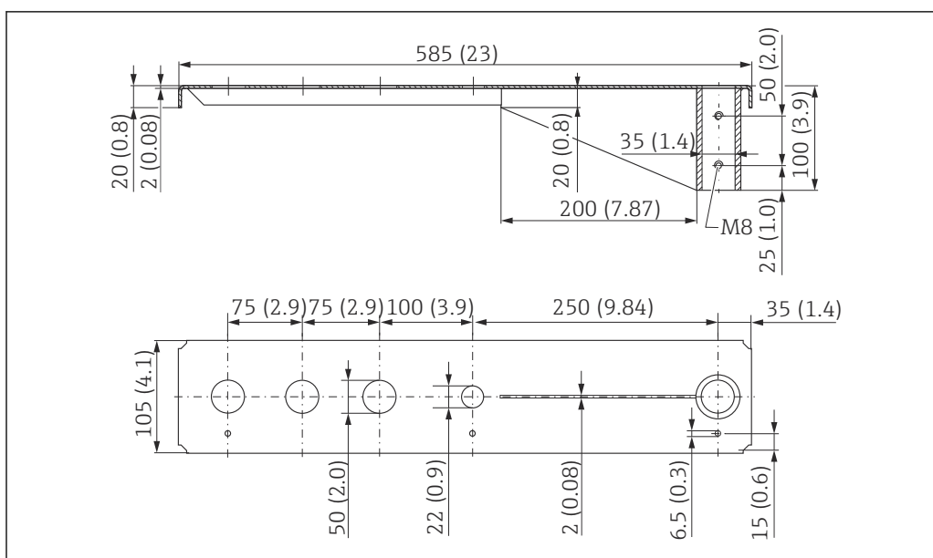
46 Medidas del soporte voladizo de 500 mm con pivote, para conexión a proceso de extremo de antena de sensor G 1½". Unidad de medida mm (in)
