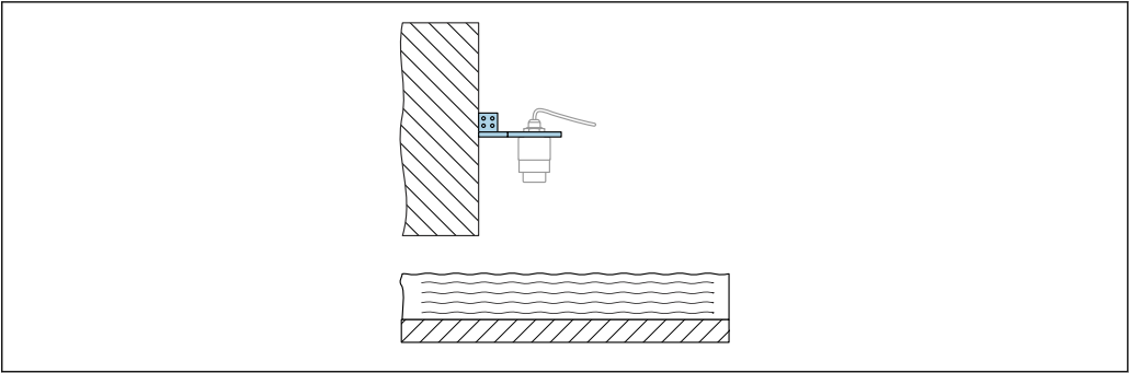
19 Soporte voladizo pivotante y ajustable con placa de montaje en pared (p. ej., para alinear el equipo con el centro de un aforador)
