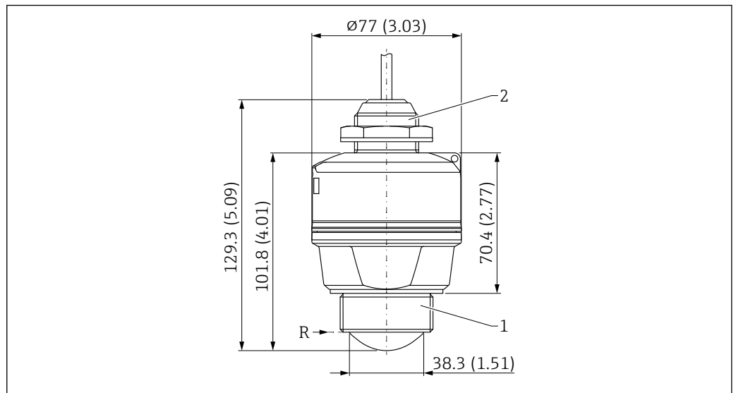
21 Medidas; antena de 40 mm (1,5 in) con entrada de cable desde arriba. Unidad de medida mm (in)
