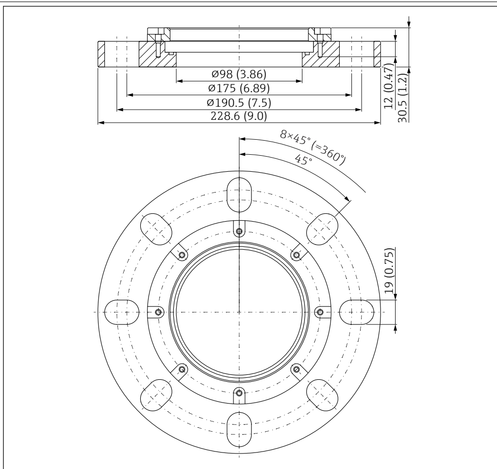
54 Medidas de brida deslizando UNI 4"/DN100/100. Unidad de medida mm (in)
