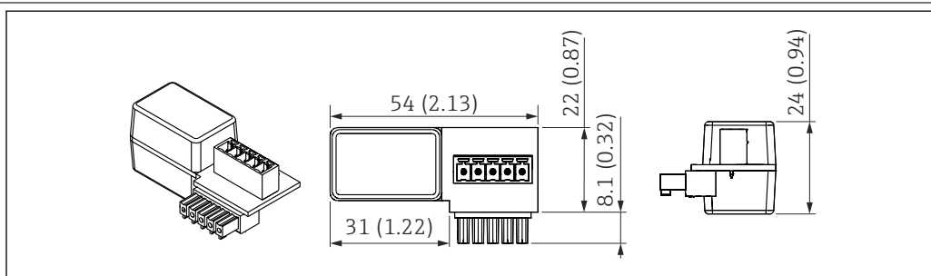
61 Medidas de la resistencia para comunicaciones HART. Unidad de medida mm (in)
