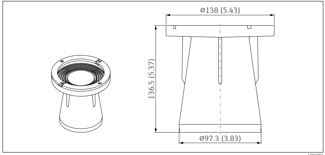
36 Medidas del tubo de protección contra desbordes 80 mm (3 in). Unidad de medida mm (in)
