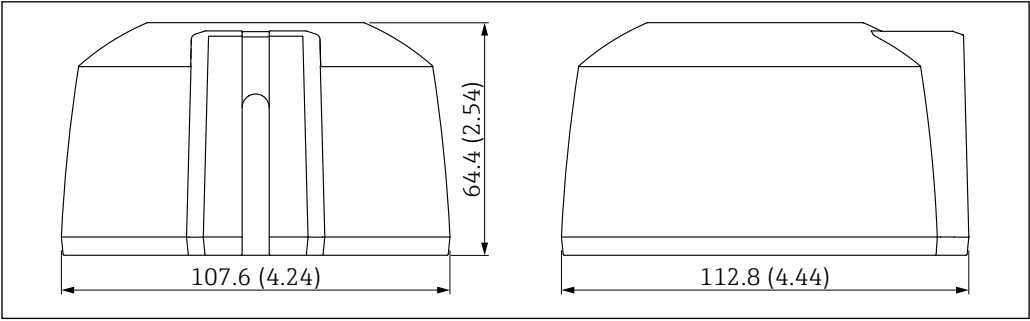
30 Medidas de la cubierta protectora con la entrada de cable en el costado. Unidad de medida mm (in)
