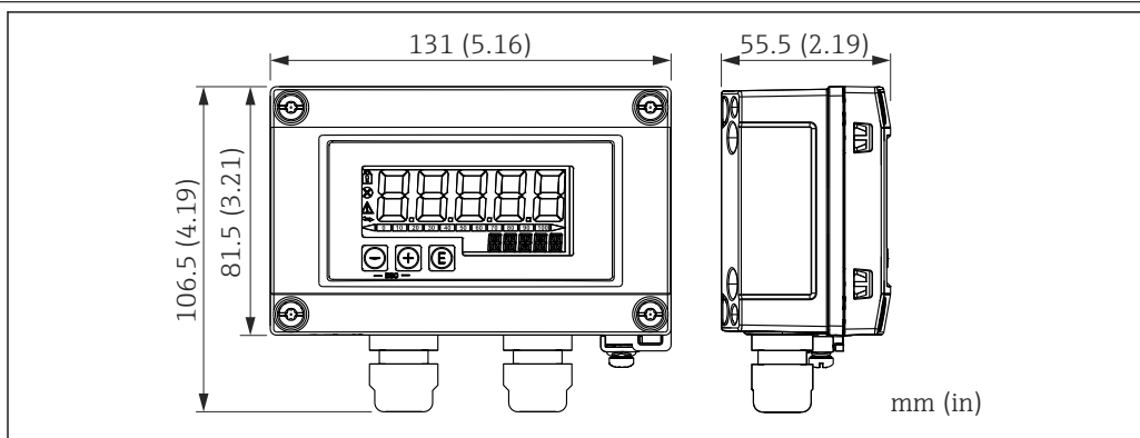
60 Medidas del RIA15 en la caja para montaje en campo. Unidad de medida mm (in)
