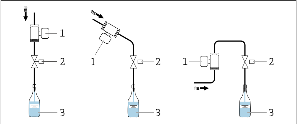
图 2 灌装系统
