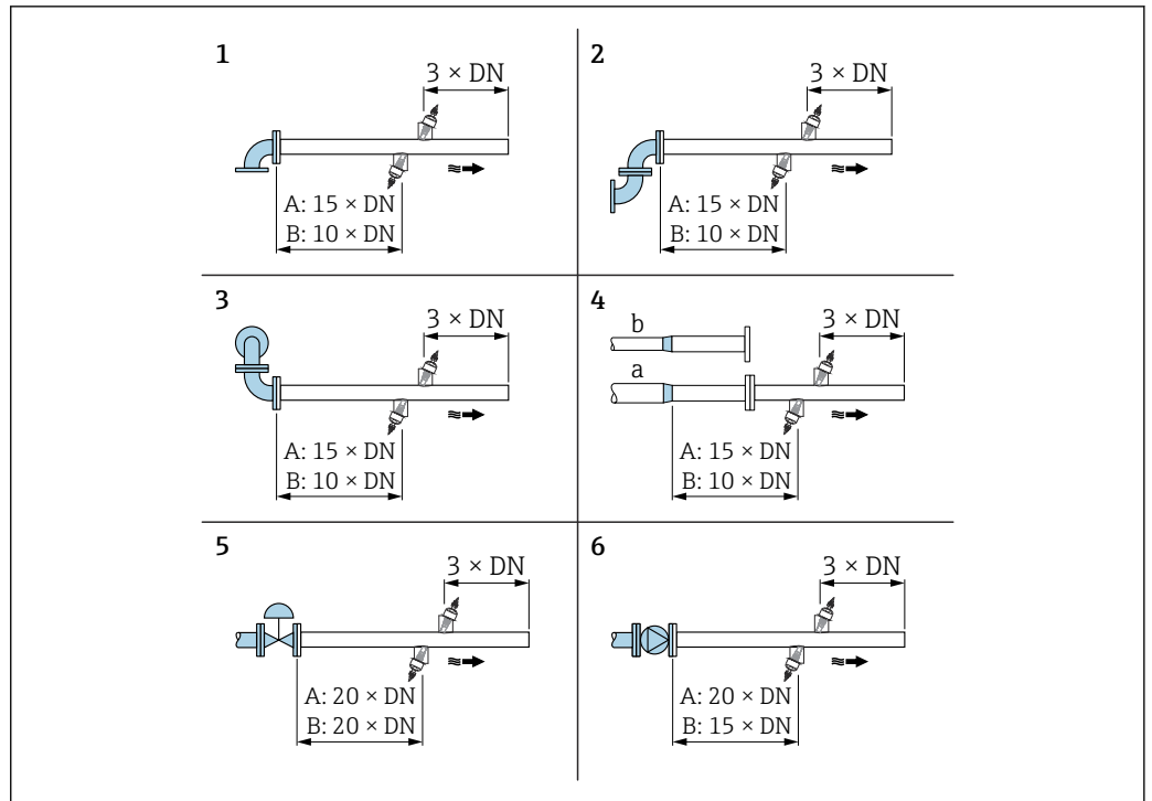
図 6 障害物が存在する場合の上流側/下流側の必要直管長 (A : 1 パス計測、B : 2 パス計測) (DN : 配管径)
