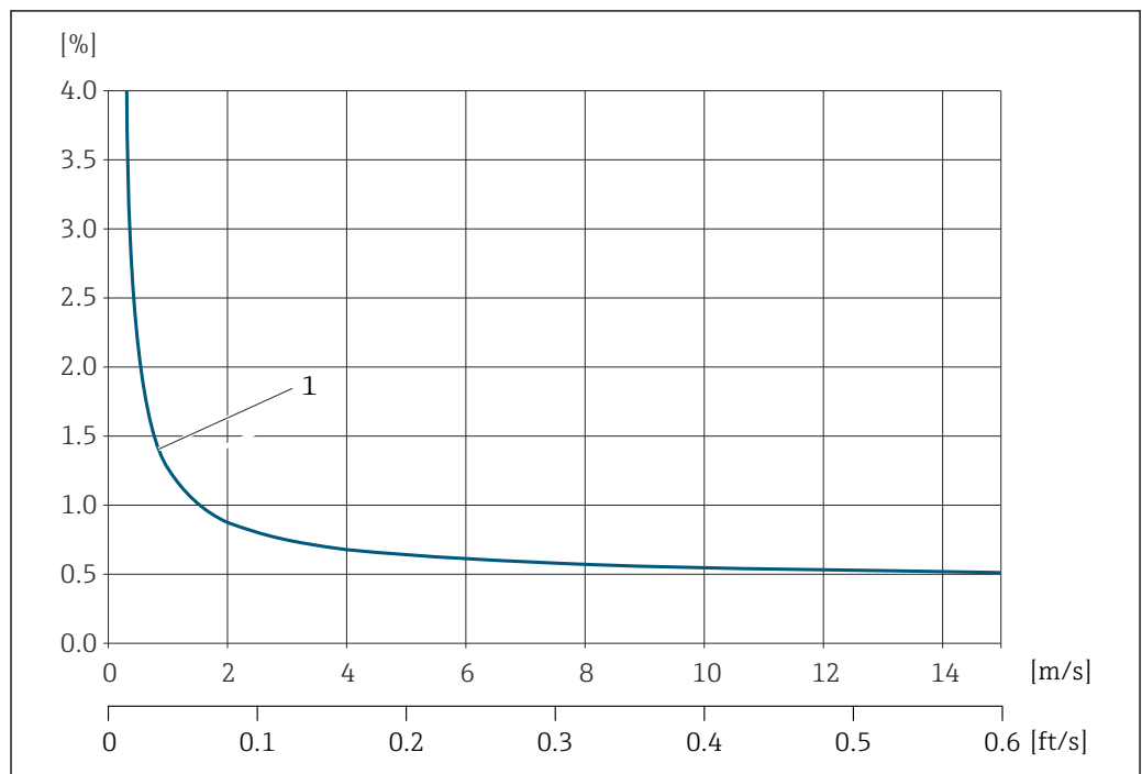
図 26 最大測定誤差の例 (体積流量) (% o.r.)
