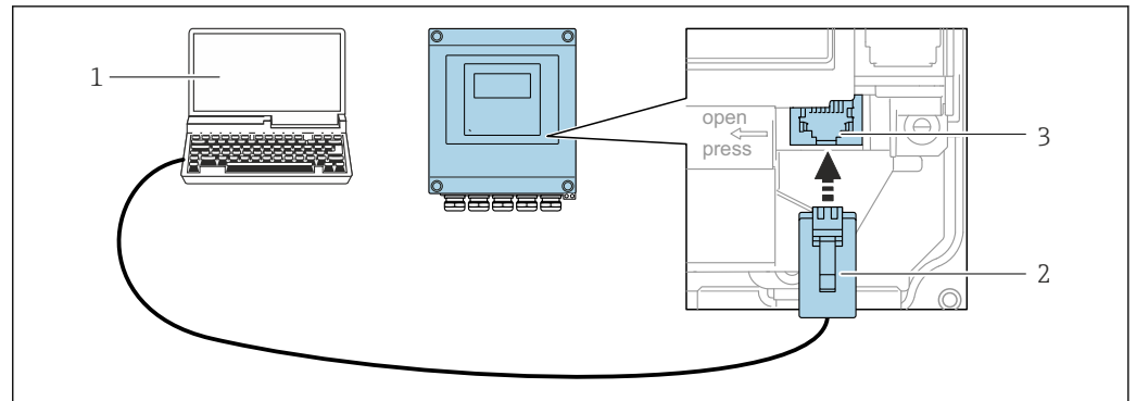
図 18 サービスインタフェース (CDI-RJ45) 経由の接続
