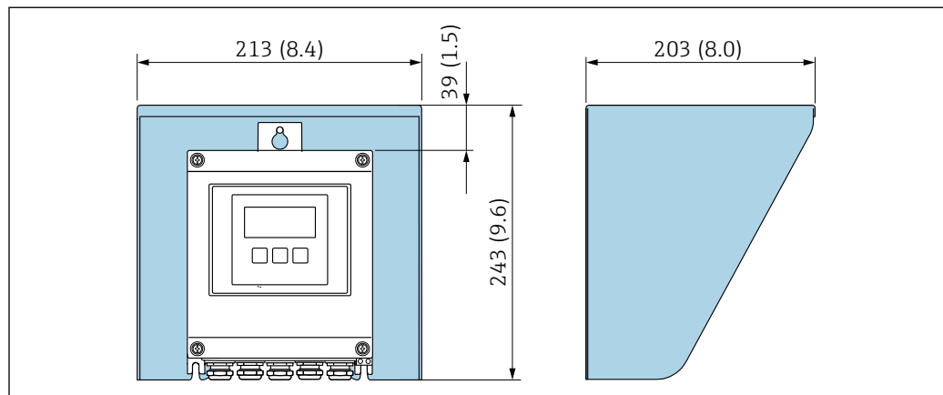
図 8 日除けカバー、寸法：mm (in)
