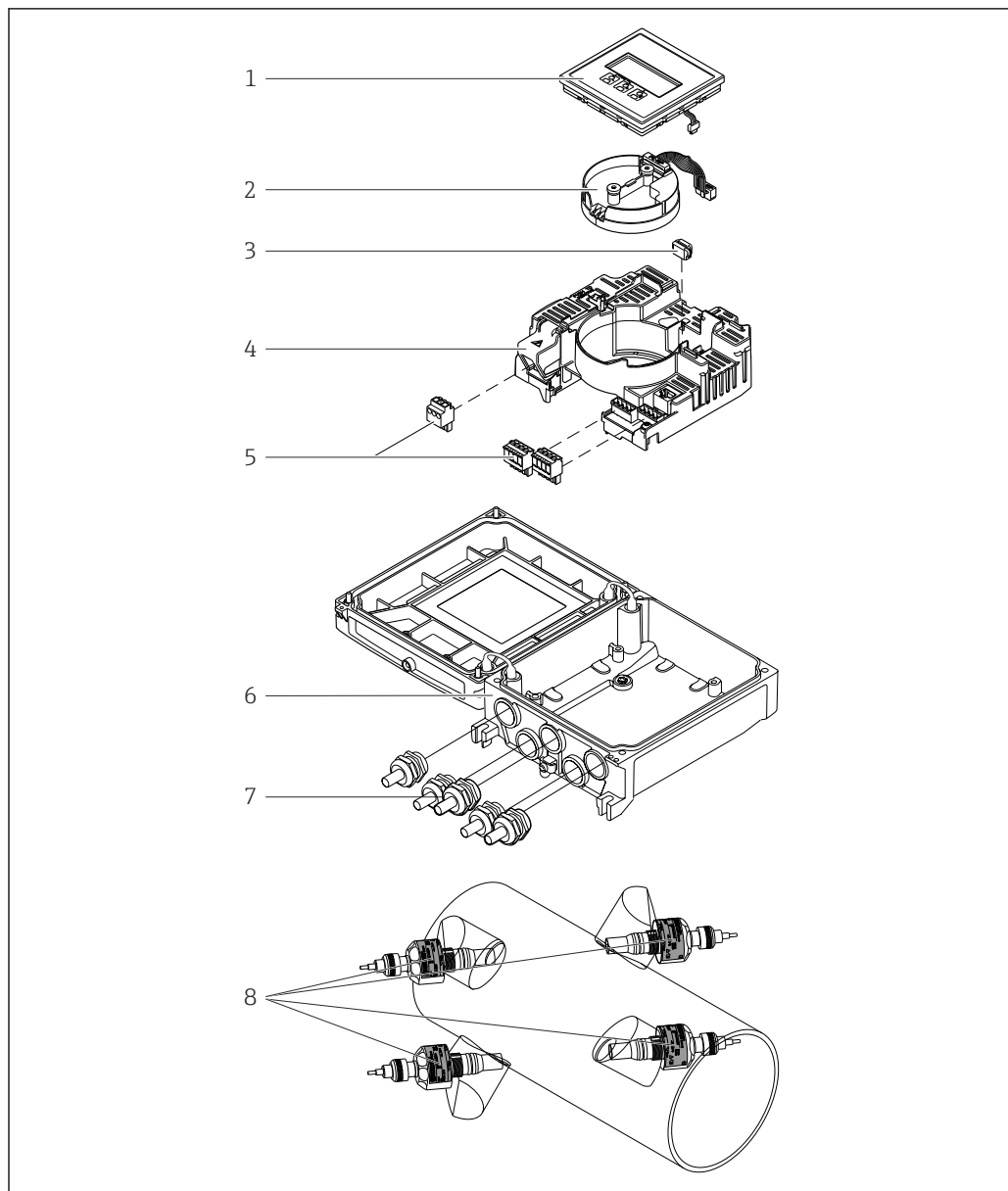
図 1 主要コンポーネント
