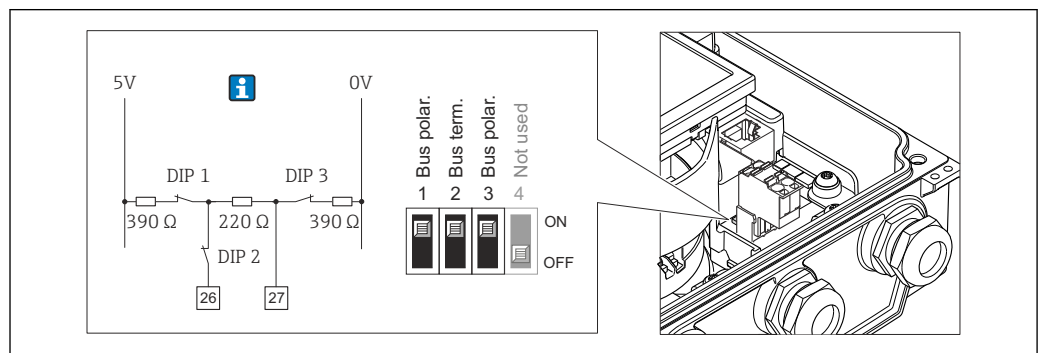
図 14 終端抵抗は電子モジュールの DIP スイッチを使用して有効にできます。
