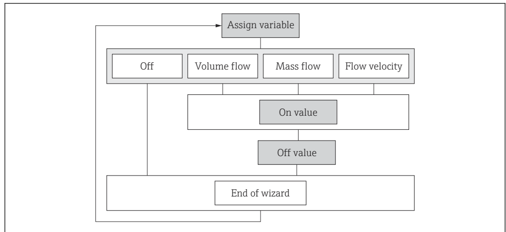
図 21 「設定」メニューの「ローフローカットオフ」ウィザード
