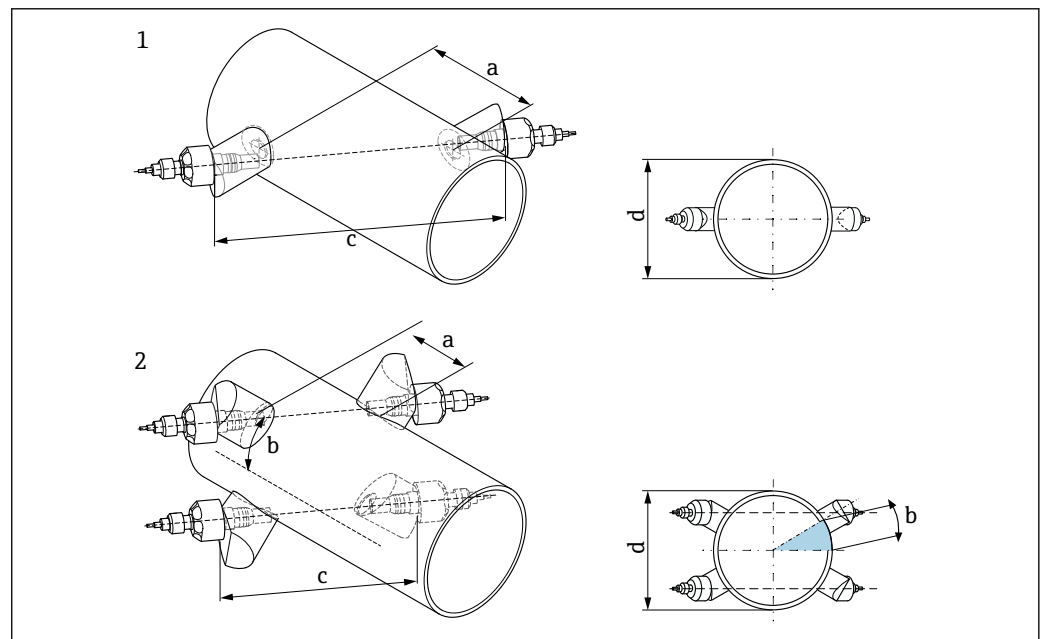
☒ 9 取付に関する用語の説明
