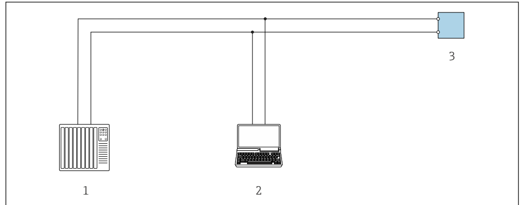
図 17 Modbus RS485 プロトコル経由のリモート操作オプション (アクティブ)
