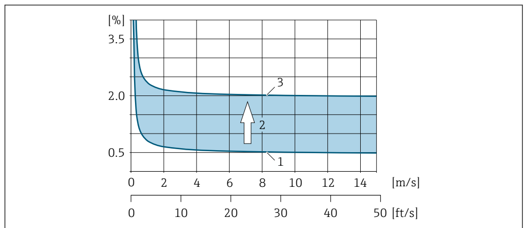
図 25 呼び口径 200A (8") 以上の配管における測定誤差の例
