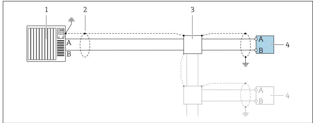
図 13 Modbus RS485（非危険場所およびゾーン 2/Div. 2 用）の接続例
