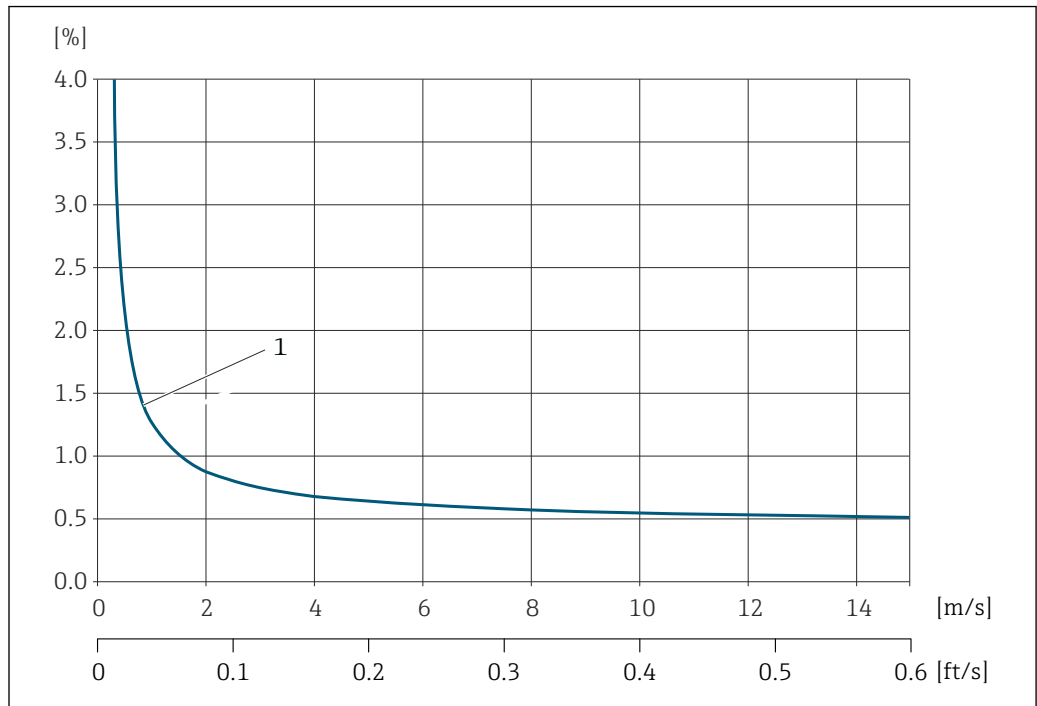
Fig. 26 Ejemplo de error de medición máx. (flujo volumétrico) en % del v. l.
