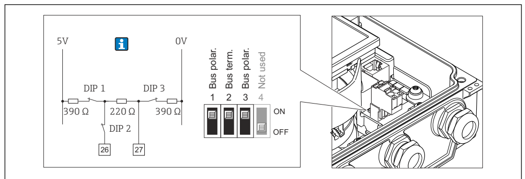
14 La resistencia de terminación se puede habilitar mediante el microinterruptor situado en el módulo del sistema electrónico
