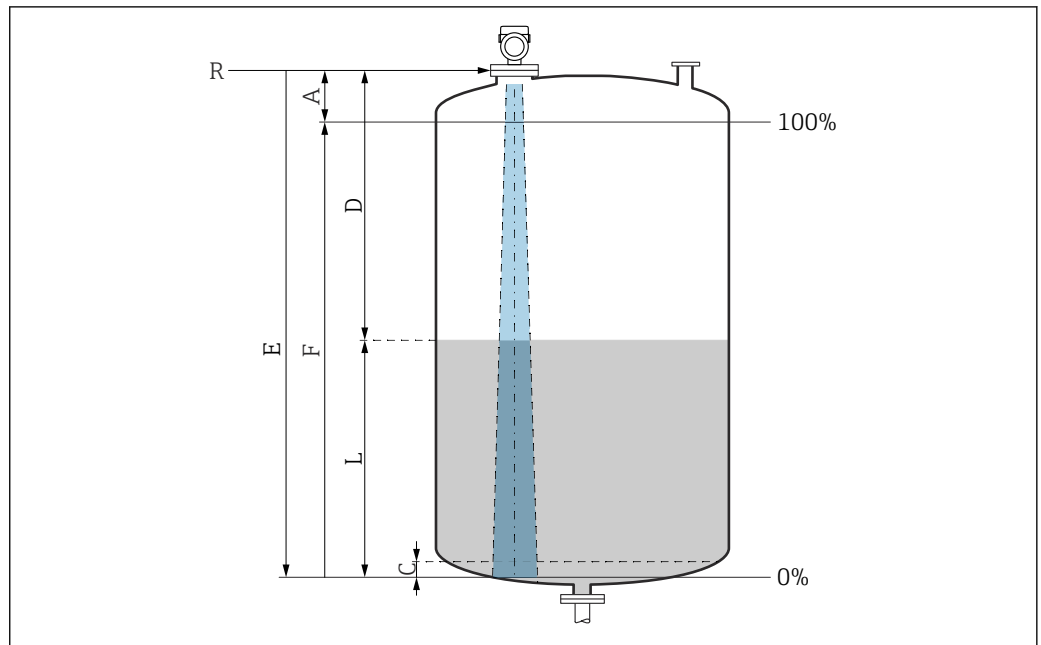
14 Parametri di configurazione per la misura di livello nei liquidi
