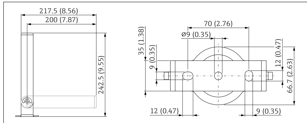
Fig. 29 Dimensioni della staffa di montaggio. Unità di misura mm (in)
