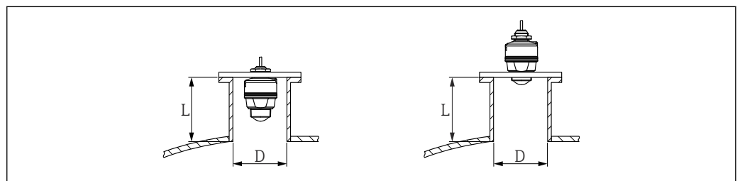
3 Installazione su tronchetto, antenna da 40 mm (1,5 in)
