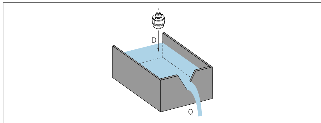
16 Parametri di configurazione per la misura di portata dei liquidi
