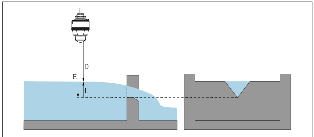
18 Esempio: stramazzo triangolare
