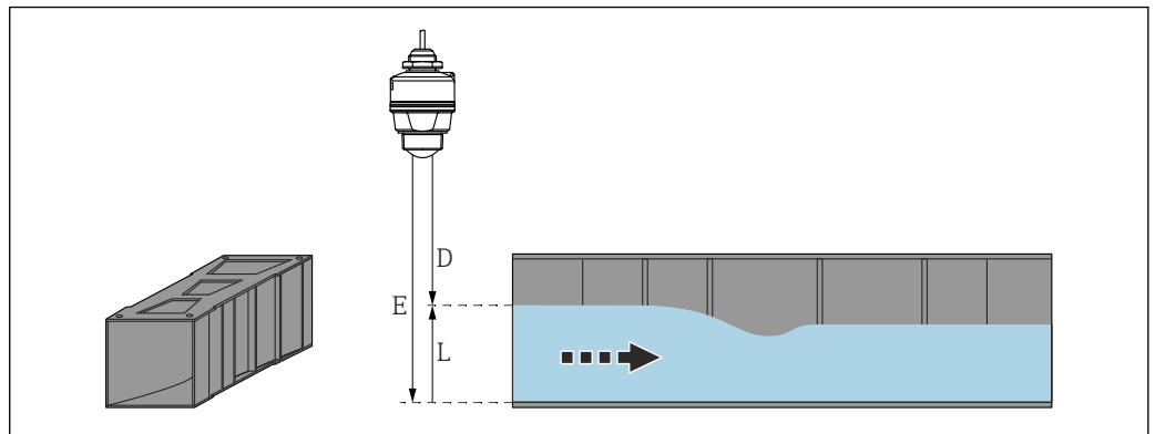
17 Esempio: canali aperti Khafagi-Venturi
