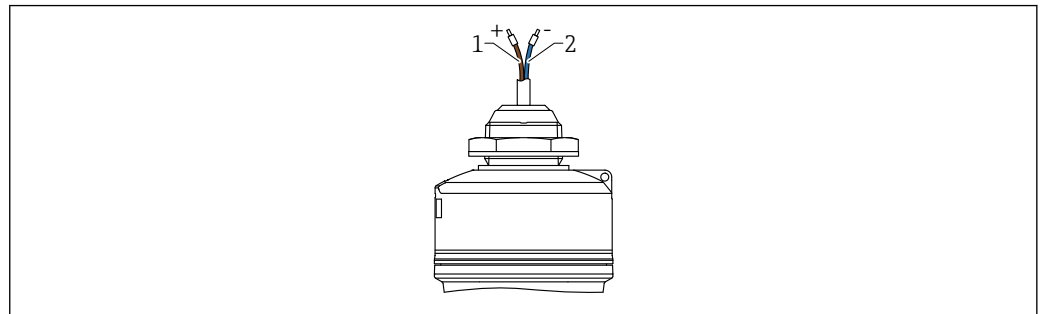
10 Assegnazione dei cavi, ingresso cavo dall'alto
