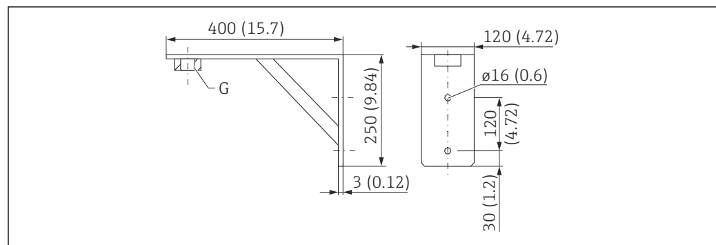
Fig. 30 Dimensioni della staffa di montaggio. Unità di misura mm (in)
