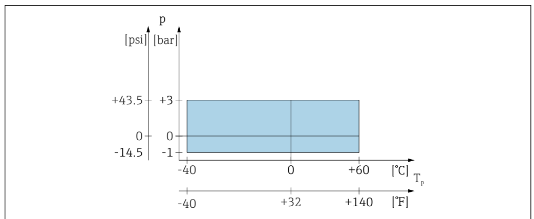
46 Campo consentito per temperatura e pressione di processo
