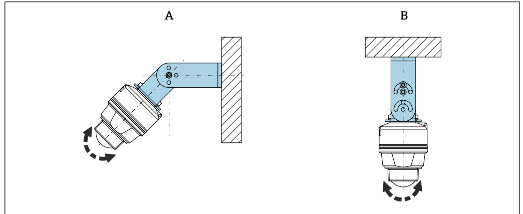
6 Installazione con staffa di montaggio, regolabile
