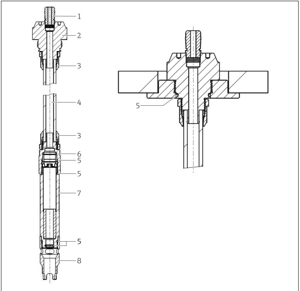
1 Aufbau CYA10
