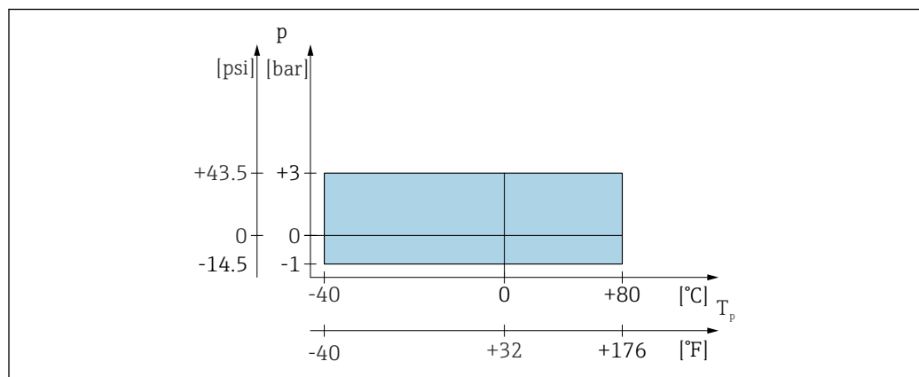
20 Faixa permitida para temperatura do processo e pressão do processo
