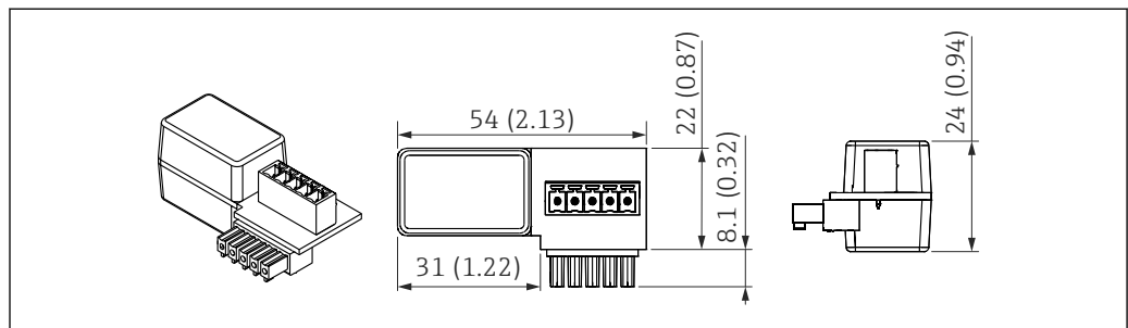
61 Dimensões do resistor de comunicação HART. Unidade de medida mm (in)
