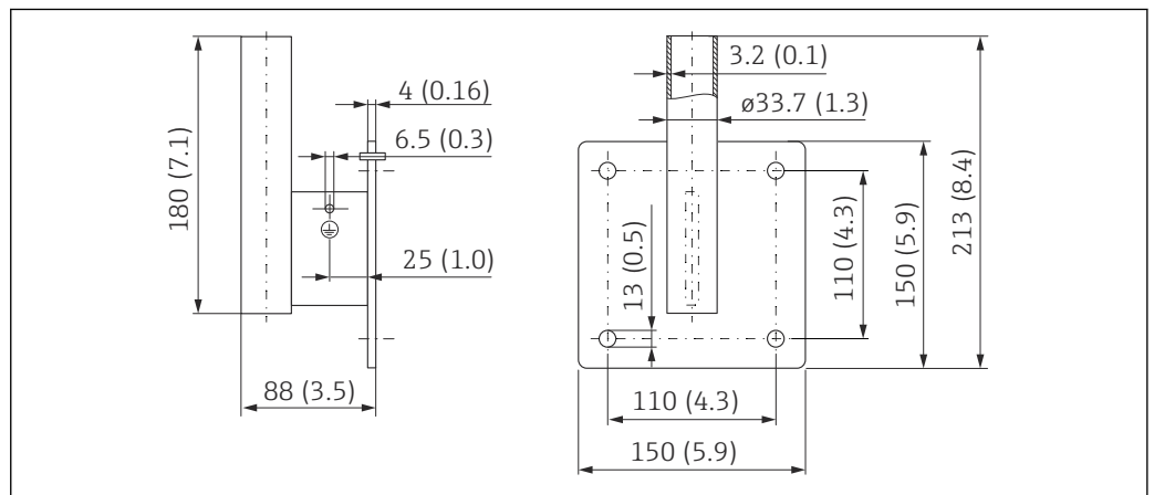
37 壁面ブラケットの寸法。測定単位 mm (in)
