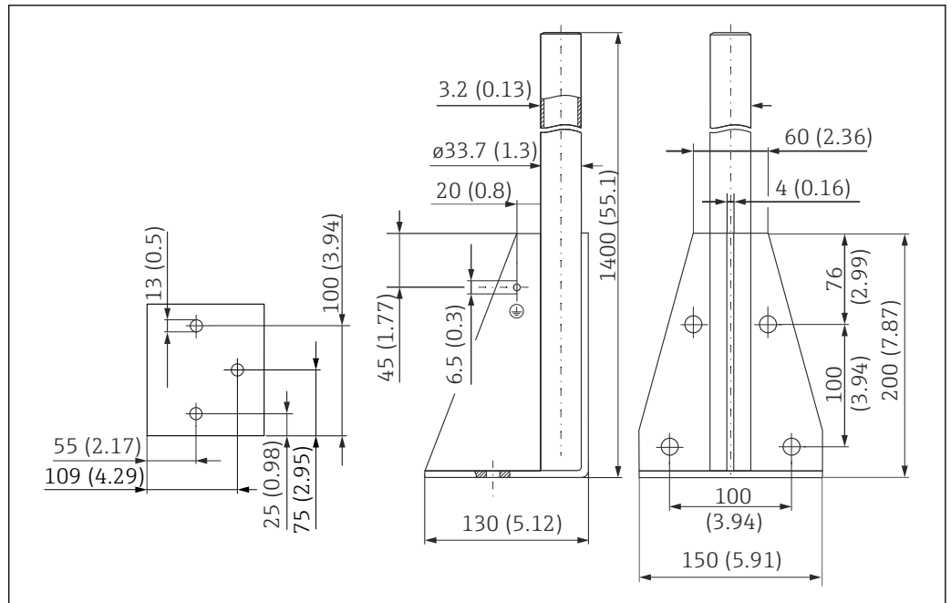
36 寸法。測定単位 mm (in)
