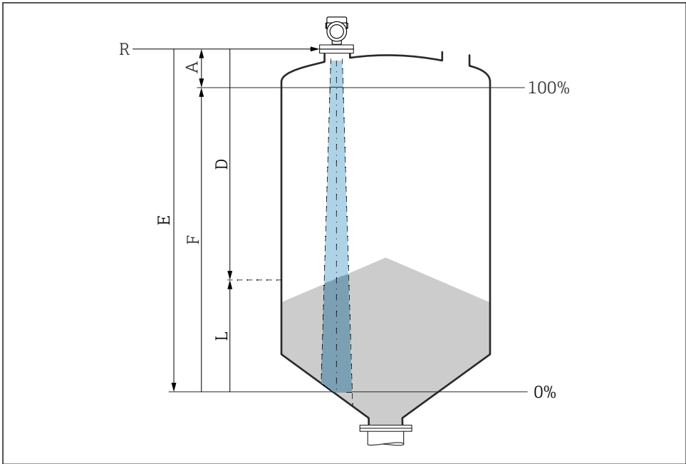
14 Konfigurationsparameter zur Füllstandmessung in Schüttgütern
