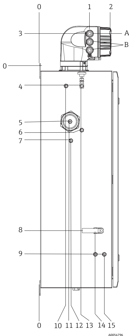
Figure 5. Dimensions de montage : Vue de côté
