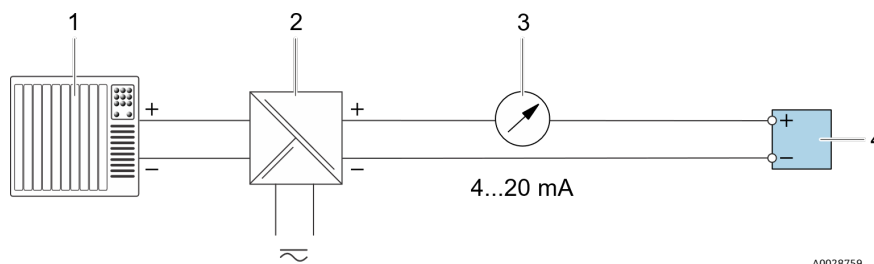
Figure 28. Exemple de raccordement pour sortie courant 4-20 mA, passive
