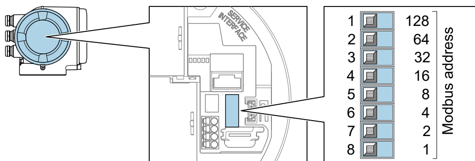
Figure 34. Commutateurs DIP pour l'adresse Modbus
