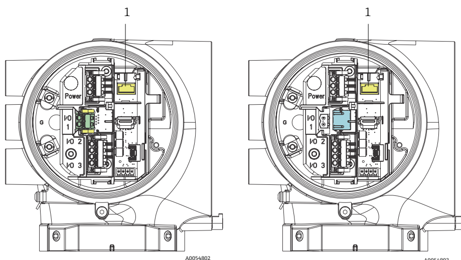
Figure 30. Connexions de l'interface service CDI-RJ45 (1) pour I/O1 avec Modbus RTU/RS485/2 fils (à gauche) et Modbus TCP/Ethernet/RJ45 (à droite)
