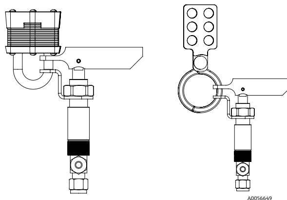
Figure 1. Verrouillage et étiquetage du TDLAS JT33
