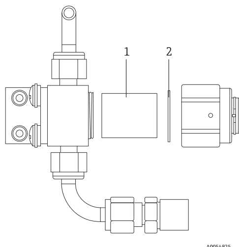
Figure 74. Retrait du filtre et du joint
