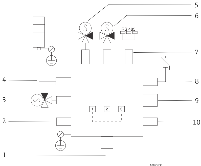
Figure 12. Emplacements des instruments/capteurs conçus pour le boîtier MAC
