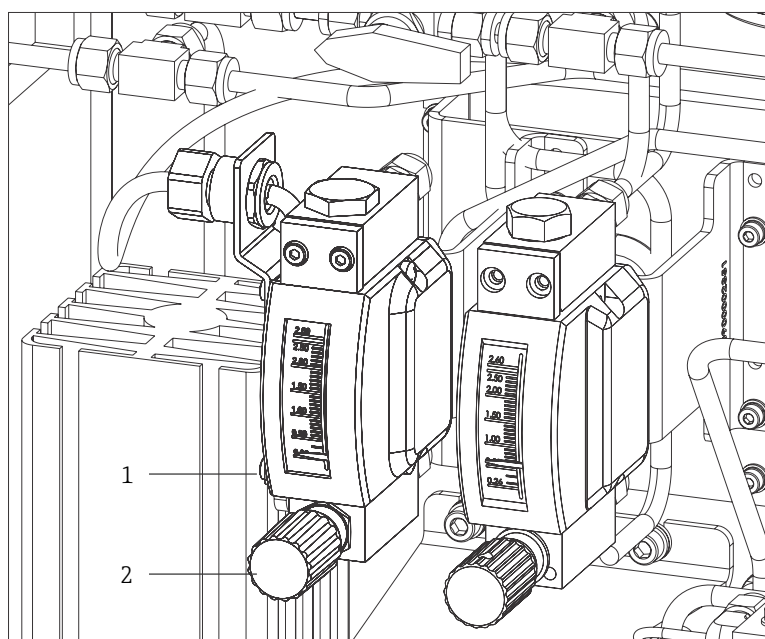
Figure 33. Réglages du détecteur de débit
