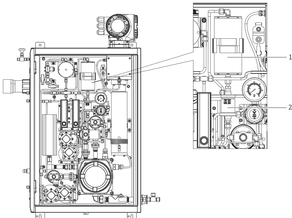
Figure 72. Épurateur et indicateur d'efficacité de l'épurateur
