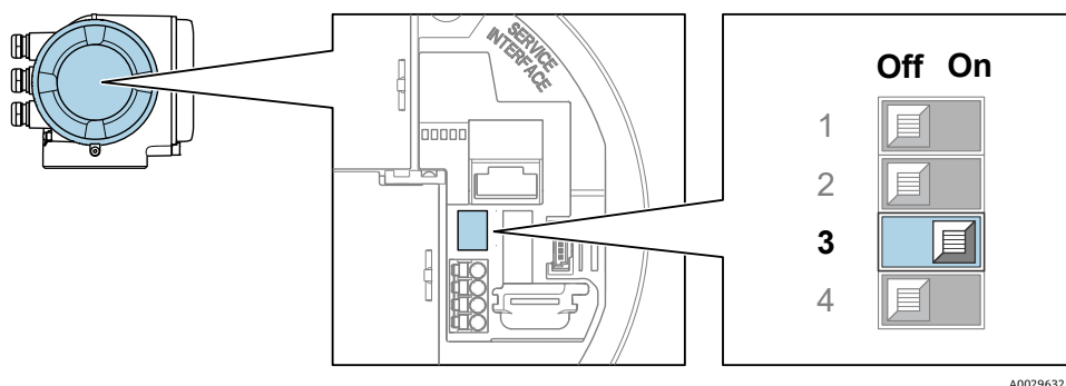
Figure 35. Sélection Off/On des commutateurs DIP pour l'activation de la résistance de fin de ligne
