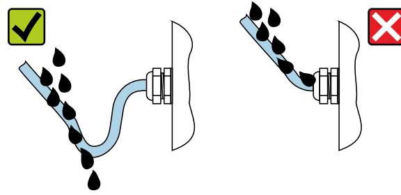
Figure 38. Garantir l'indice de protection IP66
