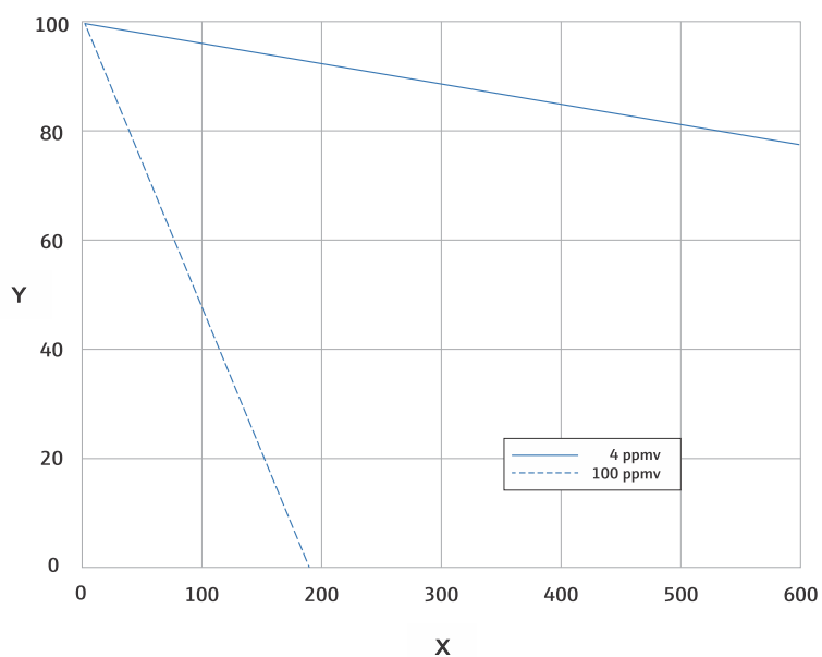
Figure 71. Durée de vie prévue de l'épurateur en fonction de la charge moyenne en H 2 S
