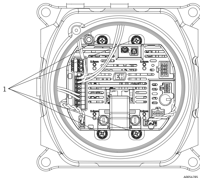
Figure 76. Emplacements des vis de panneau imperdables (1)
