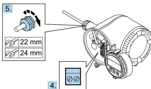
Figure 17. Raccordement des câbles et serrage des presse-étoupe
