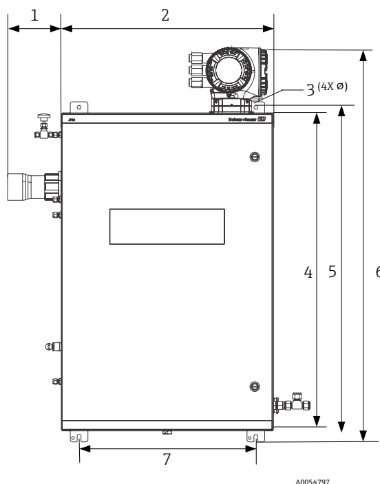
Figure 6. Dimensions de montage : Vue de face
