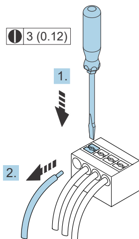
Figure 29. Déconnexion d'un câble. Unité de mesure : mm (in)
