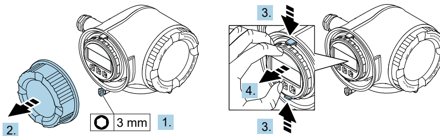
Figure 18. Retirer le support du module d'affichage
