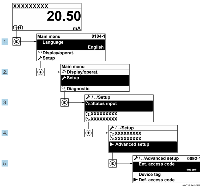
Figure 57. Navigation vers le menu Advanced setup
