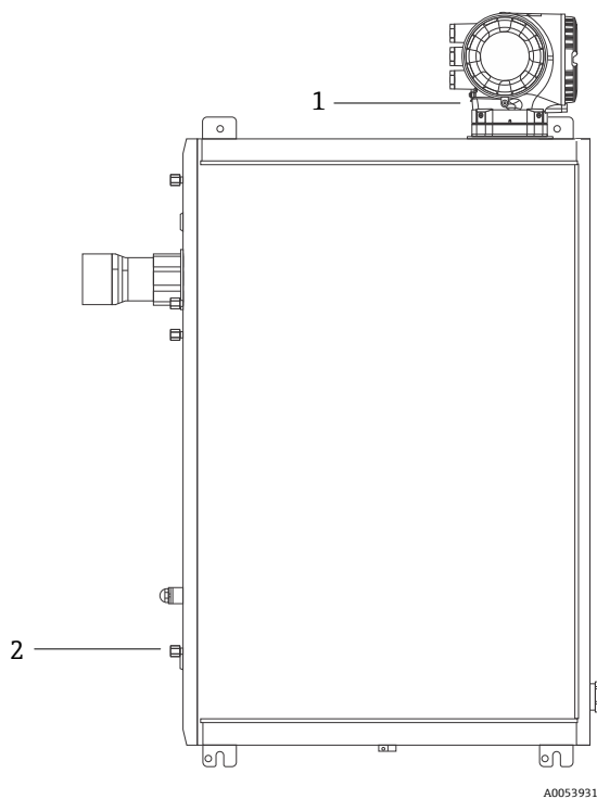
Figure 10. Prises de terre
