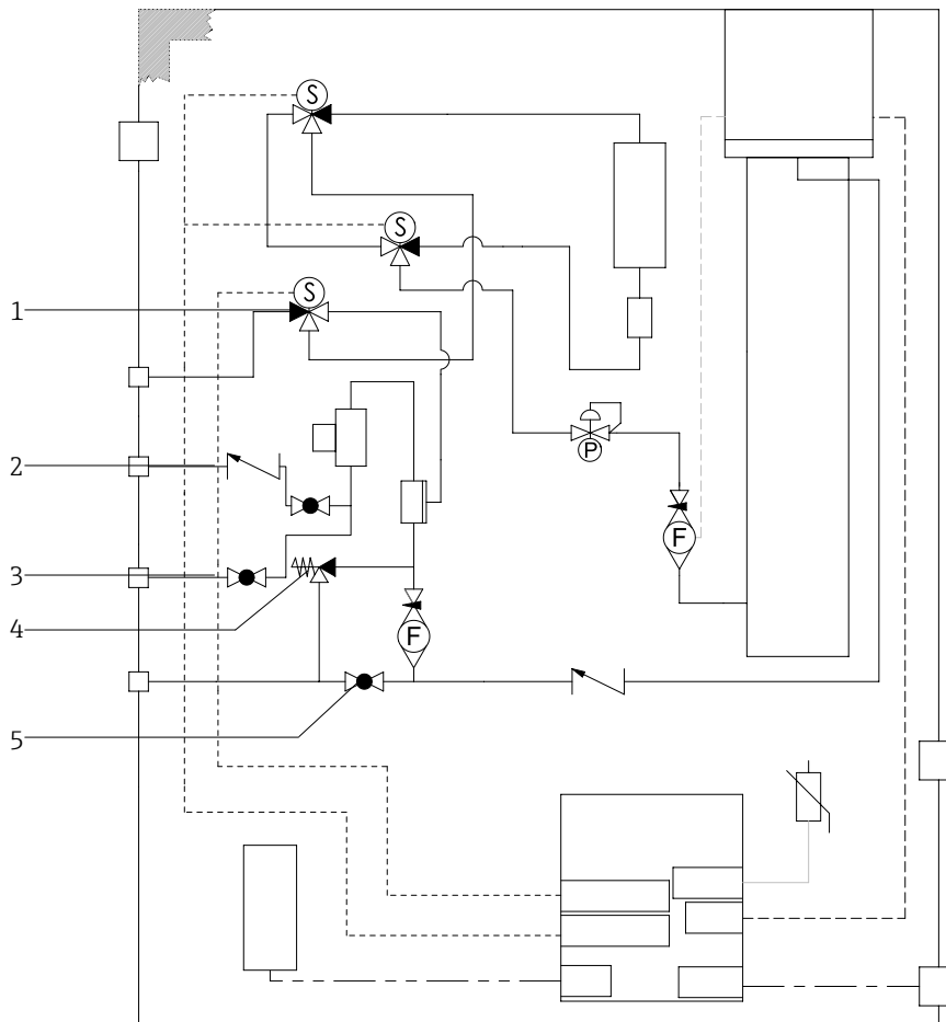
Figure 32. Emplacements des vannes
