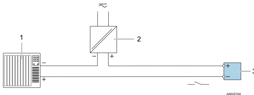
Figure 24. Exemple de raccordement pour sortie relais, passive
