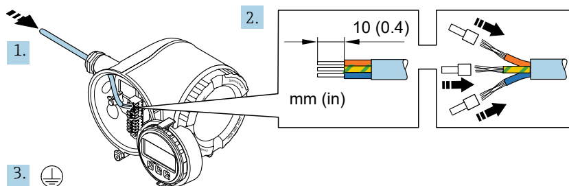
Figure 21. Câblage de l'alimentation et raccordement de la terre de protection
