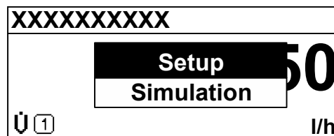
Figure 45. Menu contextuel
