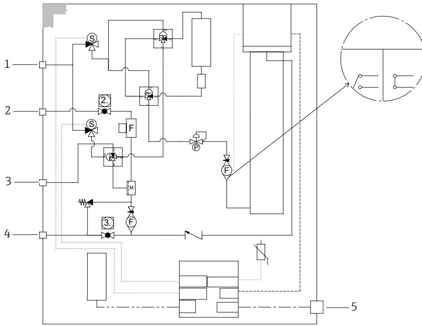
Figure 85. Différentiel pneumatique avec validation en un point
