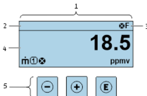
Figure 42. Affichage de fonctionnement
