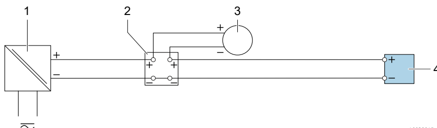
Figure 25. Exemple de raccordement pour entrée courant 4 à 20 mA
