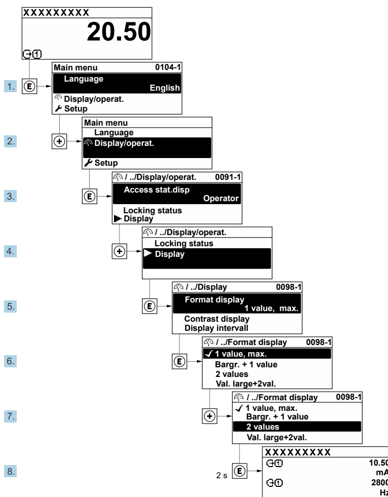
Figure 46. Réglage du nombre de valeurs mesurées affichées sur 2 valeurs
