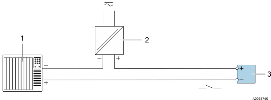
Figure 23. Exemple de raccordement pour la sortie tor, passive
