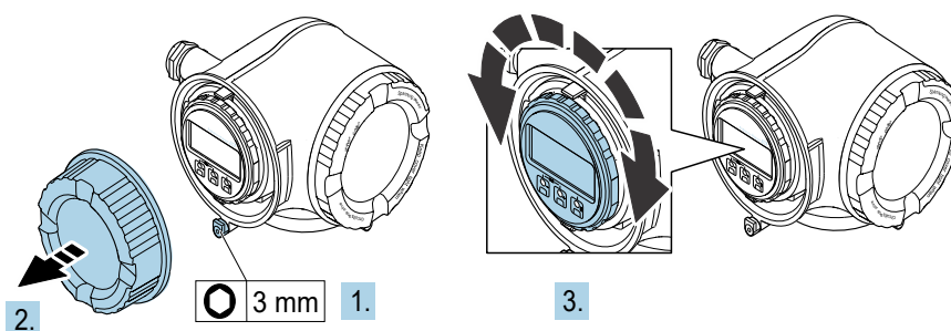
Figure 9. Rotation du module d'affichage
