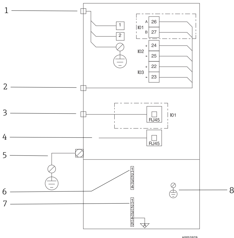
Figure 11. Raccords électriques de l'analyseur JT33
