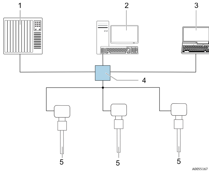
Figure 54. Connexion via le protocole Modbus TCP
