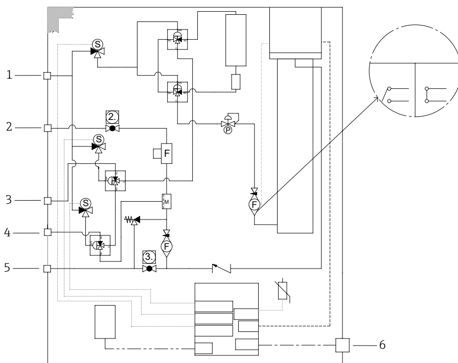
Figure 86. Différentiel pneumatique avec validation en deux points
