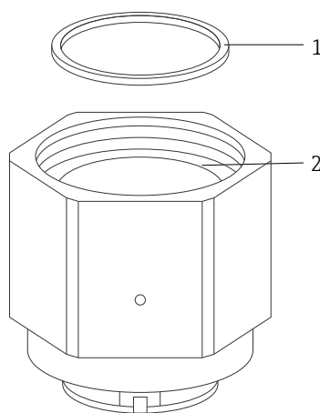
Figure 75. Centrage du joint sur la surface d'étanchéité du capuchon
