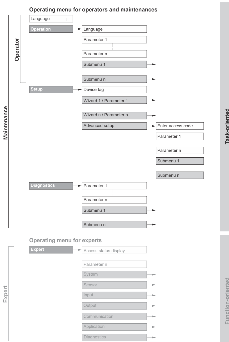
Figure 40. Structure schématique du menu de configuration
