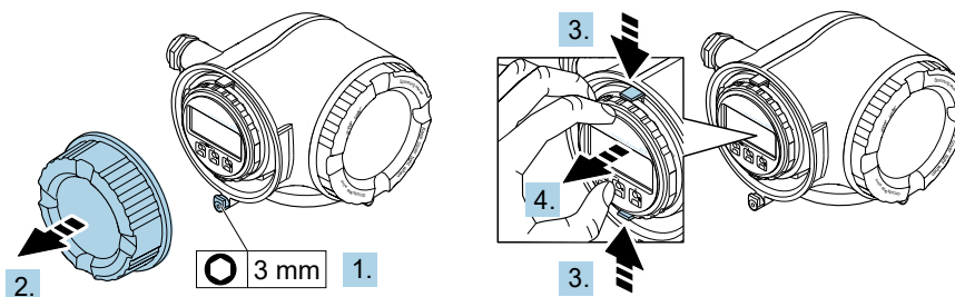
Figure 14. Retirer le support du module d'affichage
