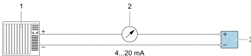
Figure 27. Exemple de raccordement pour sortie courant 4-20 mA, active
