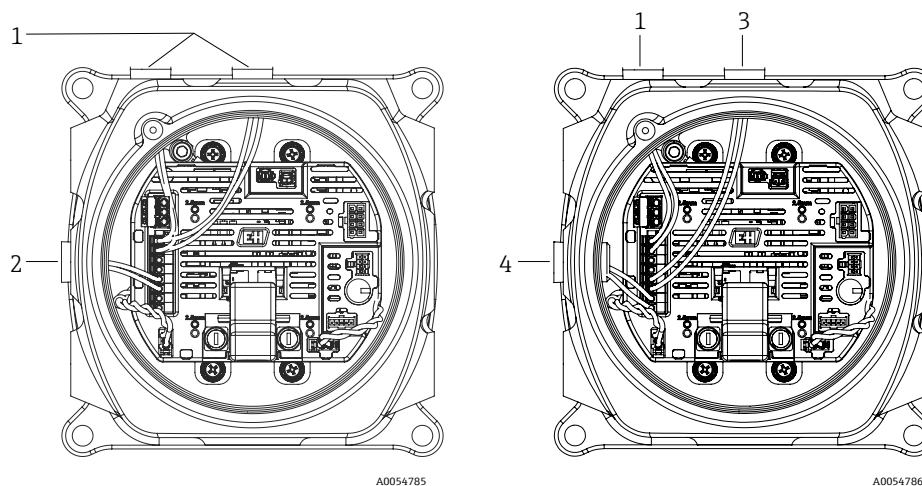
Figure 81. Câblage des électrovannes : configuration électrique (à gauche) et pneumatique (à droite)
