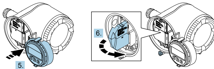
Figure 19. Ouverture du cache-bornes
