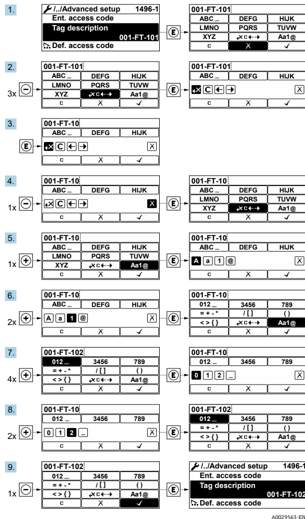
Figure 48. Modification de la désignation du point de mesure dans le paramètre "Tag description"
