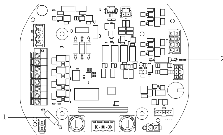
Figure 78. Emplacements des fusibles de coupure thermique
