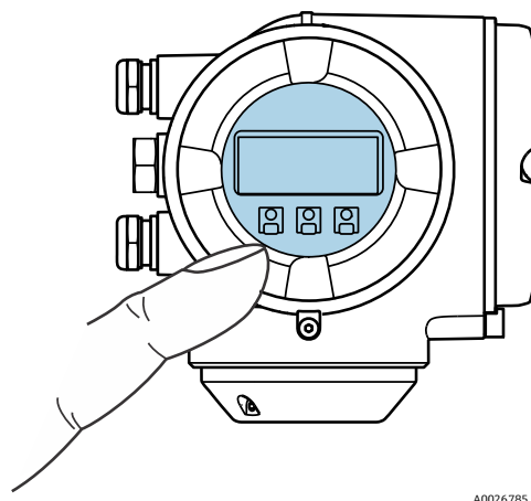
Figure 41. Configuration par éléments de commande tactiles
