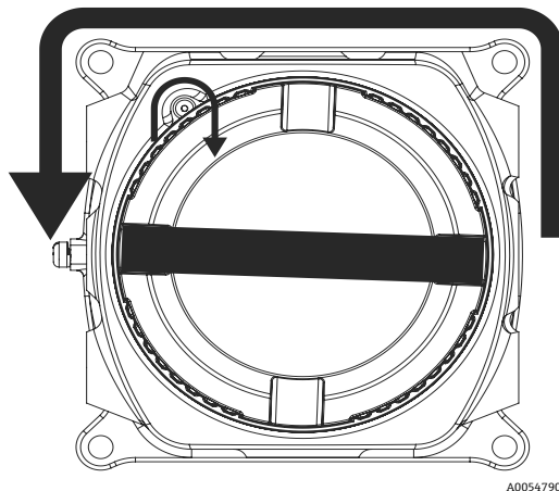
Figure 80. Retrait du couvercle MAC
