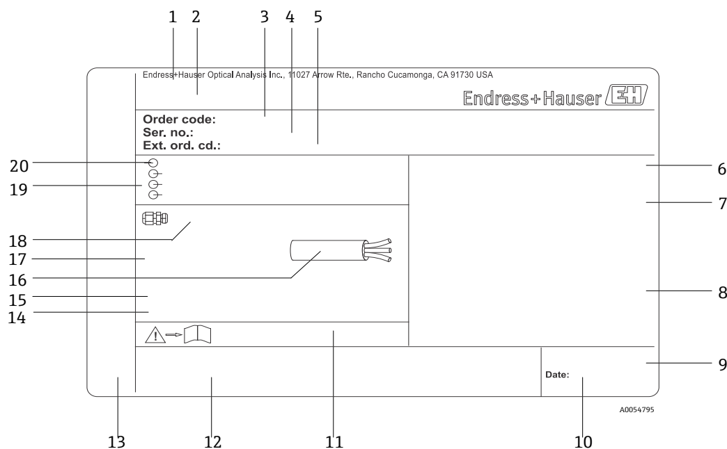
Figure 3. Modèle de plaque signalétique de l'analyseur de gaz TDLAS JT33
