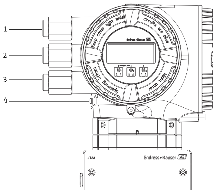
Figure 13. Entrées filetées
