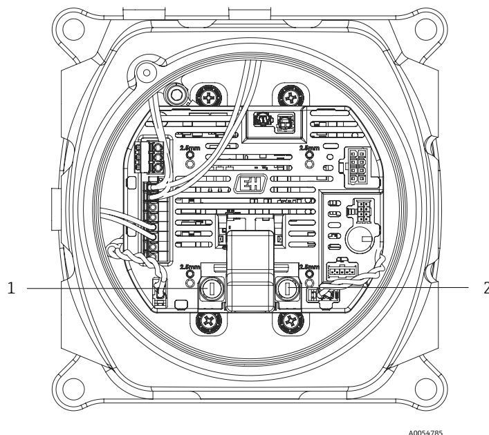
Figure 77. Emplacements des fusibles du circuit MAC
