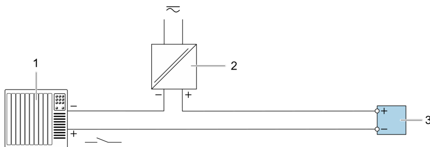
Figure 26. Exemple de raccordement pour l'entrée état
