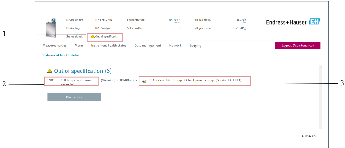
Figure 68. Informations de diagnostic dans le navigateur web
