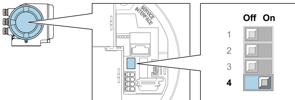
Figure 37. Commutateur DIP pour l'adresse IP par défaut
