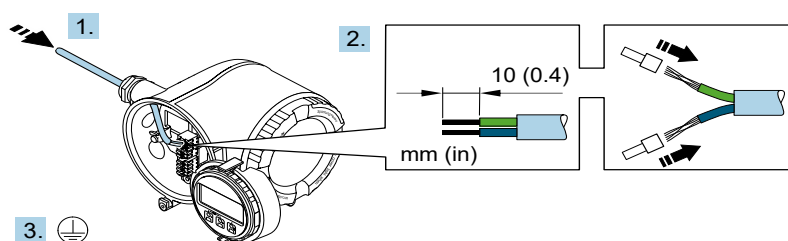
Figure 16. Câblage de l'alimentation et raccordement de la terre de protection
