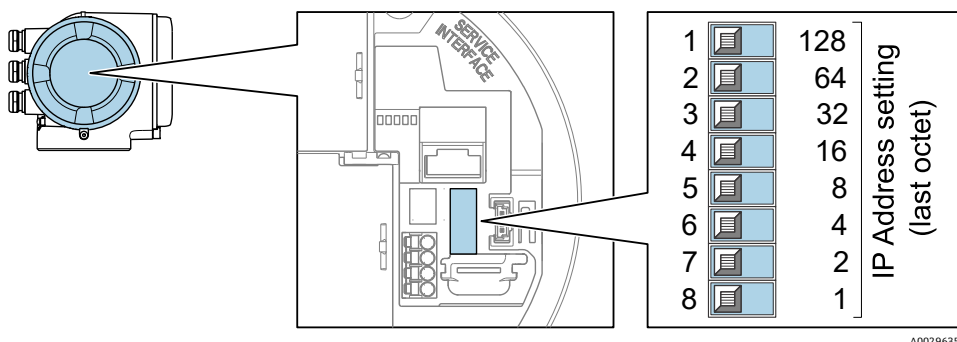
Figure 36. Commutateurs DIP pour le réglage de l'adresse IP
