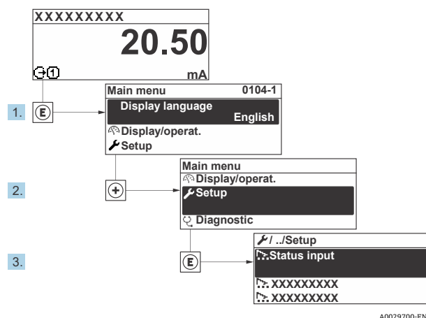
Figure 55. Exemple de l'afficheur local
