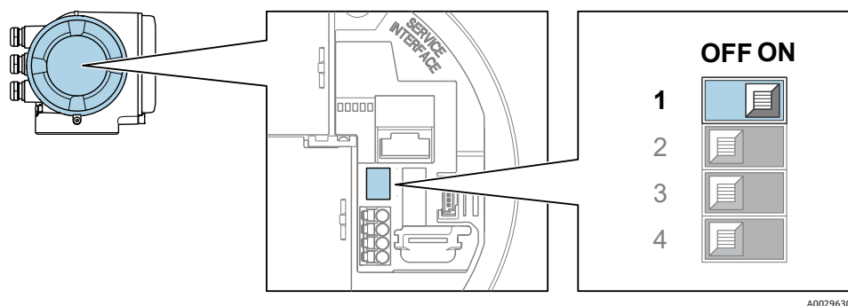
Figure 59. Commutateur DIP pour la protection en écriture
