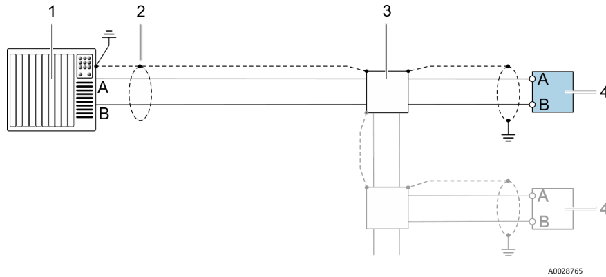
Figure 22. Exemple de raccordement pour Modbus RS485, zone non explosible et Zone 2/Div.2
