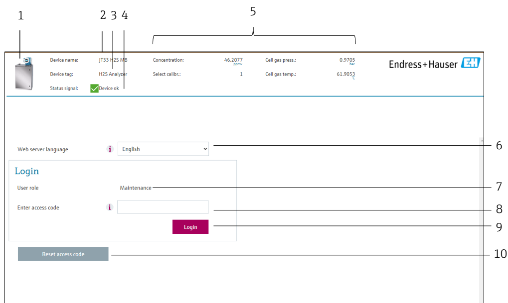
Figure 51. Page de connexion
