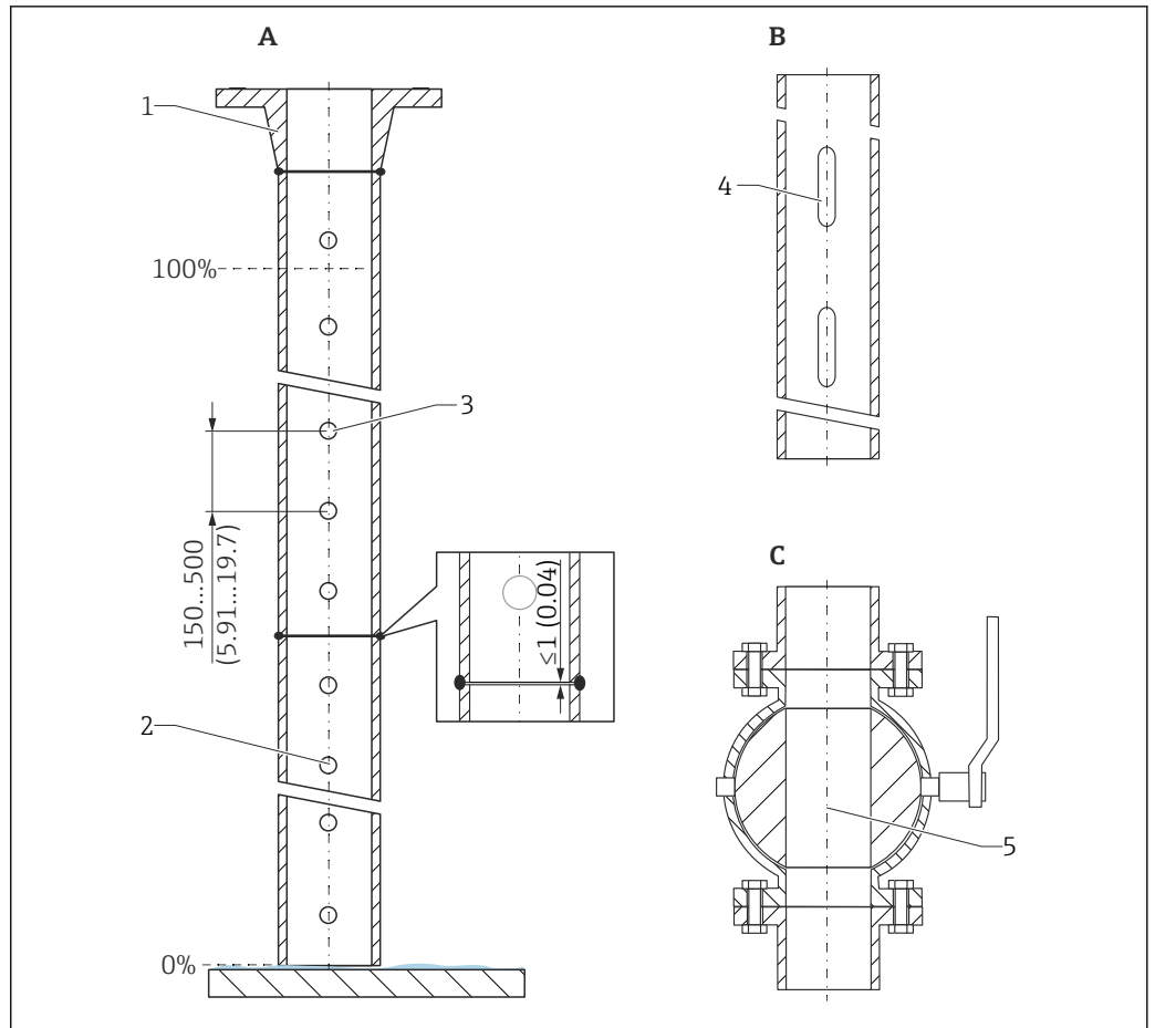
12 Konstruktionsbeispiel Schwallrohr. Maßeinheit mm (in)
