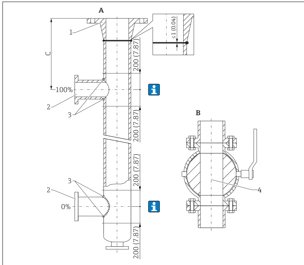
14 Konstruktionsbeispiel Bypass. Maßeinheit mm (in)
