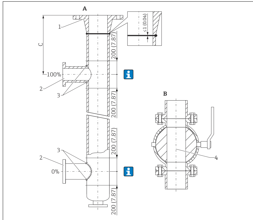
13 Konstruktionsbeispiel Bypass. Maßeinheit mm (in)
