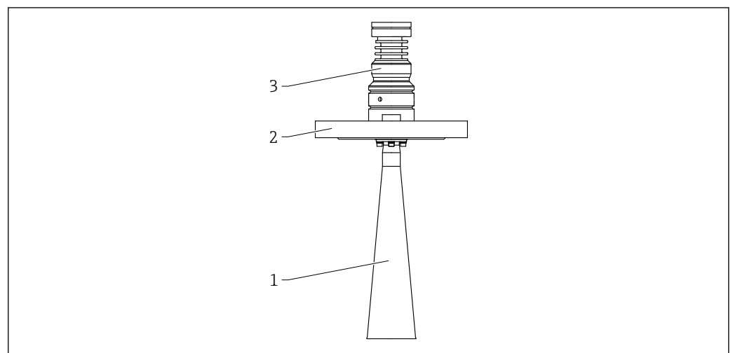
62 Material; DN65 Hornantenne. Maßeinheit mm (in)
