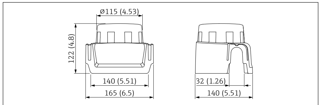
69 Abmessungen Wetterschutzhaube, Kunststoff, XW111. Maßeinheit mm (in)
