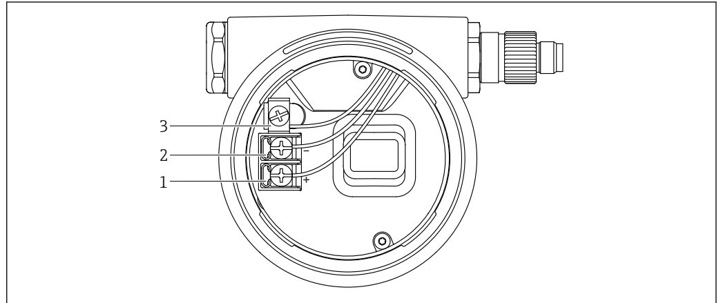
图 2 接线腔中的接线端子和接地端
