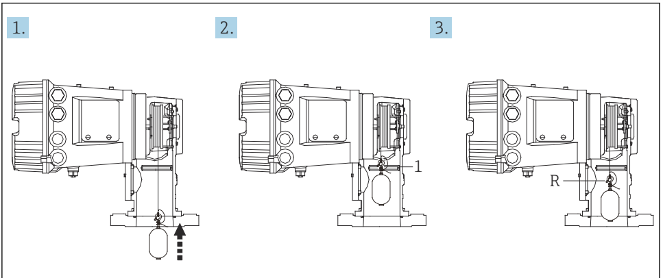
28 Vertailukalibroinnin vaiheet
