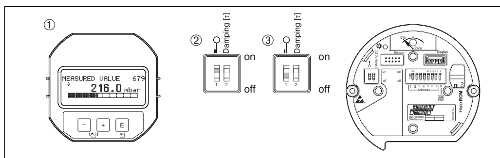
Fig. 14: Posição da minisseletores "Hardware locking" na unidade eletrônica
