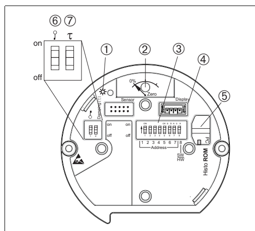
Fig. 8: Tecla de operação e elementos de operação, interno
