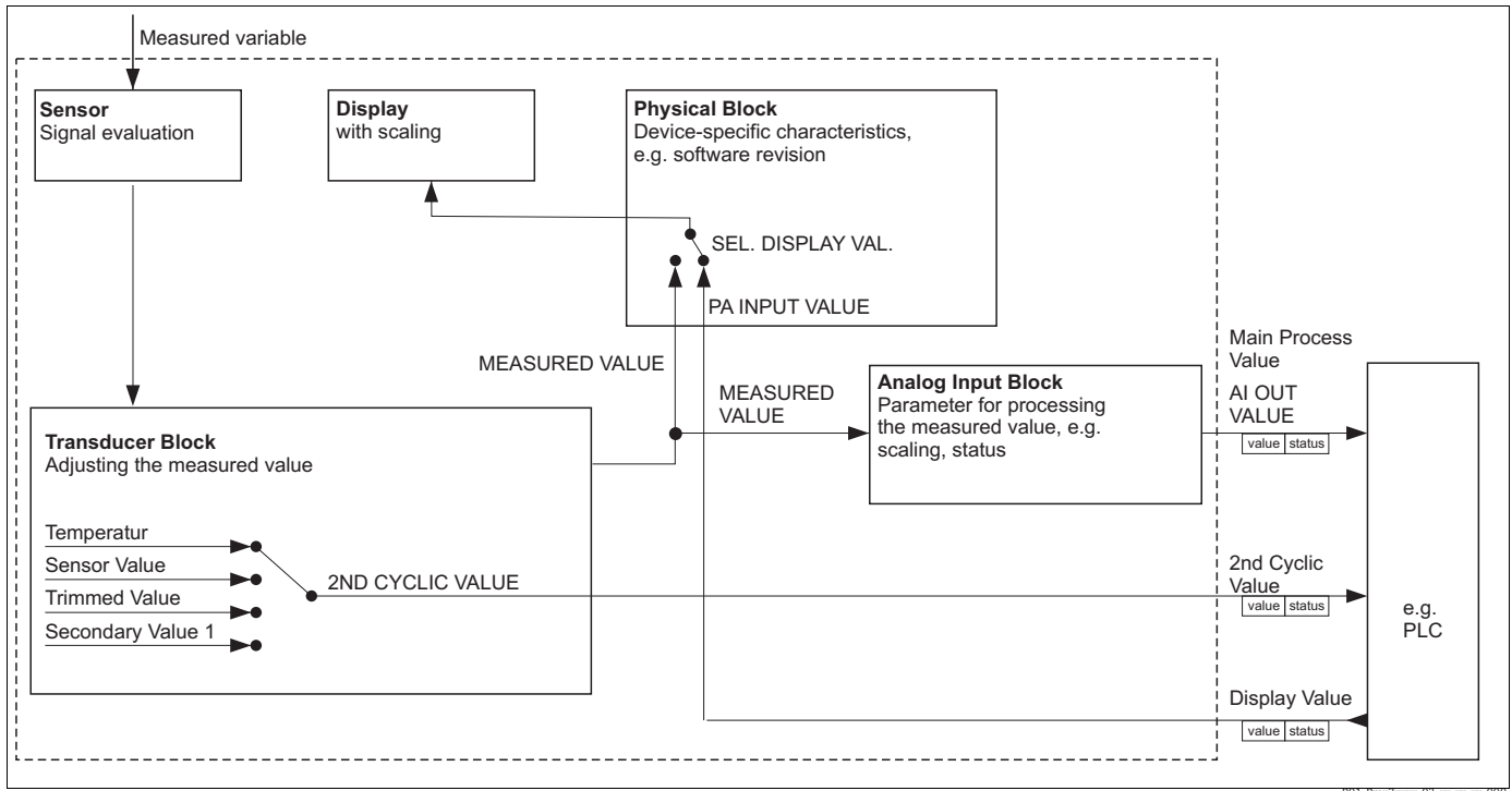
Fig. 12: O modelo de blocos mostra quais dados podem ser transmitidos entre o Deltapilot S e o mestre Classe 1 (por ex., CLP) durante a troca cíclica de dados. Usando o software de configuração do seu CLP, compile o telegrama de dados cíclicos com a ajuda dos módulos (→ consulte também este capítulo, seção "Módulos para o diagrama de dados cíclicos"). Os parâmetros, escritos em MAIÚSCULAS, são parâmetros no programa de operação (por ex., FieldCare) que podem ser usados para fazer configurações para o telegrama de dados cíclicos ou para exibir valores (→ consulte também este capítulo, seção Descrição do parâmetro).
