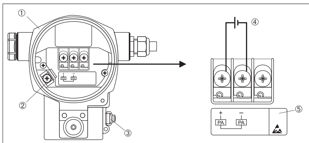
Fig. 5: Conexão elétrica do PROFIBUS PA → Consulte também → 18, cap. 5.2.1 "Tensão de alimentação".
