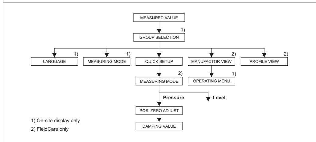
Fig. 16: Menu Quick Setup para modo de medição "Pressure"
