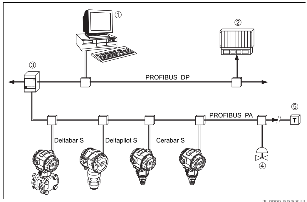
Fig. 9: Arquitetura do sistema PROFIBUS
