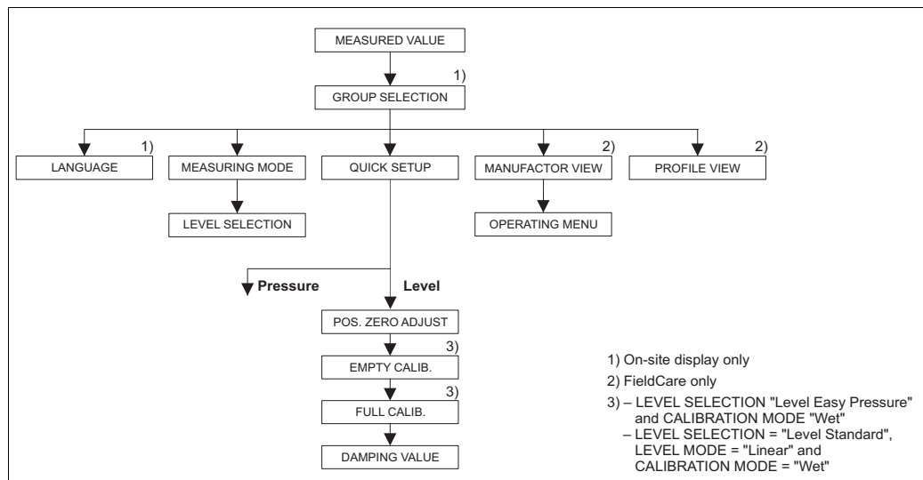
Fig. 15: Menu quick setup para modo de medição "Level"
