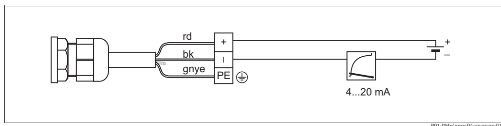
Fig. 6: rd = vermelho, bk = preto, gnye = verde/amarelo
