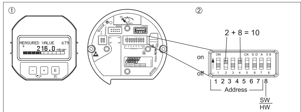
Fig. 10: Configuração do endereço do instrumento utilizando minisseletoras
