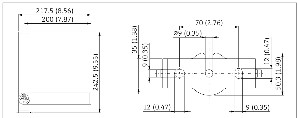
图 28 安装架的外形尺寸示意图。测量单位 mm (in)
