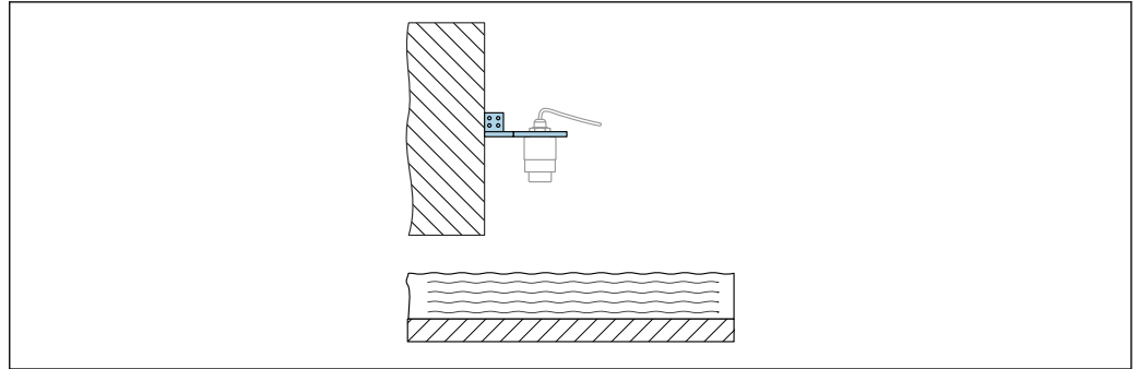
图 14 使用悬臂和墙装架安装，悬臂可以旋转和调节（例如在水渠正上方定位设备）
