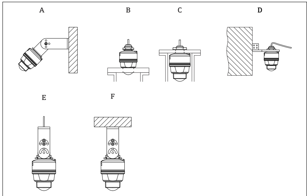
图 6 安装在墙壁或罐顶上
