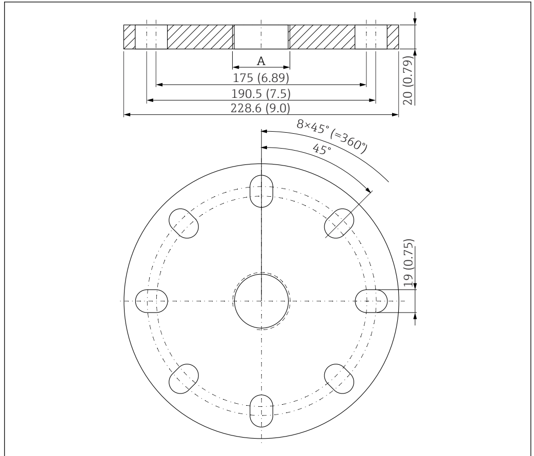
图 44 UNI 4"/DN100/100 法兰的外形尺寸示意图。测量单位 mm (in)
