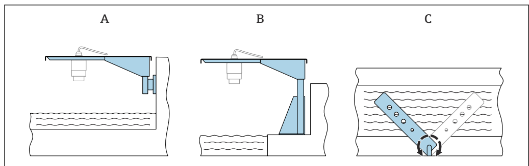
图 13 使用悬臂安装（可旋转）
