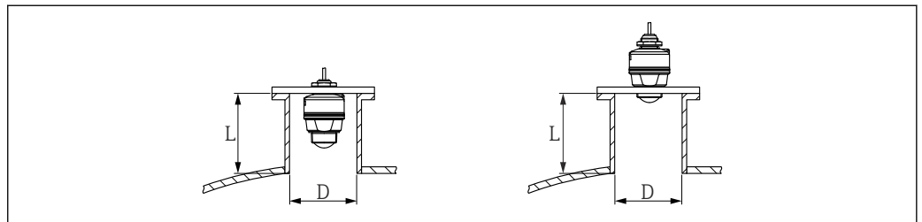
7 安装在安装短管中 (40 mm (1.5 in) 口径天线)
