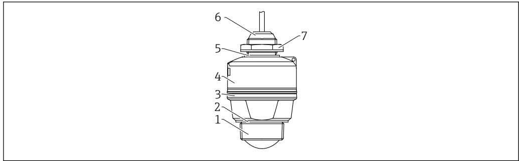
图 18 材质概览：40 mm (1.5 in)口径天线，电缆入口螺纹
