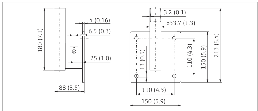
图 39 墙装架的外形尺寸。测量单位 mm (in)
