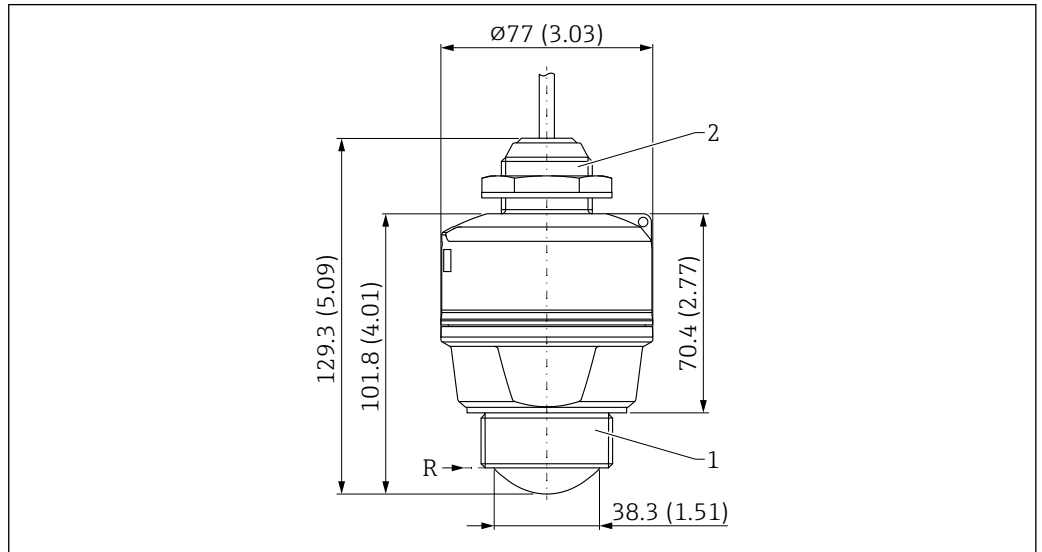
图 16 外形尺寸示意图；40 mm (1.5 in)口径天线，顶部电缆入口。测量单位 mm (in)
