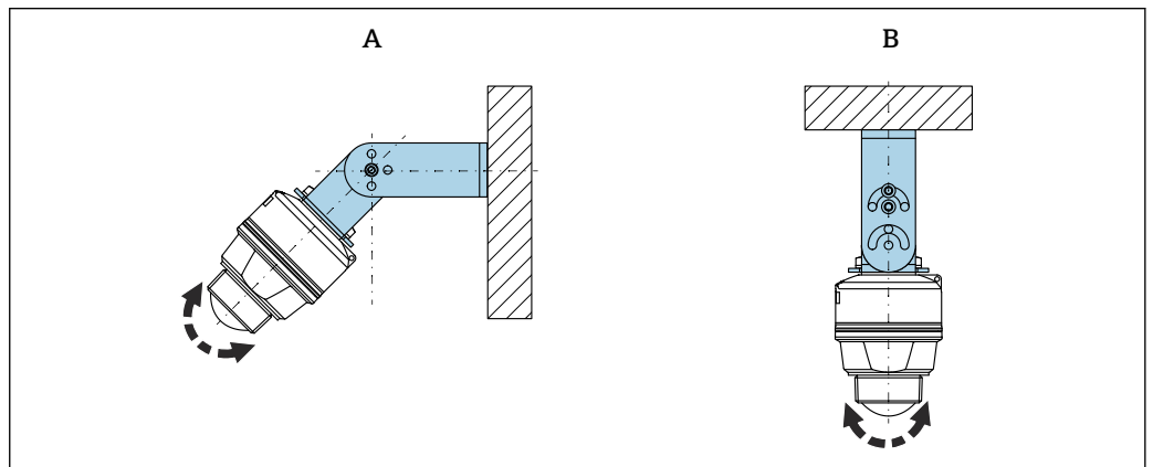
图 11 使用安装架安装（可调节）
