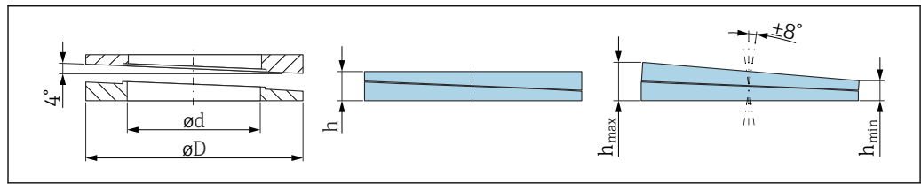
图 45 外形尺寸
