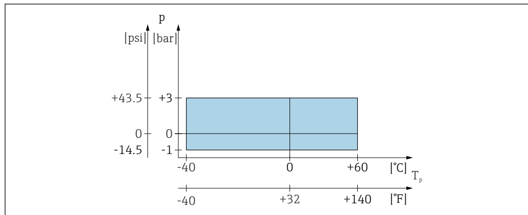
图 15 允许过程温度和过程压力
