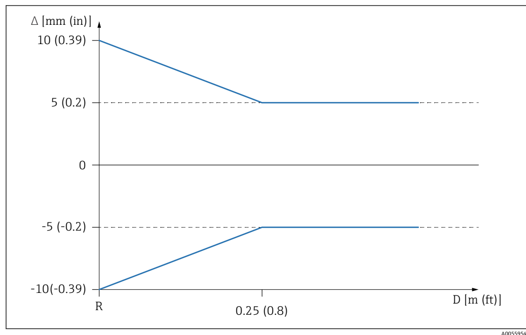
图 4 近距离测量时的最大测量误差
