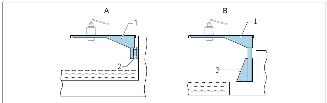
图 34 传感器天线端过程连接的安装方式
