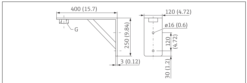
图 30 安装架的外形尺寸示意图。测量单位 mm (in)
