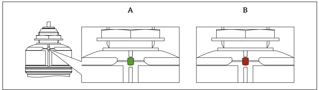
图 19 设备上的 LED 指示灯
