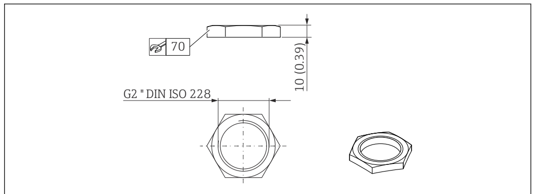
图 22 锁紧螺母的外形尺寸。测量单位 mm (in)
