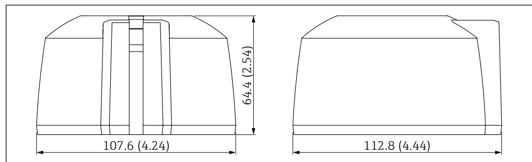
图 20 G1/NPT1 防护罩的外形尺寸 (顶部电缆入口)。测量单位 mm (in)
