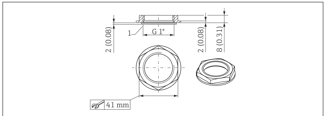
图 17 外形尺寸示意图；锁紧螺母，顶部电缆入口过程连接。测量单位 mm (in)
