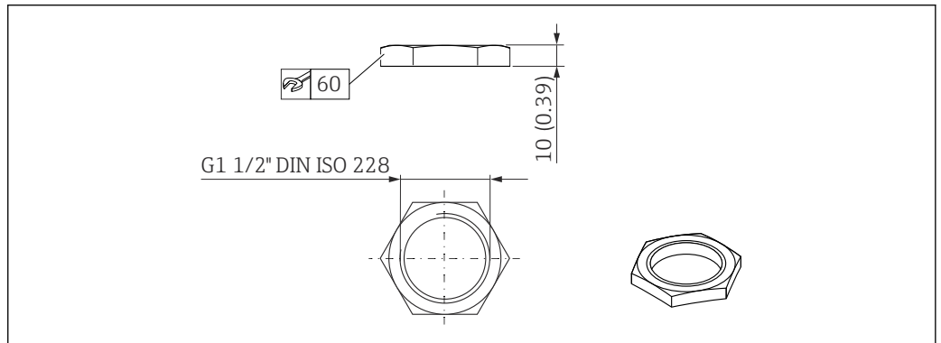
图 21 锁紧螺母的外形尺寸。测量单位 mm (in)
