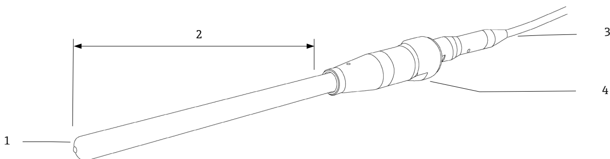
图 8. Rxn-40 探头，不带法兰过程连接
