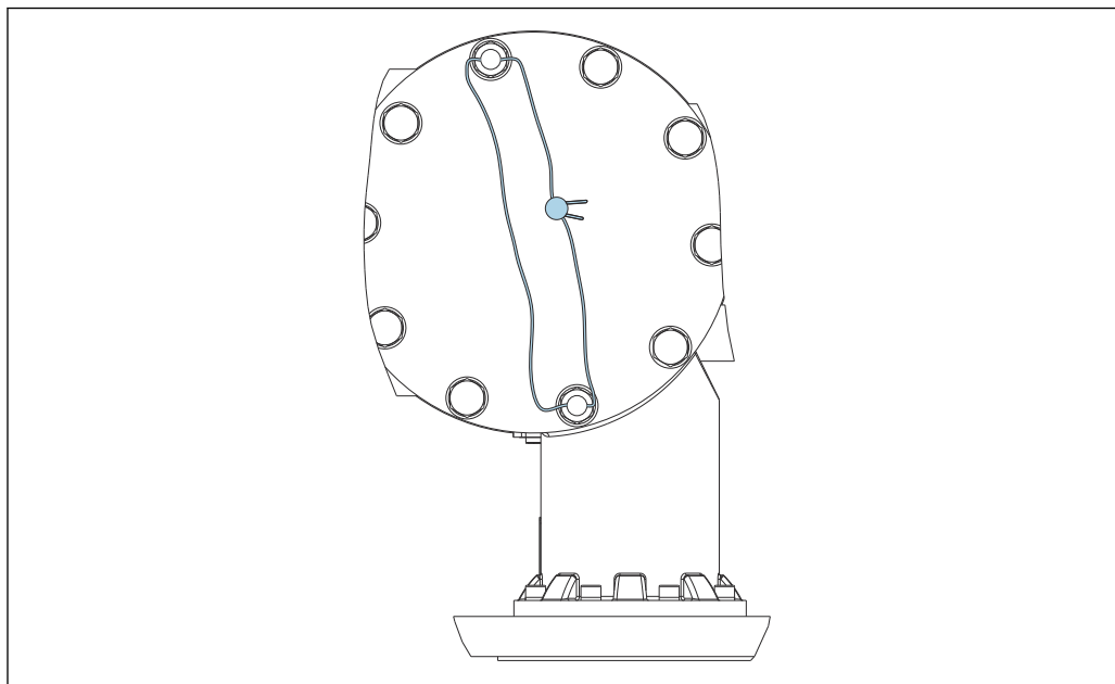
37 Пломбирование задней крышки (на примере NMS81/NMS83)
