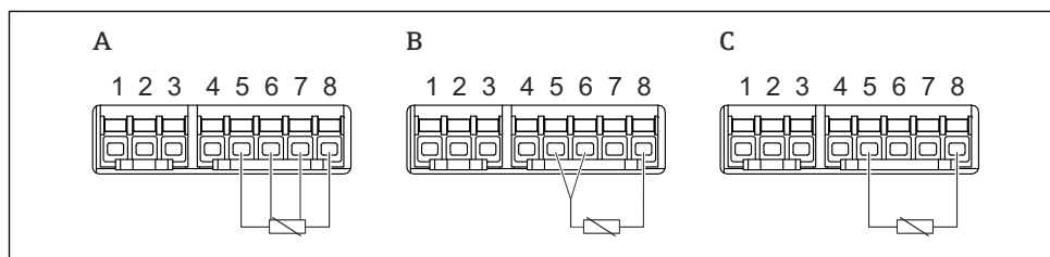
66 Типы подключений RTD
