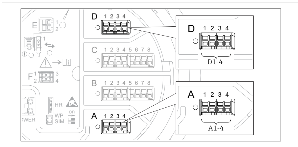
77 Возможное расположение модулей WM550 (примеры); в зависимости от исполнения прибора данные модули также могут находиться в гнезде B или C → 51.
