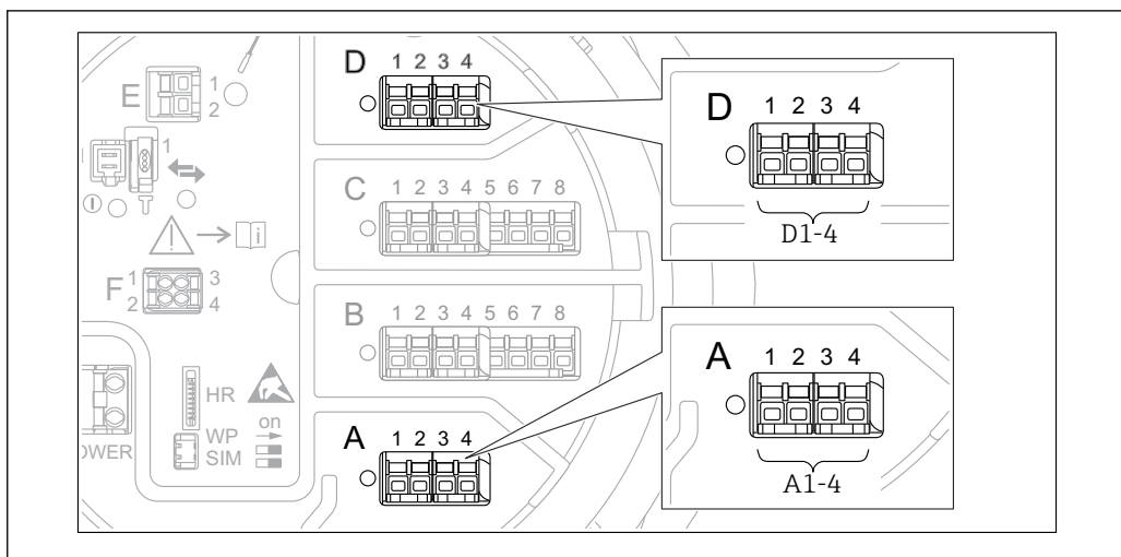
76 Возможное расположение модулей V1 (примеры); в зависимости от исполнения прибора данные модули также могут находиться в гнезде B или C → 51.
