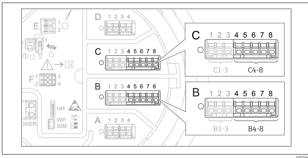
91 Клеммы для подменю "Analog IP" (B4-8 или C4-8, соответственно)
