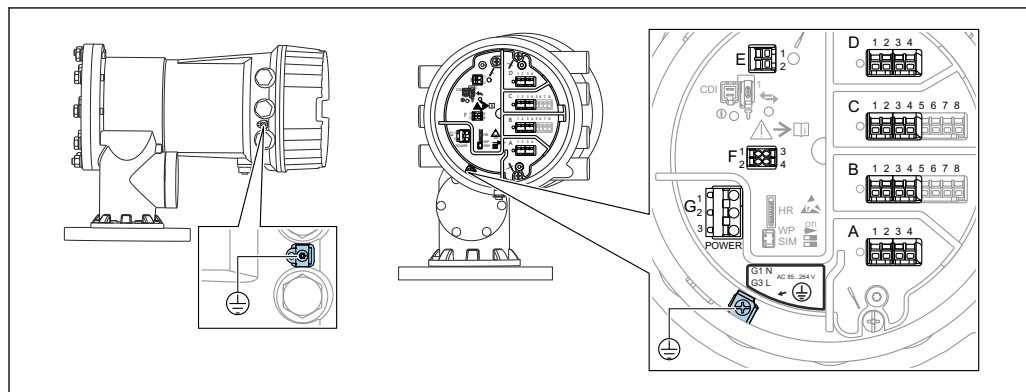
19 Клемный отсек (типовой пример) и клеммы заземления
