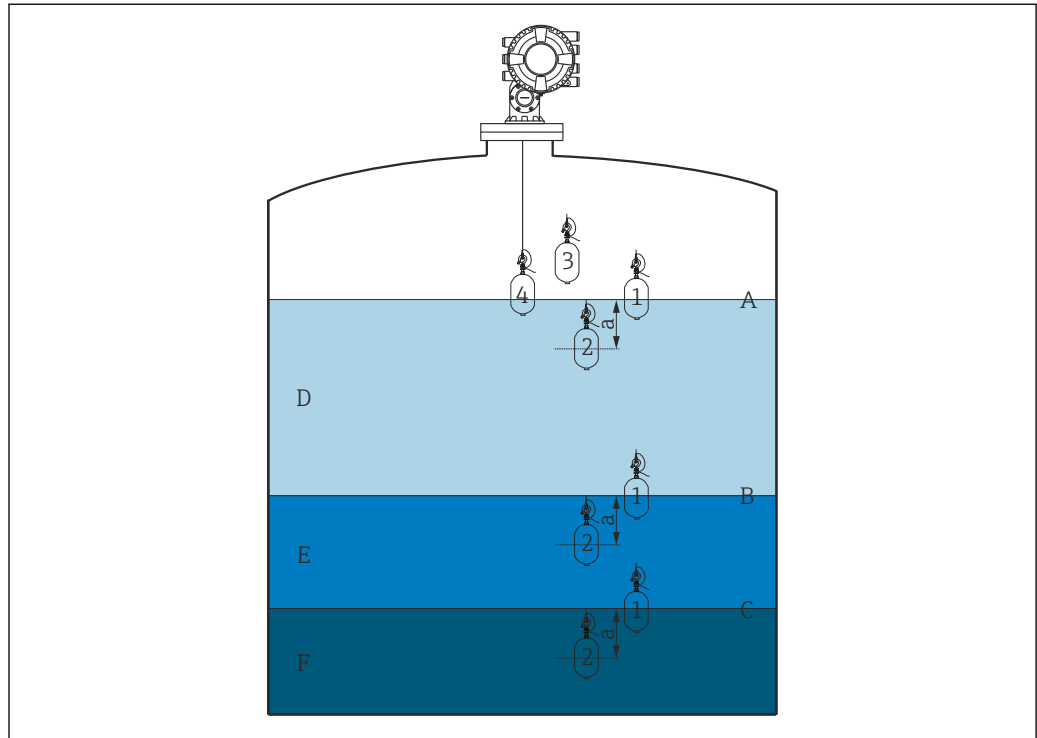
55 Точечная плотность (числа обозначают последовательность движения поплавка)
