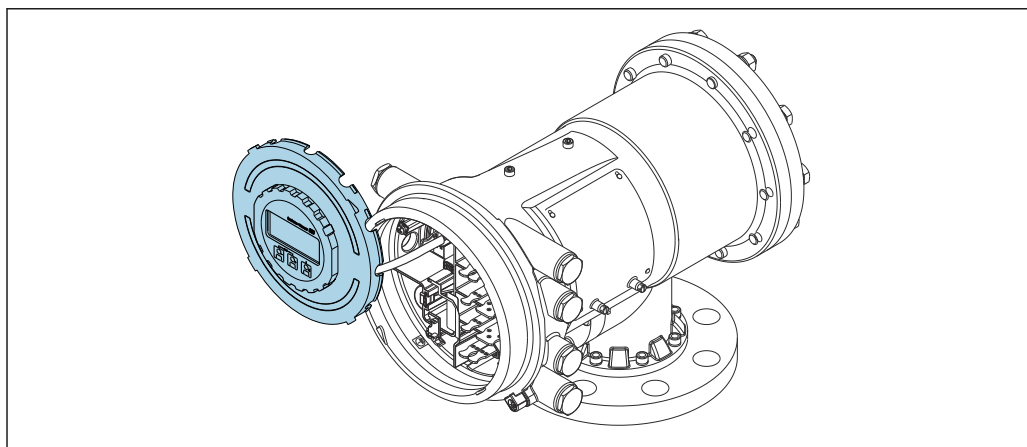
38 NMS81: дисплей прижат к краю клеммного отсека
