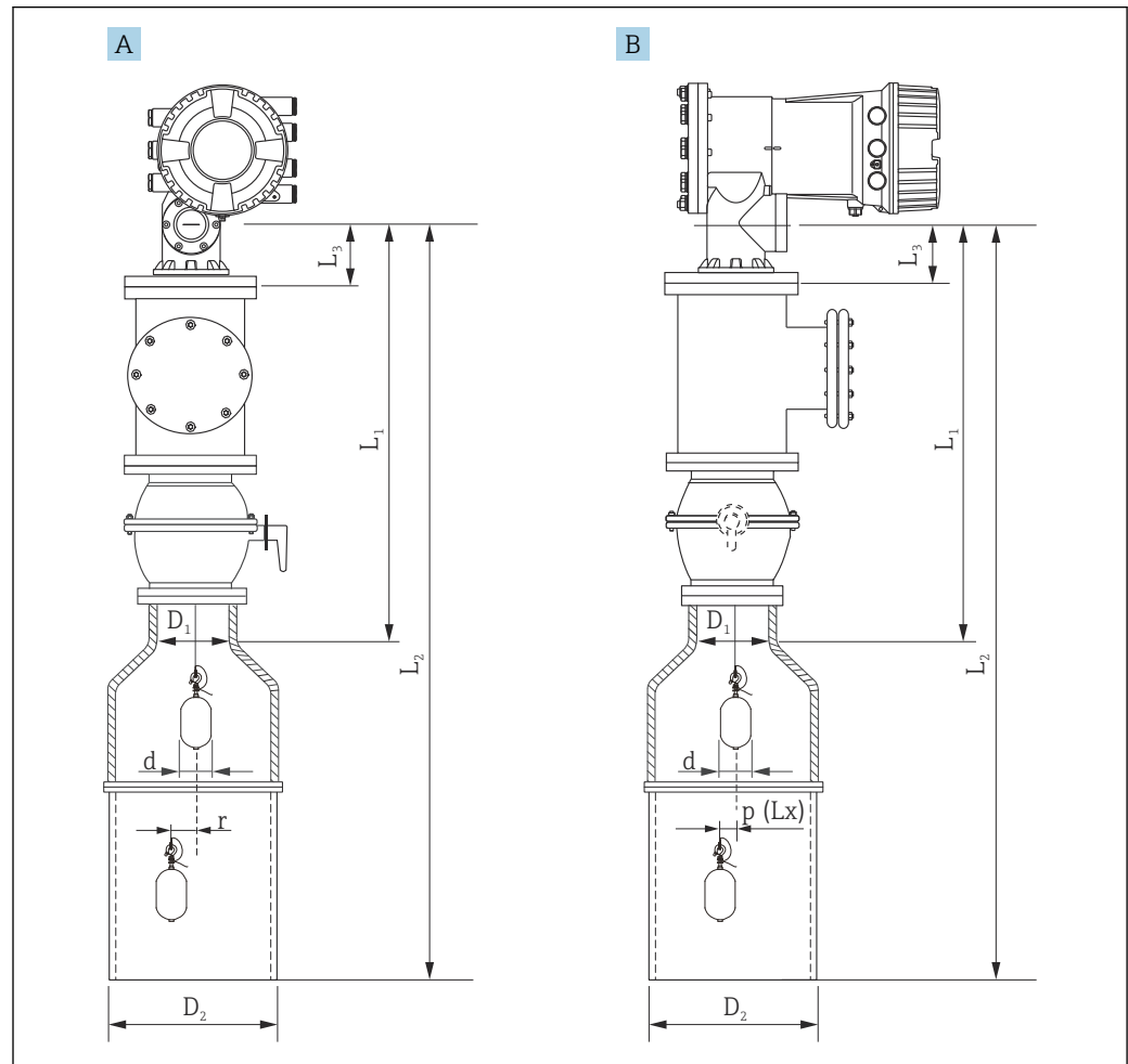
6 Монтаж с концентрической успокоительной трубой
