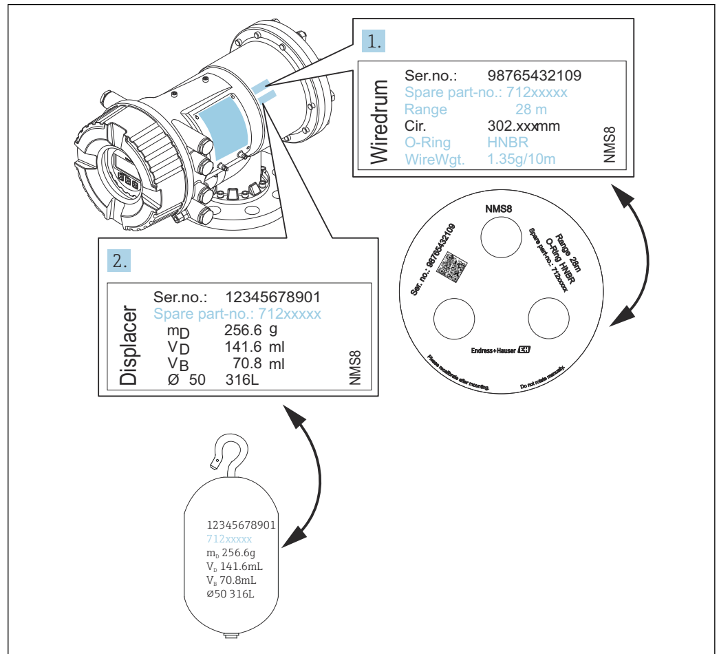
15 Проверка поплавка и барабана с тросом A0028025
