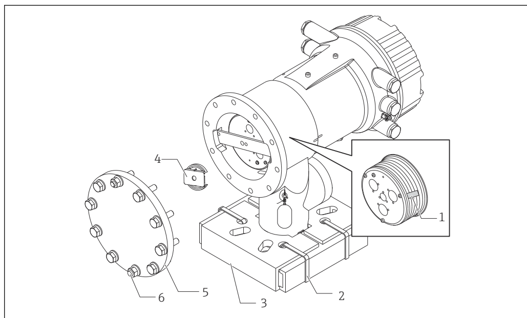
16 Снятие упаковочных материалов
