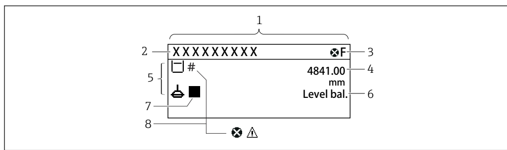
31 Типичный внешний вид основного экрана (отображение измеренного значения)
