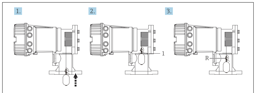
46 Последовательность калибровки точки отсчета
