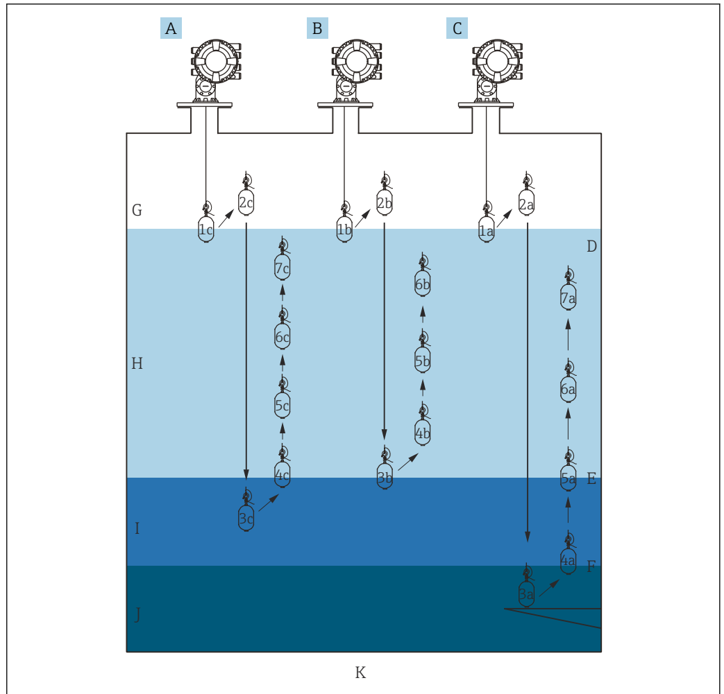
56 Обзор профиля плотности (обозначения 1a, 2a, 3a... соответствуют последовательности перемещений поплавка)
