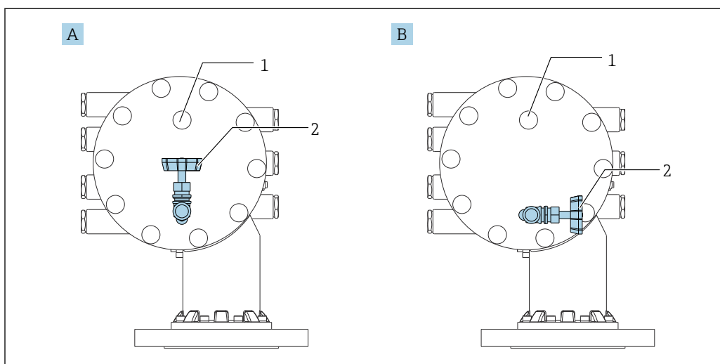
87 Очистительный патрубок и перепускной клапан
