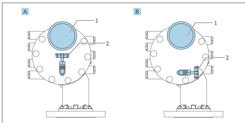
83 Монтажная позиция перепускного клапана и манометра
