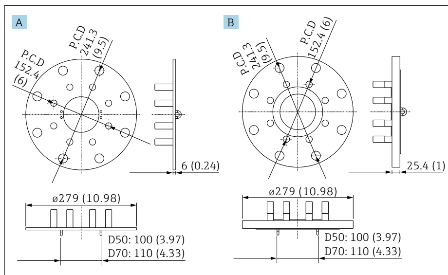
11 Размеры переходной пластины
