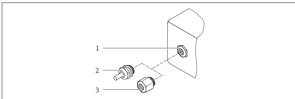
23 Возможные варианты кабельных вводов/кабельных уплотнений
