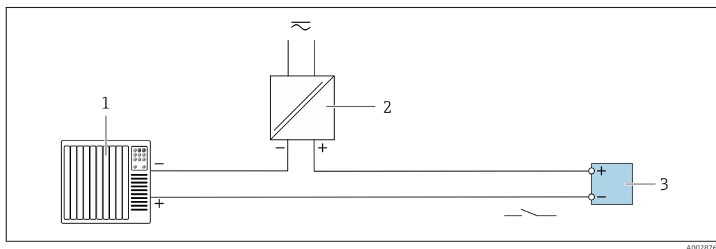
9 Пример подключения для релейного выхода (пассивного)
