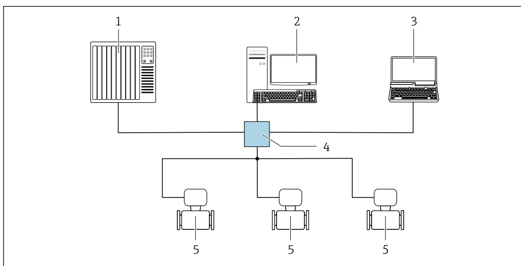
15 Варианты дистанционного управления через сеть EtherNet/IP: топология «звезда»
