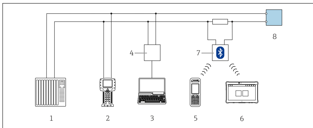
16 Варианты дистанционного управления по протоколу HART
