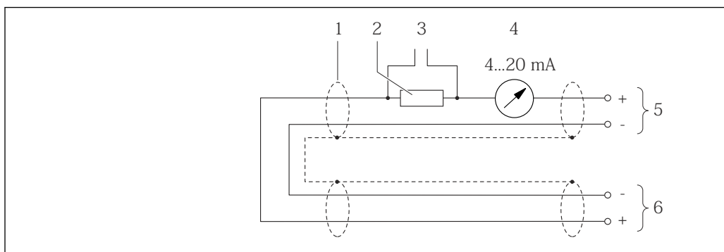
13 Пример подключения для входа HART (в пакетном режиме) через токовый выход (активный)
