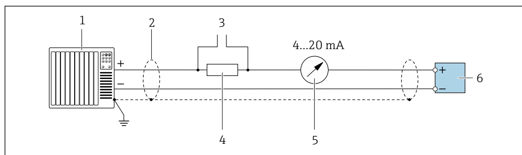
9 Пример подключения токового выхода 4-20 мА HART (активного)
