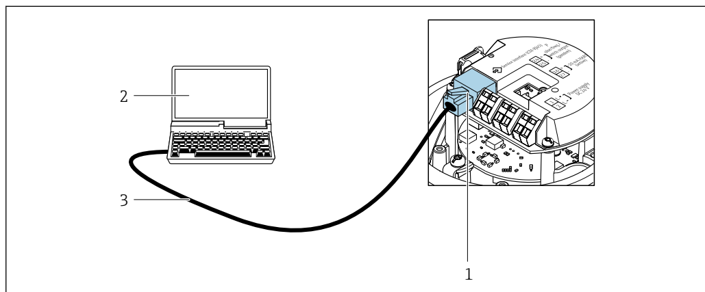
17 Подключение для кода заказа «Выход», опция В «4-20 мА HART, импульсный/частотный/релейный выход»
