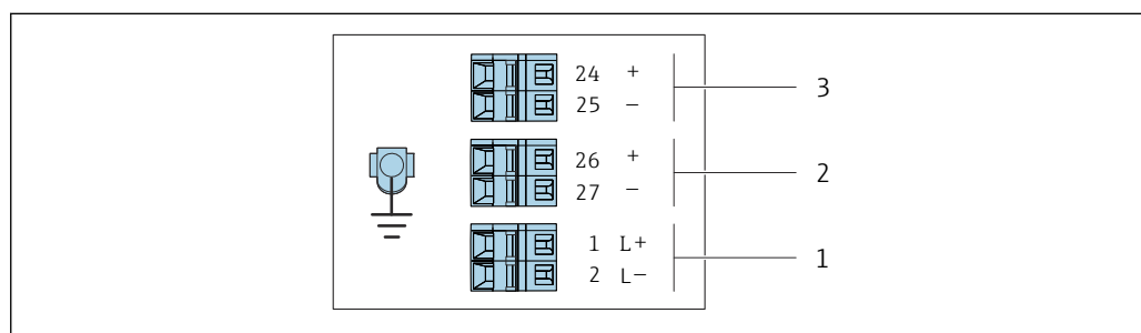
6 Назначение клемм: 4–20 мА HART с импульсным/частотным/релейным выходом
