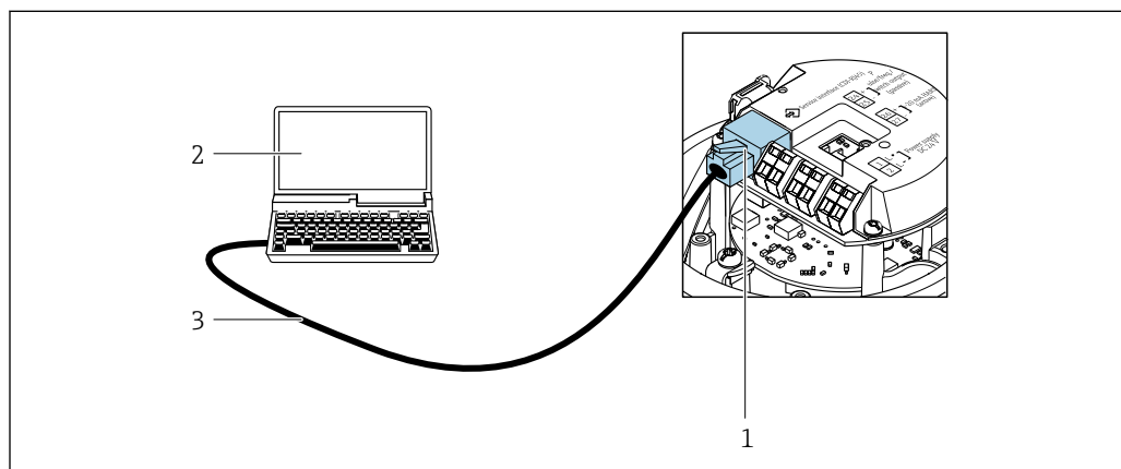
20 Подключение для кода заказа «Выход», опция В «4-20 мА HART, импульсный/частотный/релейный выход»
