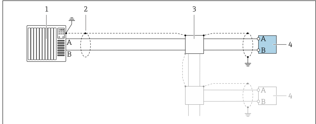
14 Пример подключения для Modbus RS485, безопасная зона и зона 2/разд. 2
