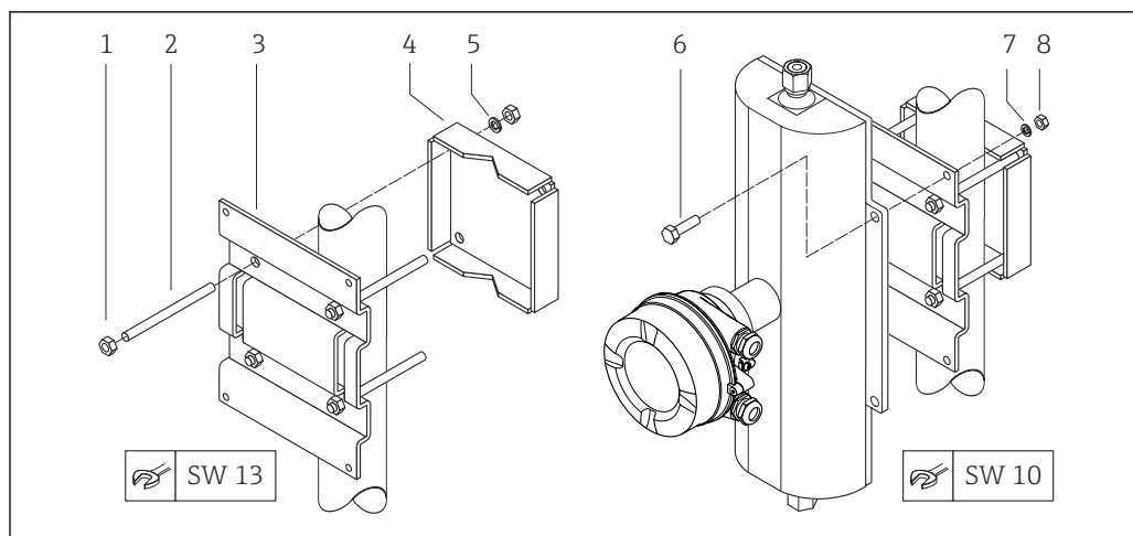
6 Комплект держателя для монтажа на опоре
