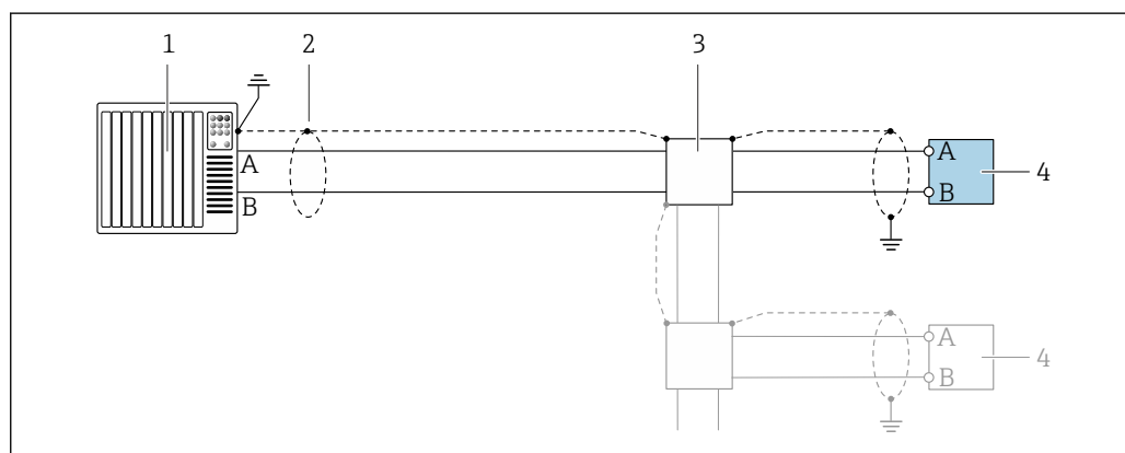
10 Пример подключения для PROFIBUS DP, невзрывоопасная зона и зона 2/разд. 2
