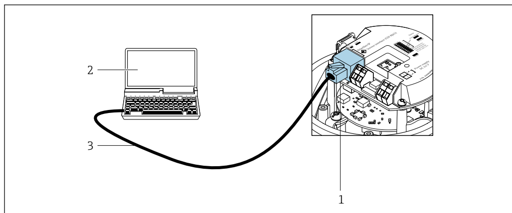
19 Подключение для кода заказа «Выход», опция L «PROFIBUS DP»
