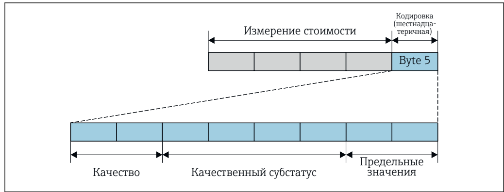
16 Структура байта кодирования
