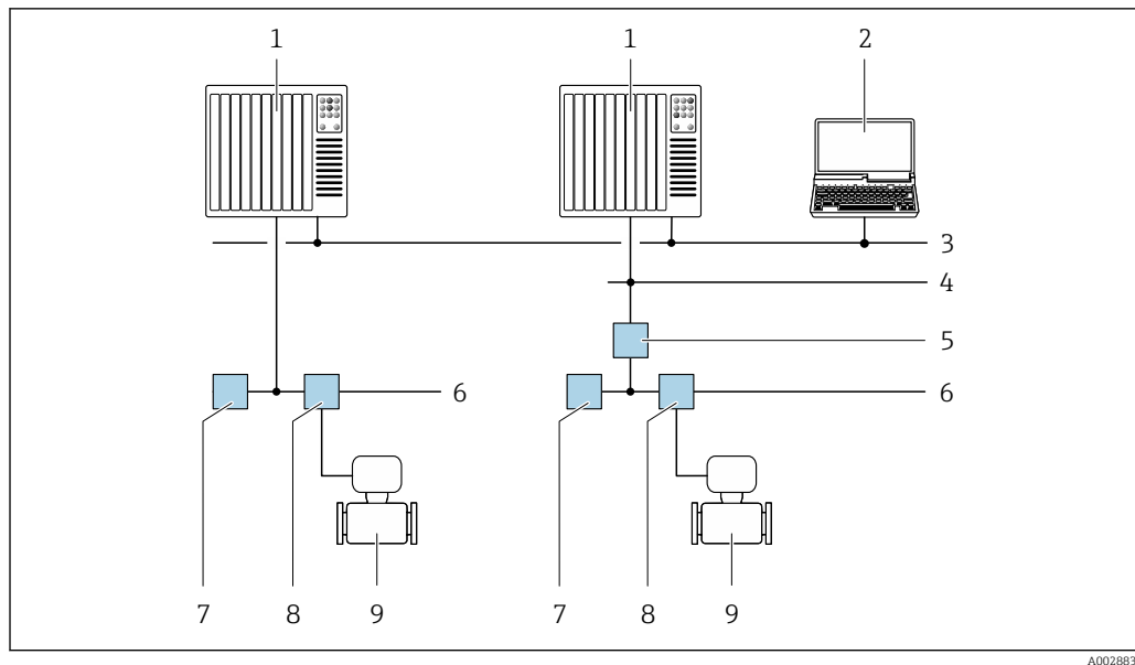
21 Варианты дистанционного управления через сеть FOUNDATION Fieldbus
