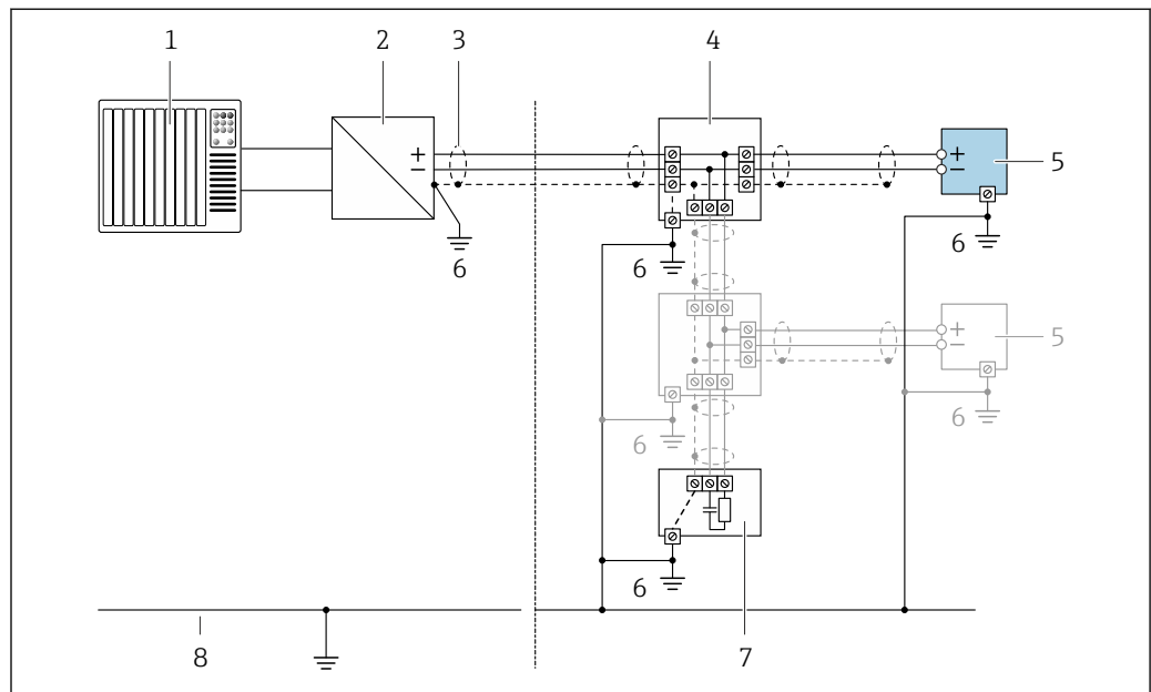
7 Пример подключения для FOUNDATION Fieldbus
