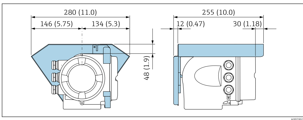
11 Защитный козырек от погодных явлений для прибора Proline 500; единицы измерения – мм (дюймы)
