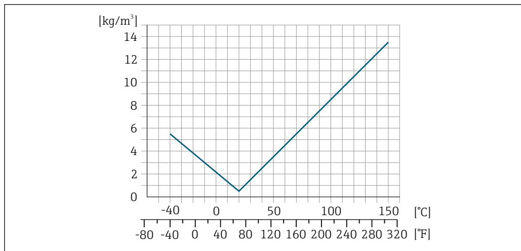
43 Калибровка по плотности на месте эксплуатации, в примере – при температуре +20 °C (+68 °F)
