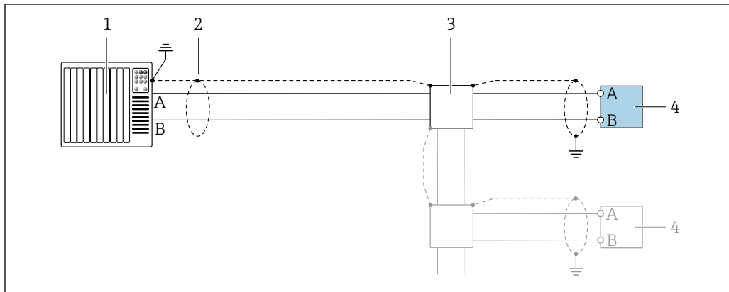
19 Пример подключения для Modbus RS485, невзрывоопасная зона и зона 2; класс I, раздел 2
