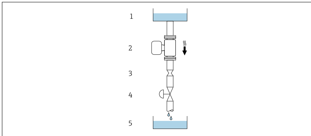
7 Монтаж в трубопроводе с нисходящим потоком (например, для дозирования)
