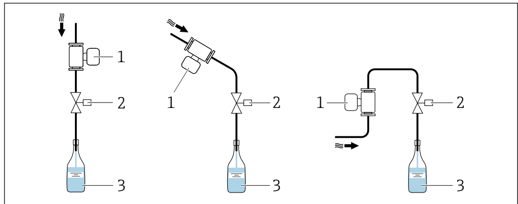
7 Система дозирования
