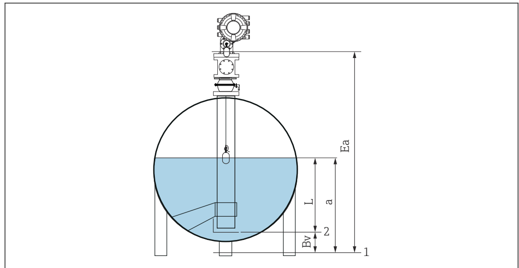
53 Geschlossener Tank für NMS80 und NMS81
