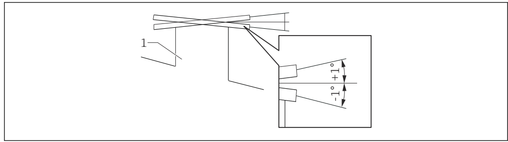
13 Zulässige Neigung des Montageflansches
