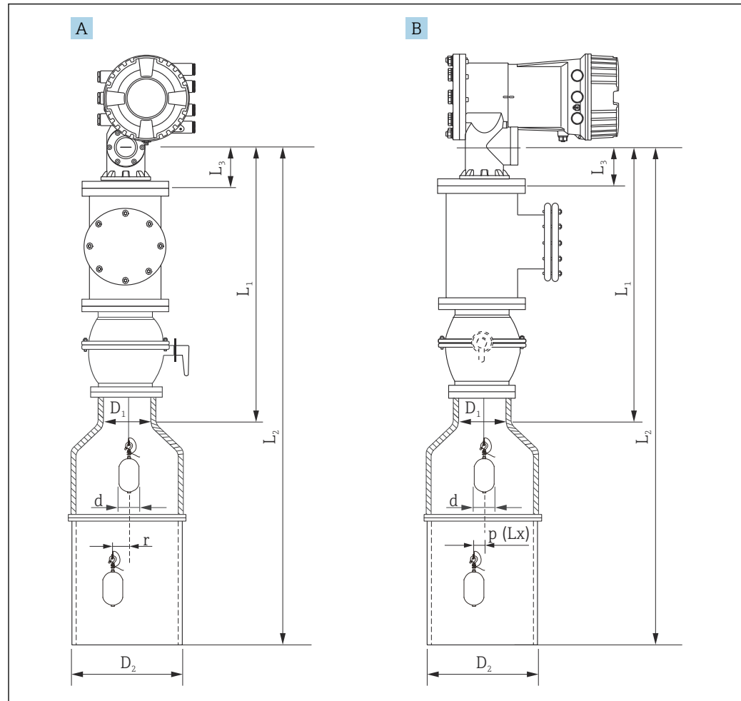
6 Montage mit konzentrischem Schwallrohr
