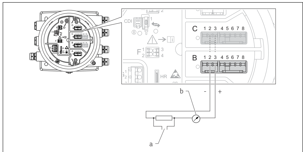
26 Aktive Nutzung des Analog I/O-Moduls im Ausgangsmodus
