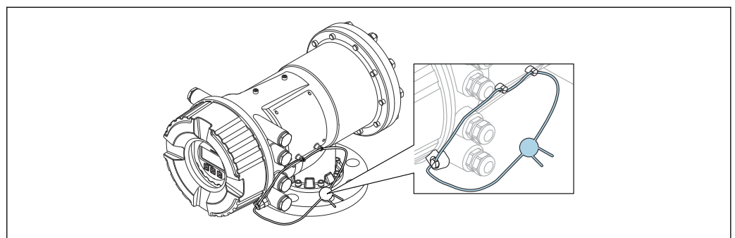
36 Versiegelung des Anschlussklemmenraumdeckels
