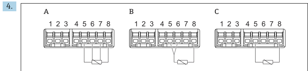
66 RTD-Anschlussarten
