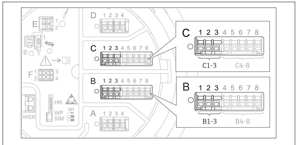
72 Mögliche Positionen der Analog I/O-Module, die als 4...20mA-Ausgang verwendet werden können. Der Bestellcode des Geräts legt fest, welches dieser Module tatsächlich vorhanden ist → 49.
