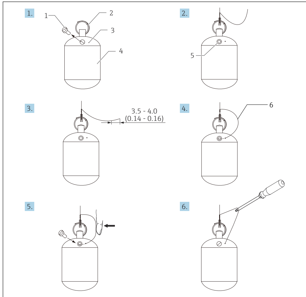
18 Montage des PTFE-Verdrängers; Maßangabe mm (in)
