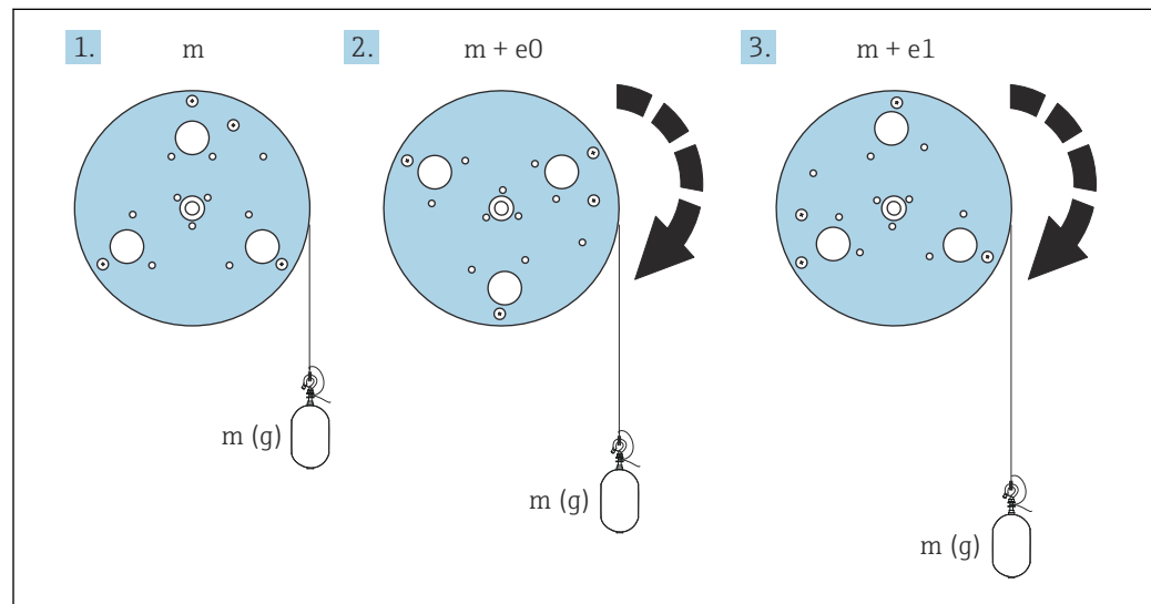
47 Messgewicht
