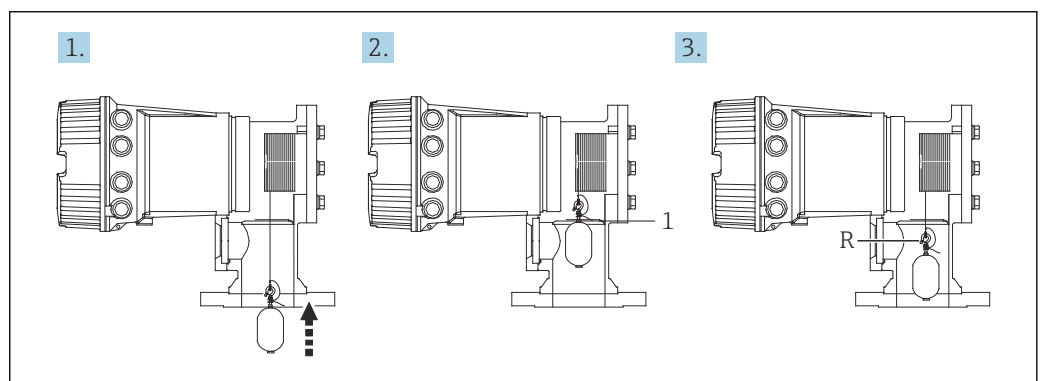
46 Ablauf Referenzkalibrierung
