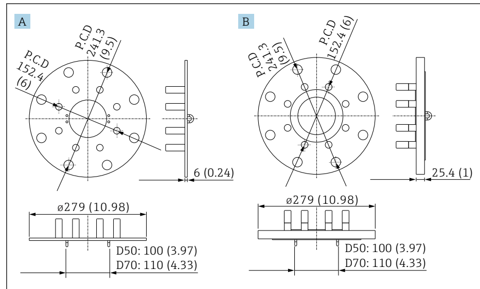
11 Abmessungen Reduzierplatte
