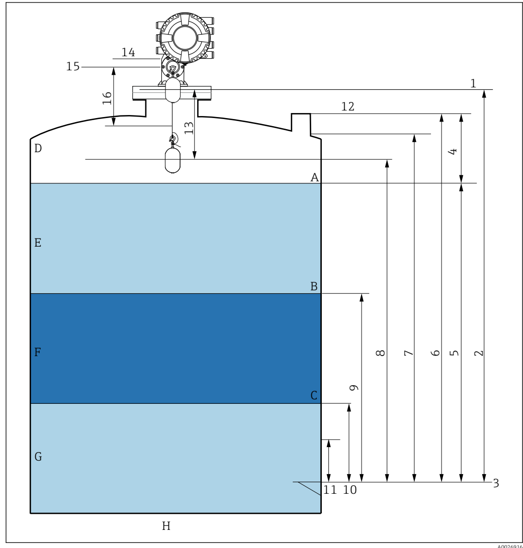
42 Auf die NMS8x-Montage bezogene Begriffe (z. B. NMS81)
