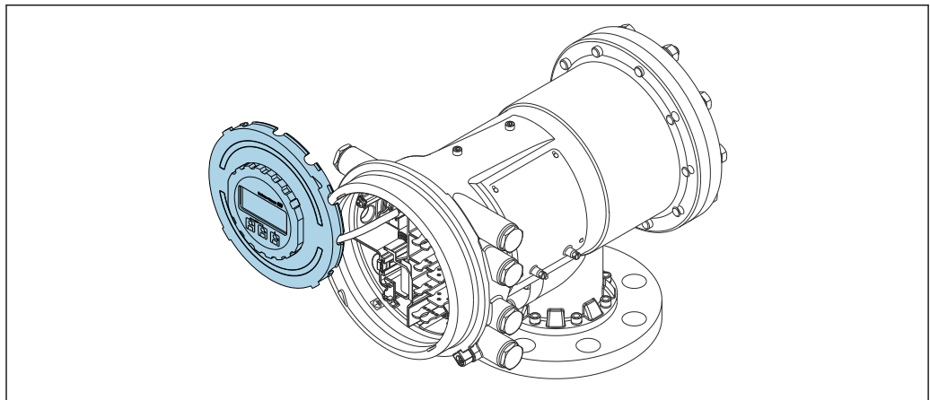
38 NMS81: Anzeigemodul steckt am Rand des Anschlussklemmenraums
