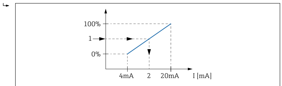
73 Tankvariable auf den Ausgangsstrom skalieren
