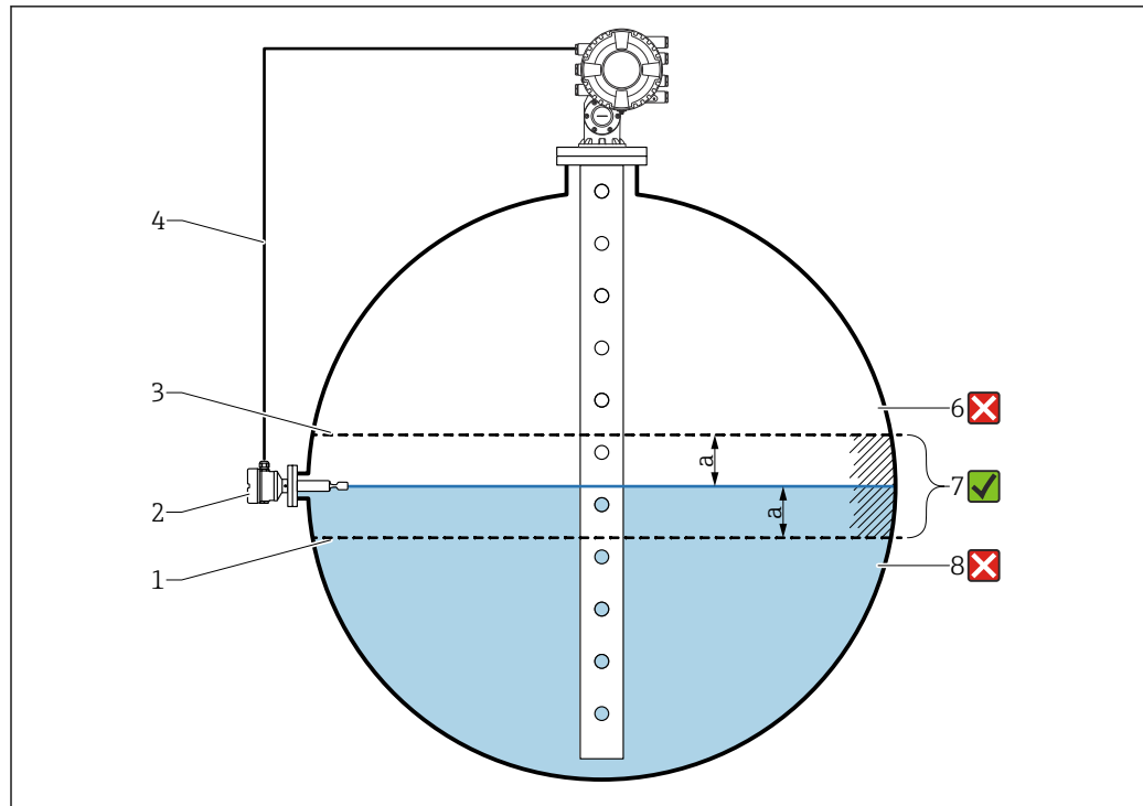
70 Anwendungsbeispiel mit Füllstandsgrenzschalter
