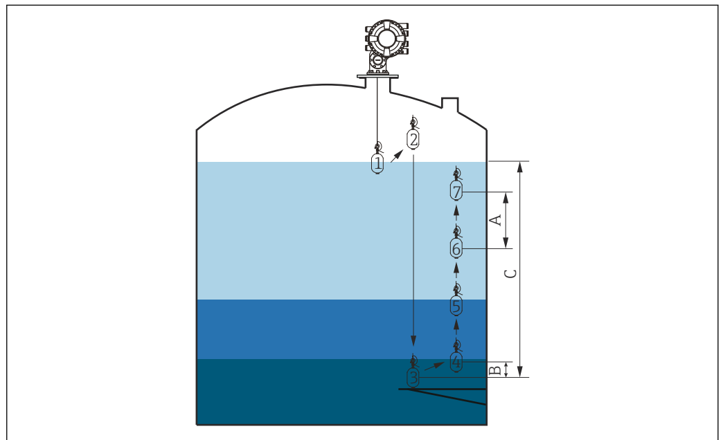
57 Bewegungsabfolge Tankprofil-Messung (die Zahlen zeigen die Abfolge der Verdrängerbewegung an)
