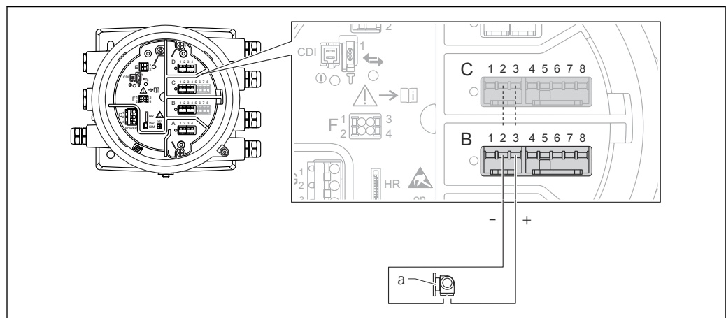
27 Aktive Nutzung des Analog I/O-Moduls im Eingangsmodus
