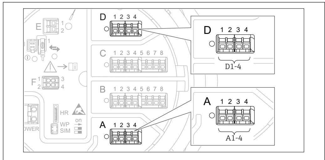
96 Bezeichnung der "Modbus"-, "V1"- oder "WM550"-Module (Beispiele); diese Module können je nach Geräteausführung auch in den Slots B oder C sitzen.
