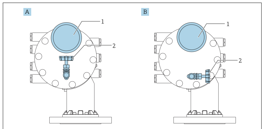
83 Montelage von Überdruckventil und Druckanzeiger
