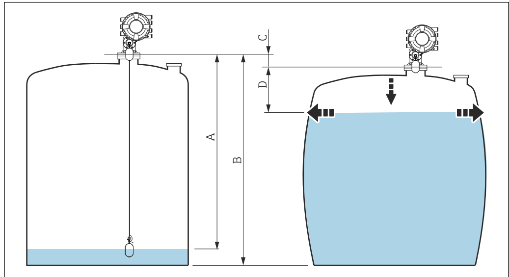
68 Korrektur der hydrostatischen Tankdeformation (HyTD)
