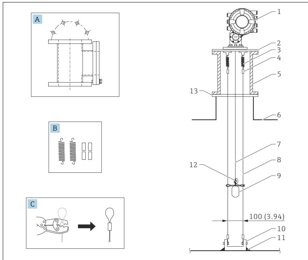
9 Führungsdraht; Maßangabe mm (in)
