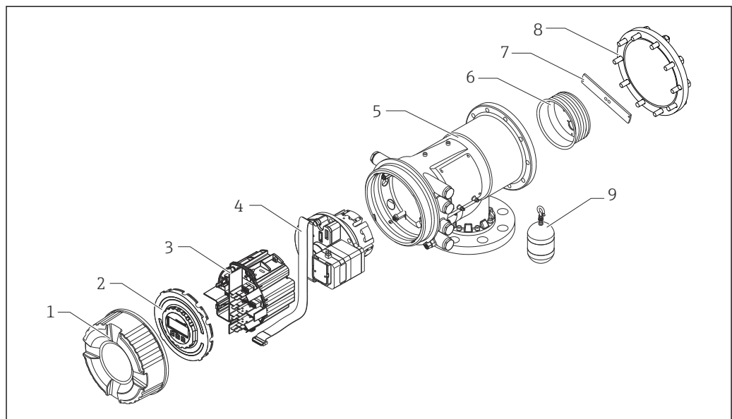
2 Konfiguration des NMS81
