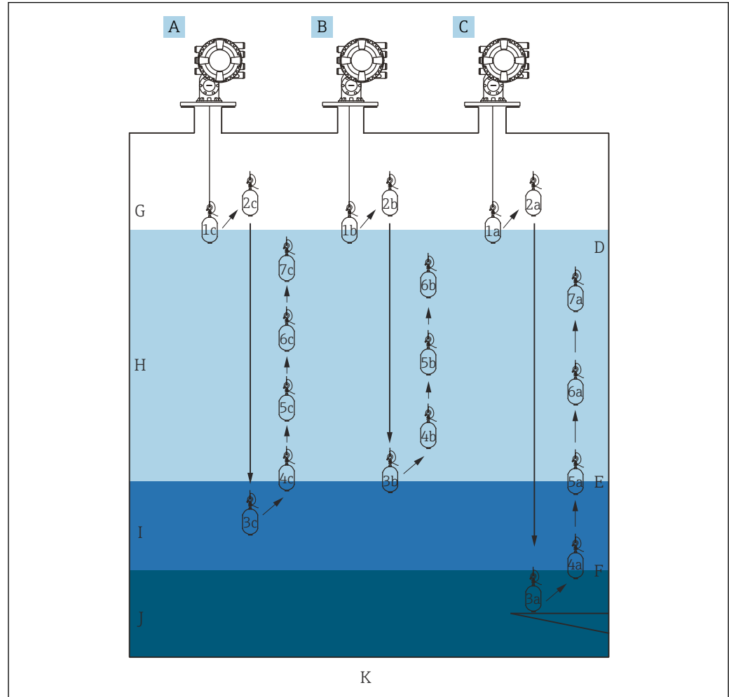
56 Übersicht über die Profildichte (1a, 2a, 3a ... zeigen die Abfolge der Verdrängerbewegung an)
