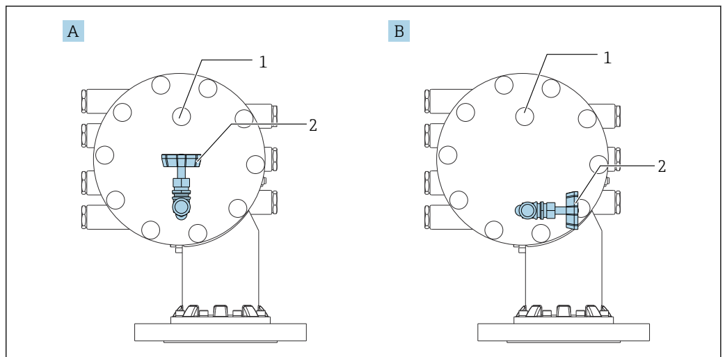
87 Reinigungsdüse und Überdruckventil
