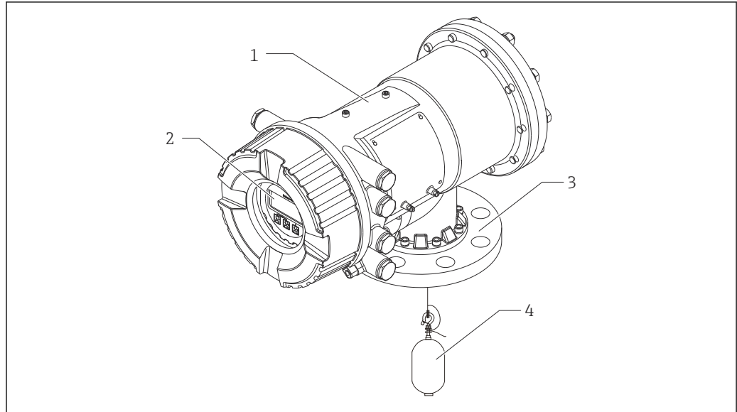
1 Aufbau des Proservo NMS81
