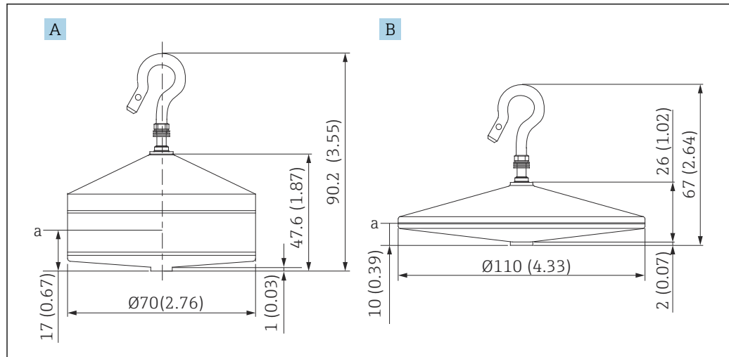
A \varnothing 70 mm (2,76 in) 316L, konischer Verdränger B \varnothing 110 mm (4,33 in) 316L, konischer Verdränger a Eintauchpunkt
