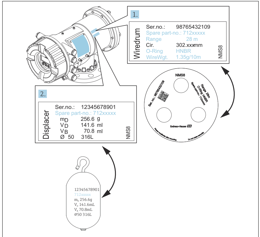
15 Verifizierung von Verdränger und Messtrommel
