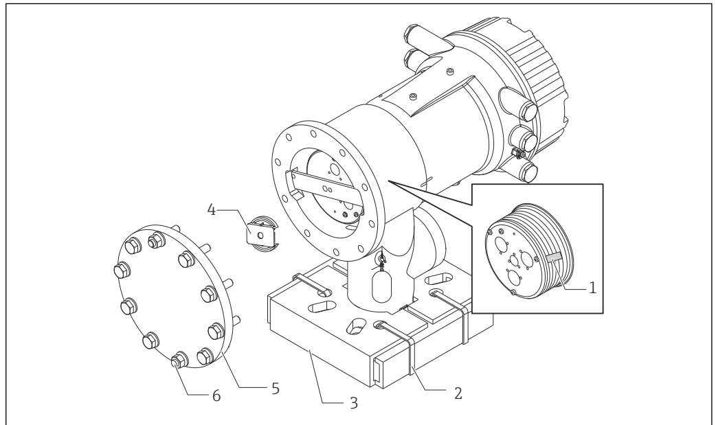
16 Entfernen der Verpackungsmaterialien
