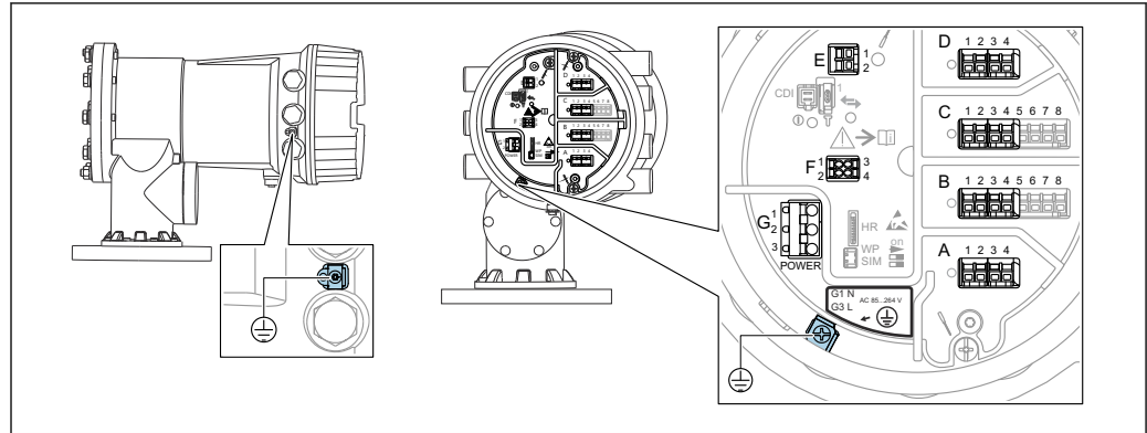
19 Anschlussklemmenraum (typisches Beispiel) und Erdungsklemmen
