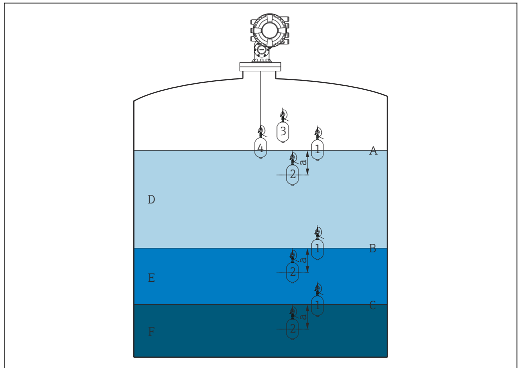
55 Punktdichte (die Zahlen zeigen die Abfolge der Verdrängerbewegung an)
