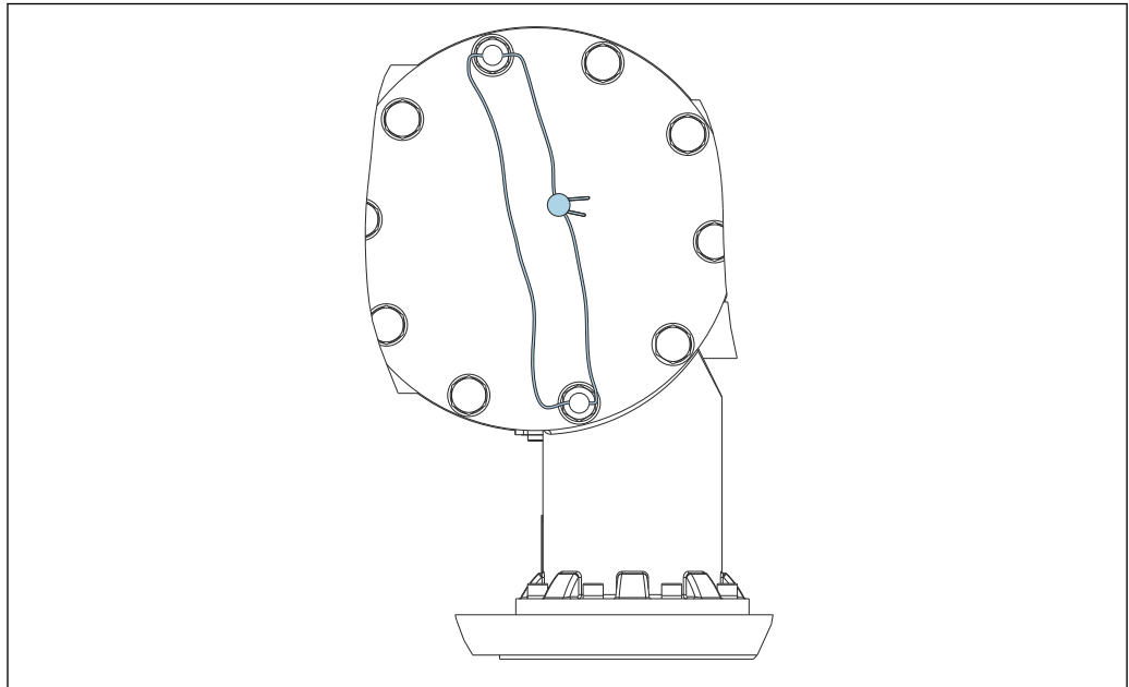
37 Versiegelung der rückwärtigen Abdeckung (z. B. NMS81/NMS83)
