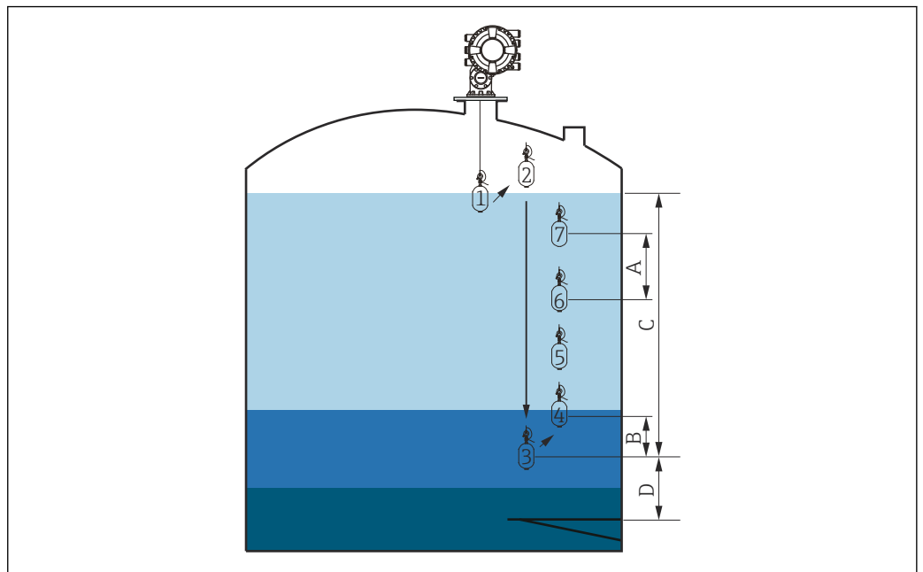
59 Bewegungsabfolge manuelle Profilmessung (die Zahlen zeigen die Abfolge der Verdrängerbewegung an)
