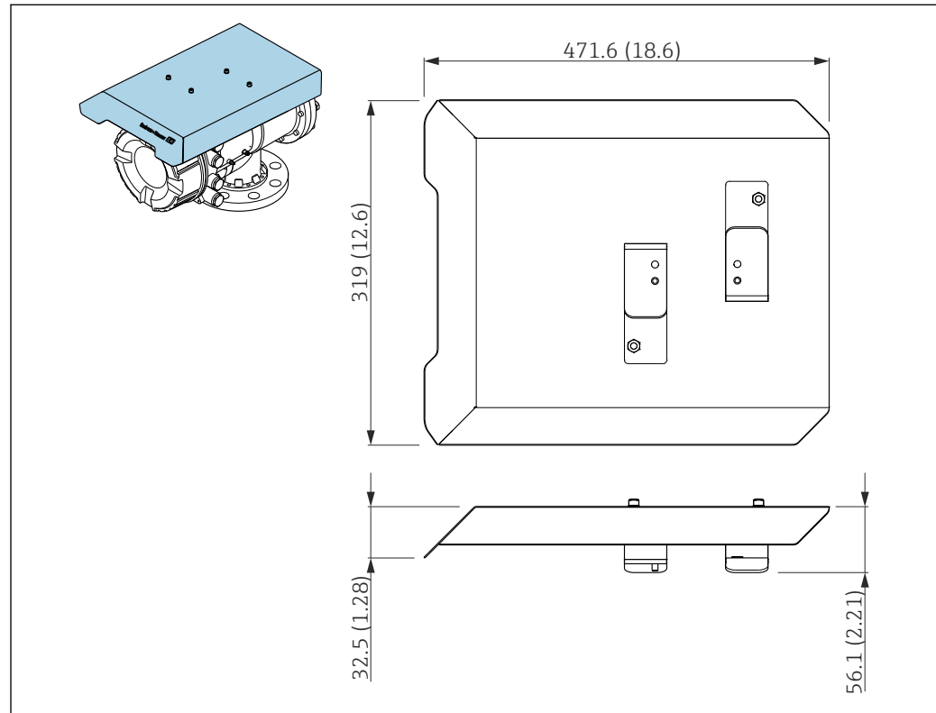
82 Wetterschutzhaube; Abmessungen: mm (in)
