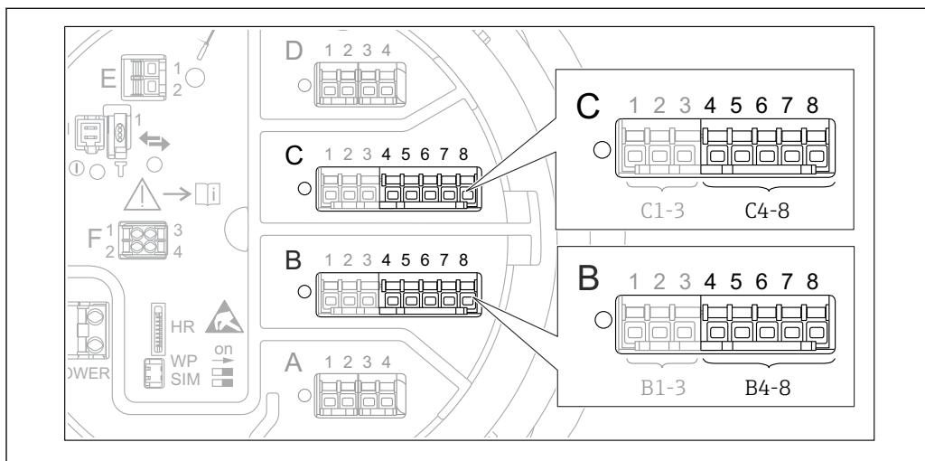
84 Клеммы для подменю "Analog IP" (B4-8 или C4-8, соответственно)
