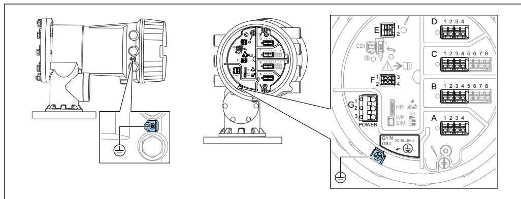
12 Клемный отсек (типовой пример) и клеммы заземления
