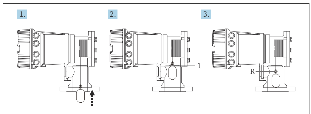
39 Последовательность калибровки точки отсчета
