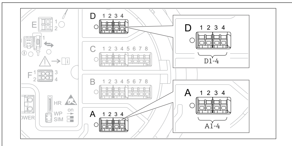
89 Обозначение модулей Modbus, V1 или WM550 (примеры). В зависимости от исполнения прибора эти модули могут находиться в гнезде B или C.
