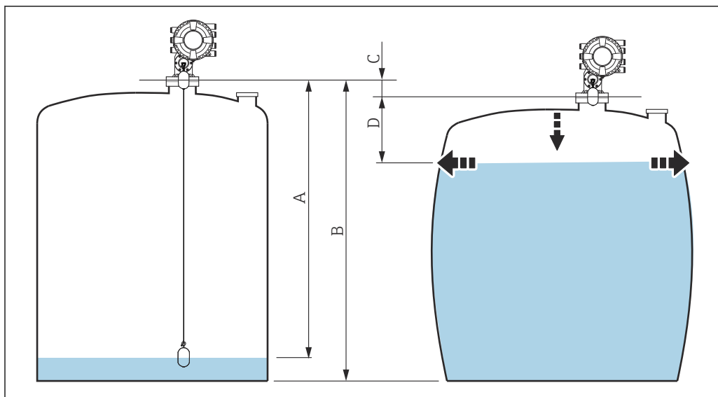
61 Коррекция гидростатической деформации резервуара (HyTD)
