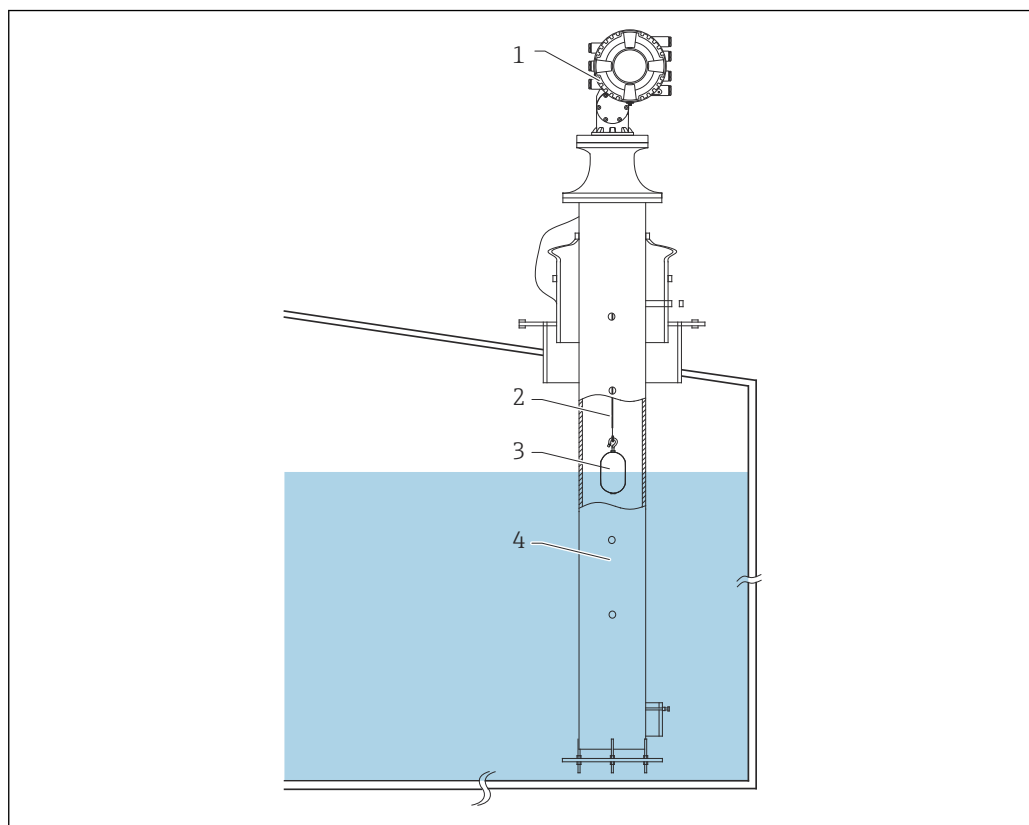
4 Типовой монтаж в резервуаре 1
