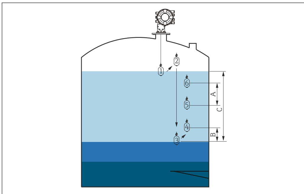
51 Движение при построении профиля границы раздела фаз (числа обозначают последовательность движения поплавка)
