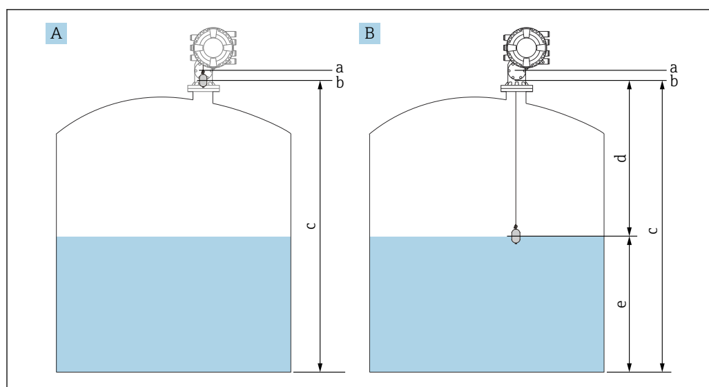
47 Настройка уровня через параметр "Пустой" (NMS83)
