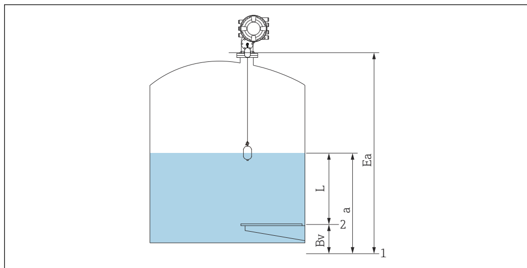
46 Закрытый резервуар для NMS83
