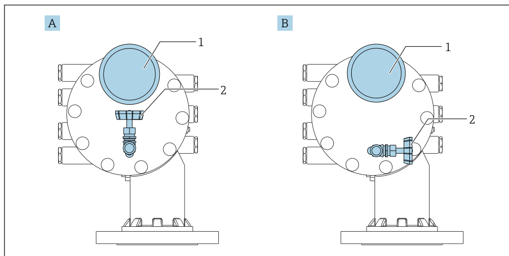
76 Монтажная позиция перепускного клапана и манометра
