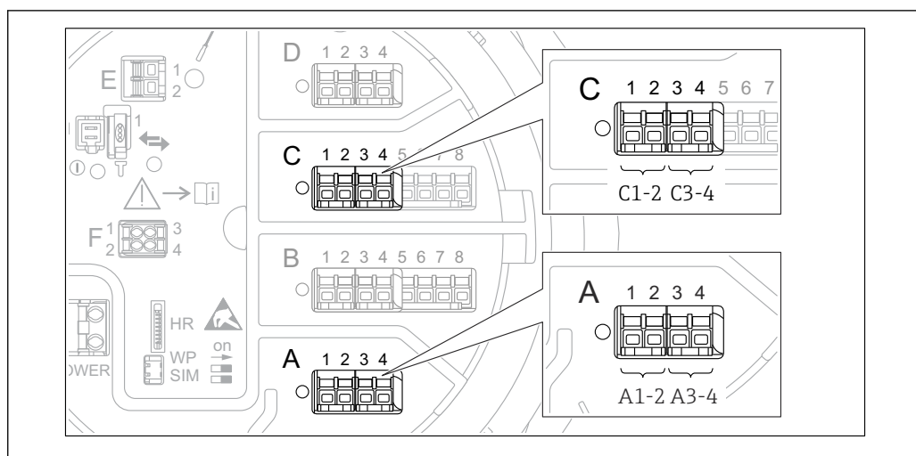
22 Обозначение цифровых входов и выходов (примеры)
