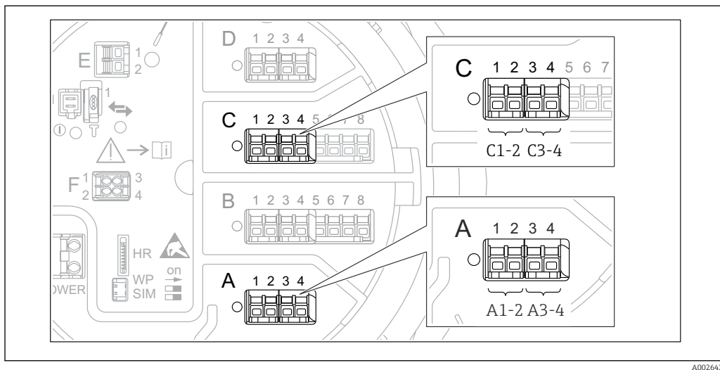
86 Обозначение цифровых входов и выходов (примеры)
