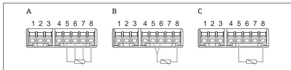
59 Типы подключений RTD
