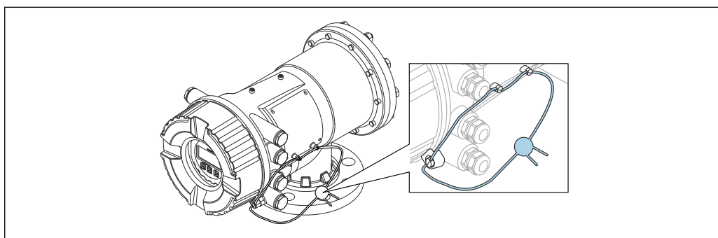
29 Пломбирование крышки клеммного отсека
