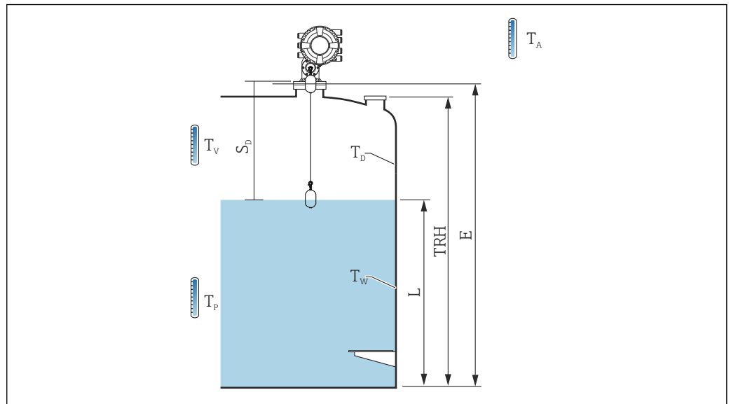
92 Параметры для вычисления значения CTSh
