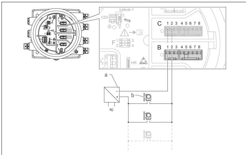
18 Использование модуля аналогового ввода/вывода в режиме пассивного ведущего устройства HART
