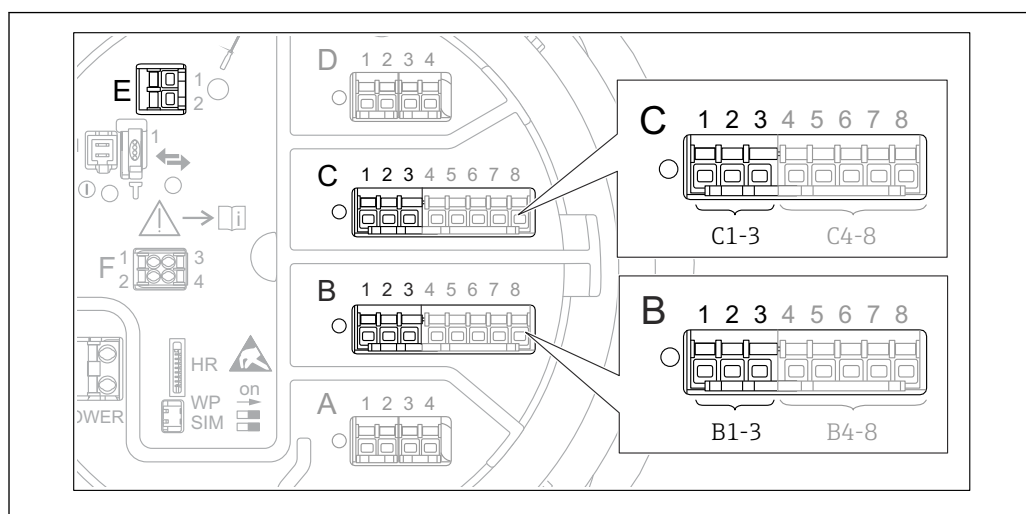
53 Доступные клеммы для цепей HART
