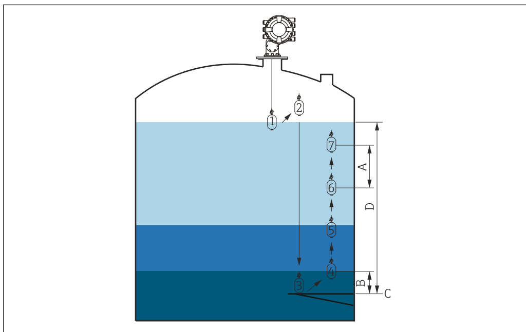
50 Движение при построении профиля резервуара (числа обозначают последовательность движения поплавка)
