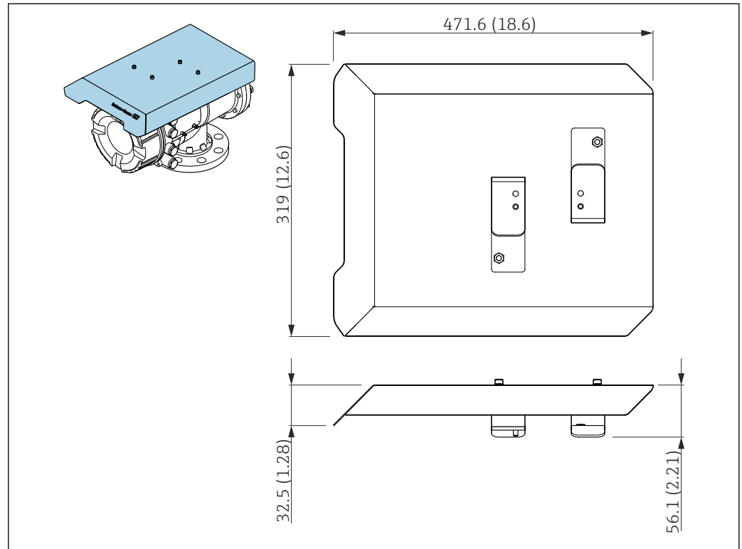
75 Защитный козырек от атмосферных явлений; размеры: мм (дюймы)
