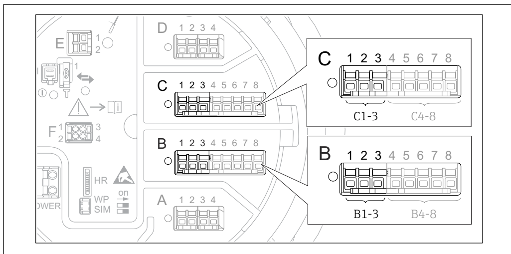
85 Клеммы для подменю "Analog I/O" (B1-3 или C1-3, соответственно)
