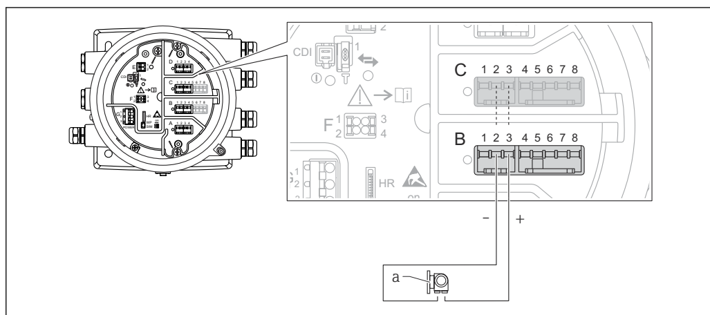
20 Использование модуля аналогового ввода/вывода в режиме активного входа
