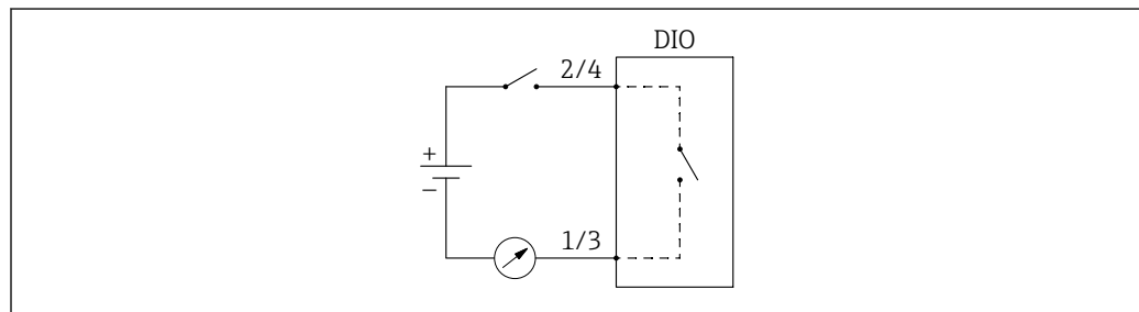
72 Использование цифрового модуля ввода / вывода в качестве цифрового выхода
