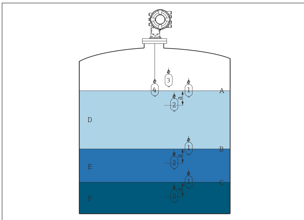
48 Точечная плотность (числа обозначают последовательность движения поплавка)
