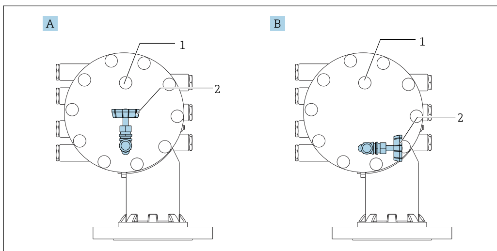
80 Очистительный патрубок и перепускной клапан
