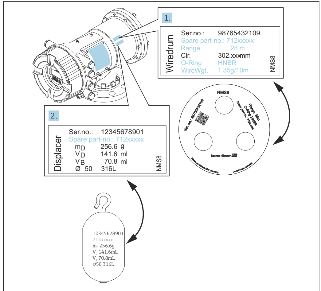
11 Проверка поплавка и барабана с тросом A0029470
