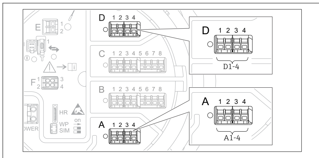
68 Возможное расположение модулей Modbus (примеры); в зависимости от исполнения прибора данные модули также могут находиться в гнезде B или C → 41.
