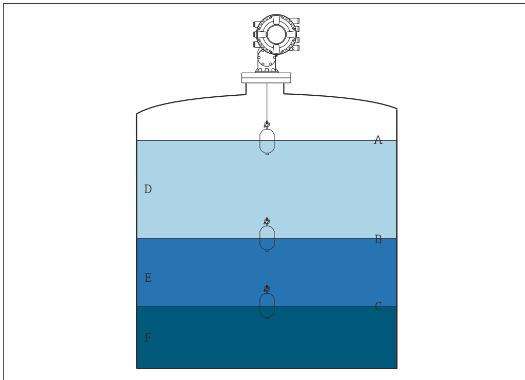
42 Конфигурация резервуара
