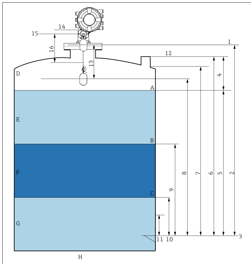
35 Термины, связанные с монтажом прибора NMS8x (на примере NMS81)
