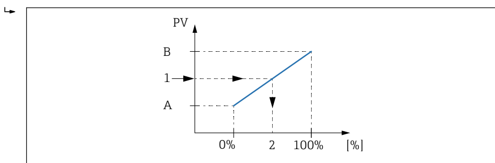
67 Масштабирование переменной резервуара в соответствии с процентным значением
