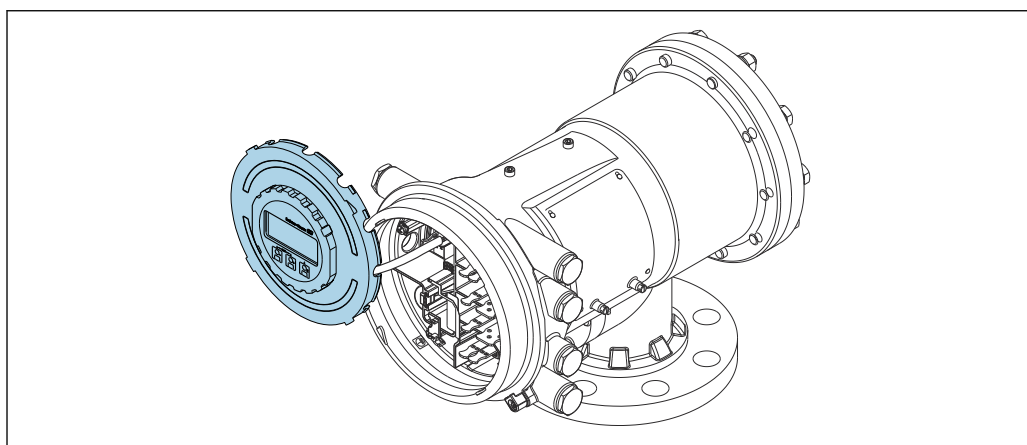
31 NMS83: дисплей прижат к краю клеммного отсека
