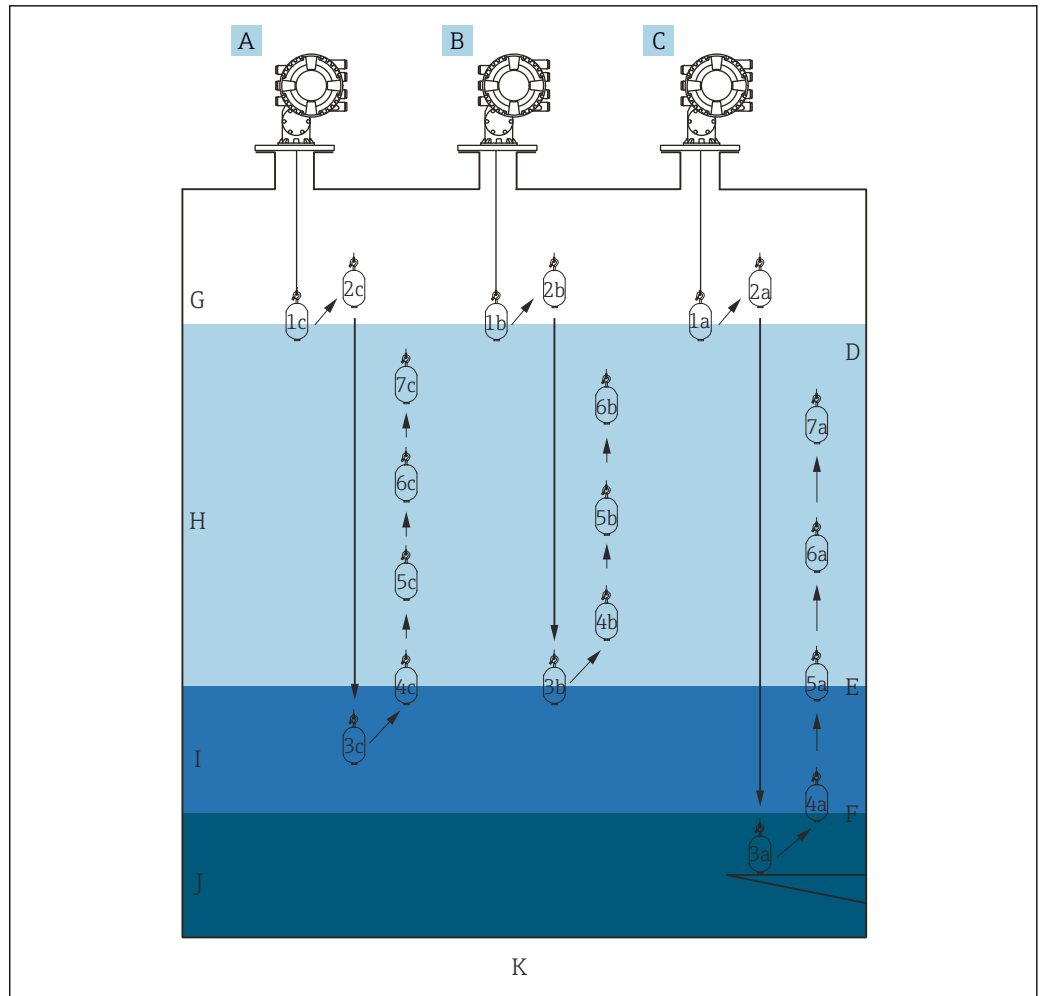
49 Обзор профиля плотности (обозначения 1a, 2a, 3a... соответствуют последовательности перемещений поплавка)
