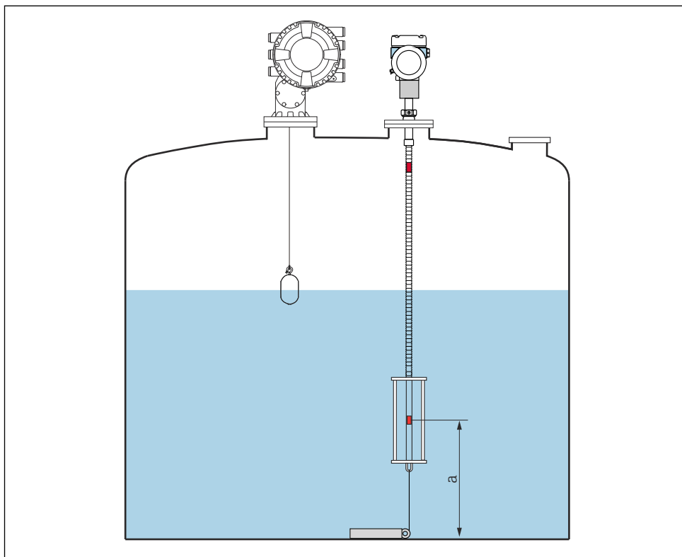
54 Prothermo NMT53x: позиция нижнего температурного элемента
