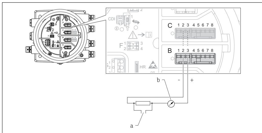
19 Использование модуля аналогового ввода/вывода в режиме активного выхода
