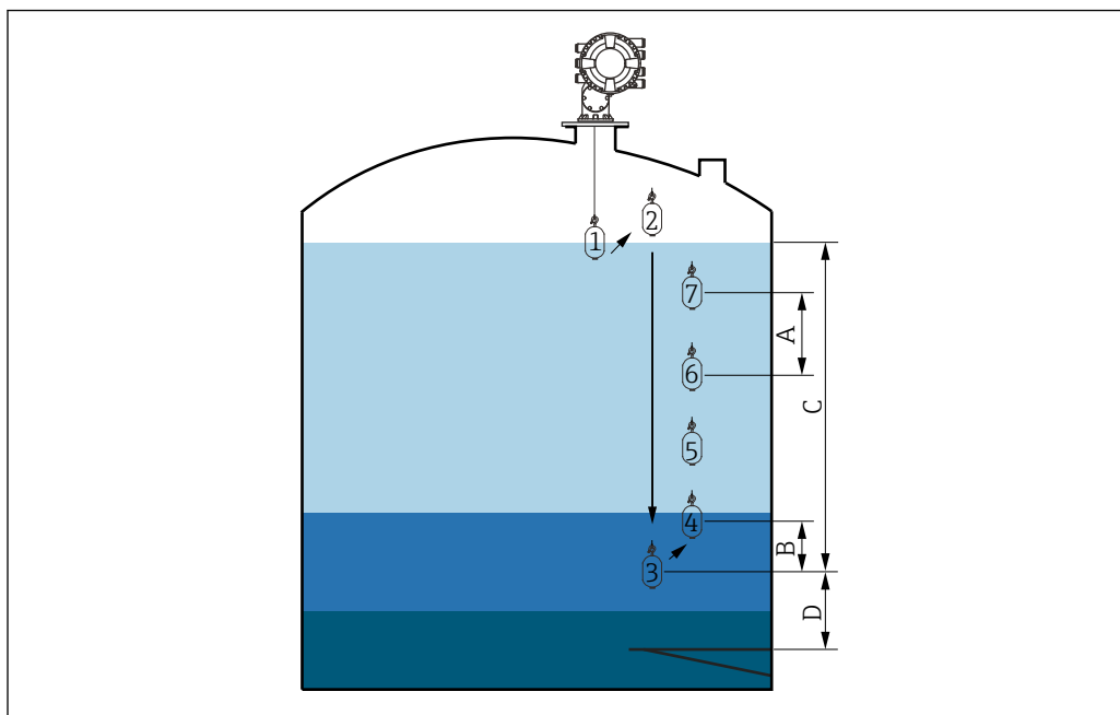
52 Движение при ручном измерении профиля (числа обозначают последовательность движения поплавка)
