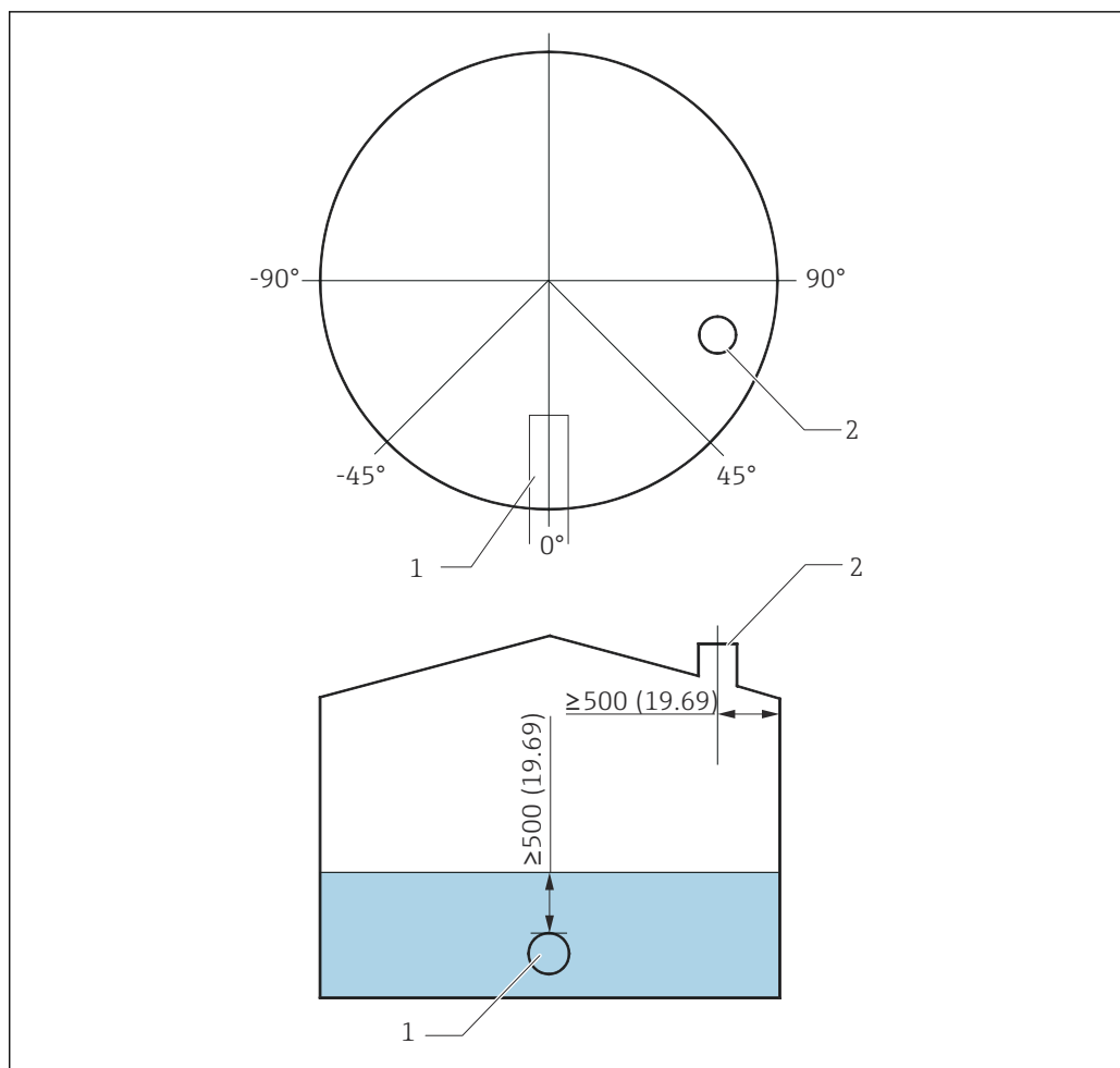
10 Рекомендуемое положение для монтажа прибора NMS8x и минимальный измеряемый уровень, размеры в мм (дюймах)
