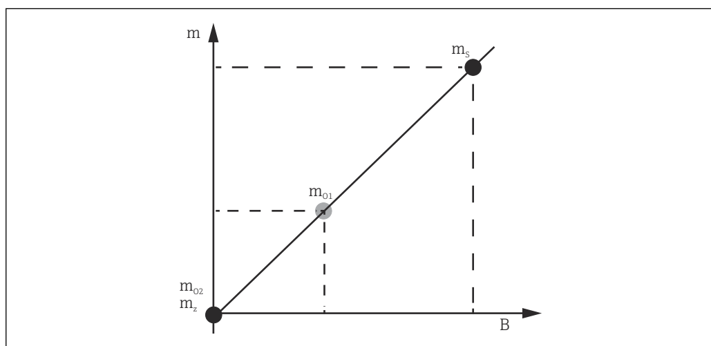
38 Концепция калибровки датчика
