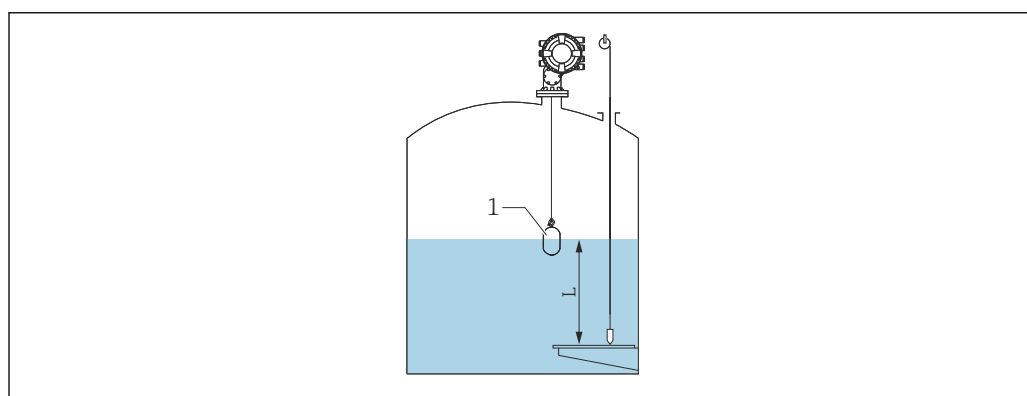
44 Установка уровня для открытого резервуара с жидкостью
