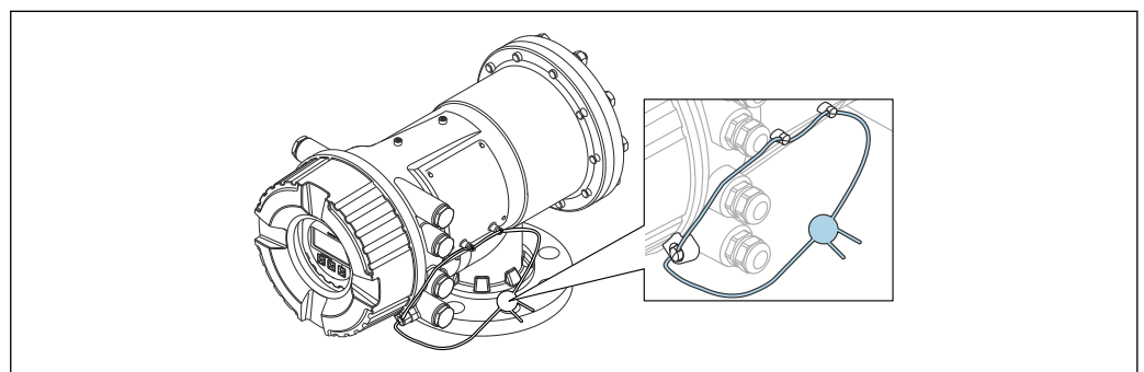
29 Versiegelung des Anschlussklemmenraumdeckels
