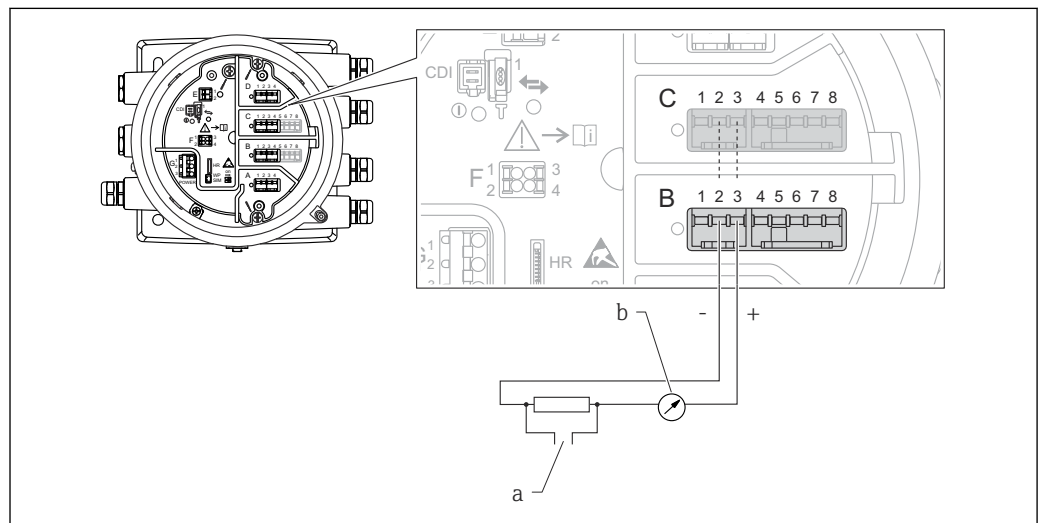
19 Aktive Nutzung des Analog I/O-Moduls im Ausgangsmodus
