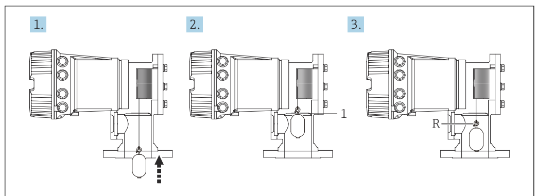
39 Ablauf Referenzkalibrierung
