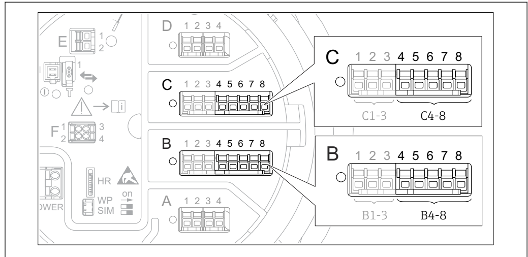
84 Klemmen für das Untermenü "Analog IP" ("B4-8" bzw. "C4-8")
