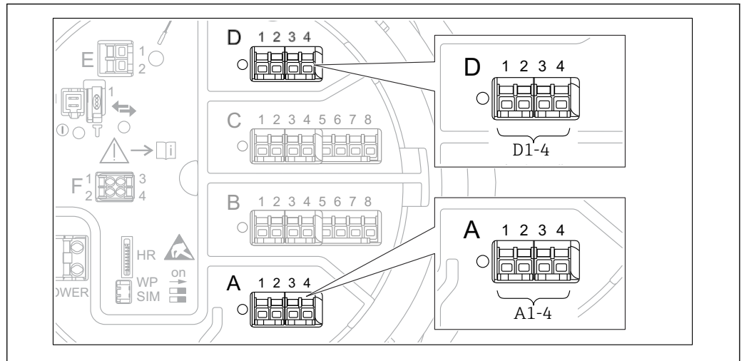
68 Mögliche Positionen der Modbus-Module (Beispiele); diese Module können je nach Geräteausführung auch in den Slots B oder C sitzen → 39 .
