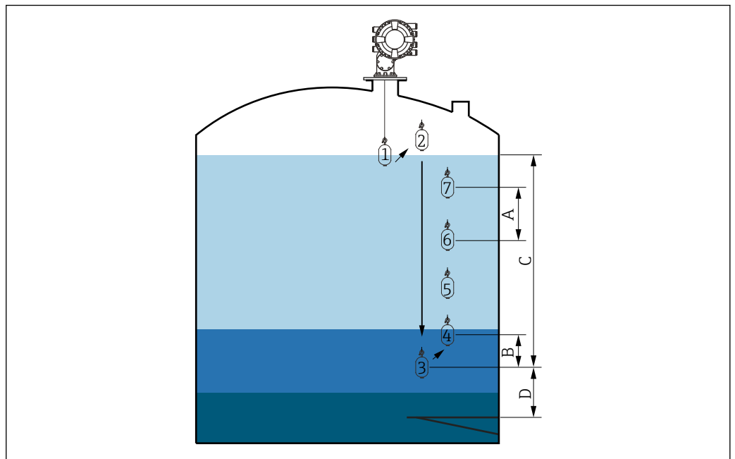
52 Bewegungsabfolge manuelle Profilmessung (die Zahlen zeigen die Abfolge der Verdrängerbewegung an)
