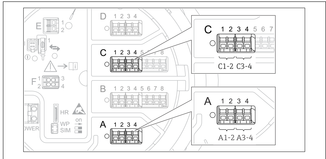
86 Bezeichnung der Digitaleingänge oder -ausgänge (Beispiele)
