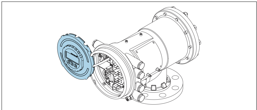
31 NMS83: Anzeigemodul steckt am Rand des Anschlussklemmenraums
