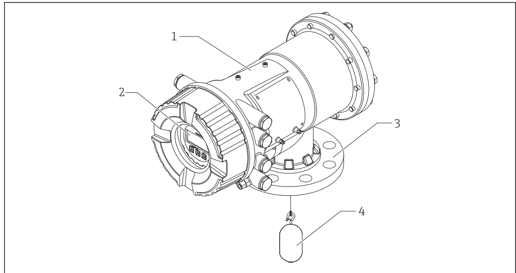
1 Aufbau des Proservo NMS83
