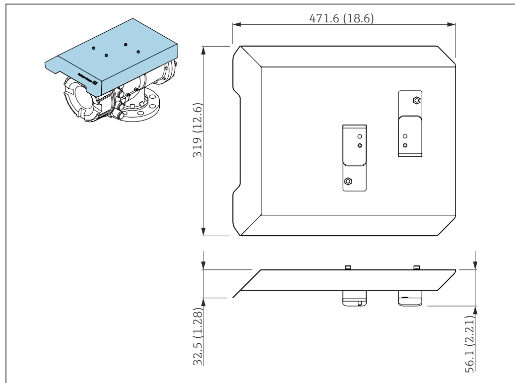
75 Wetterschutzhaube; Abmessungen: mm (in)
