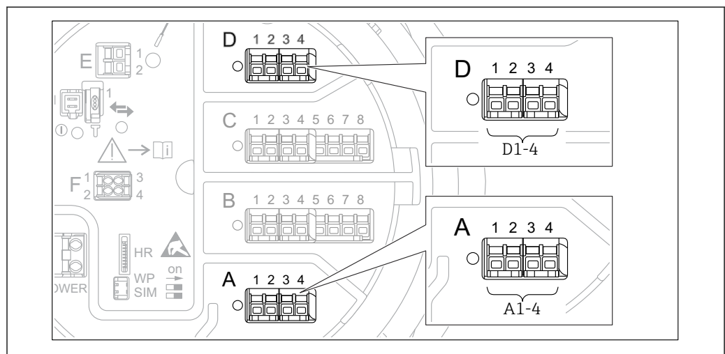
70 Mögliche Positionen der WM550-Module (Beispiele); diese Module können je nach Geräteausführung auch in den Slots B oder C sitzen → 39.
