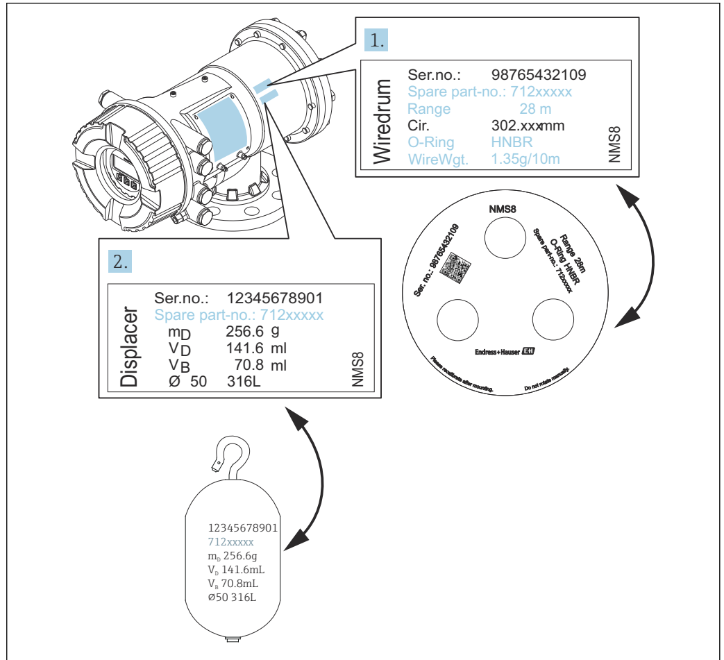
11 Verifizierung von Verdränger und Messtrommel
