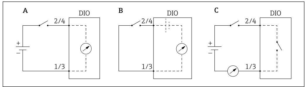
87 Betriebsarten des Digital I/O-Moduls
