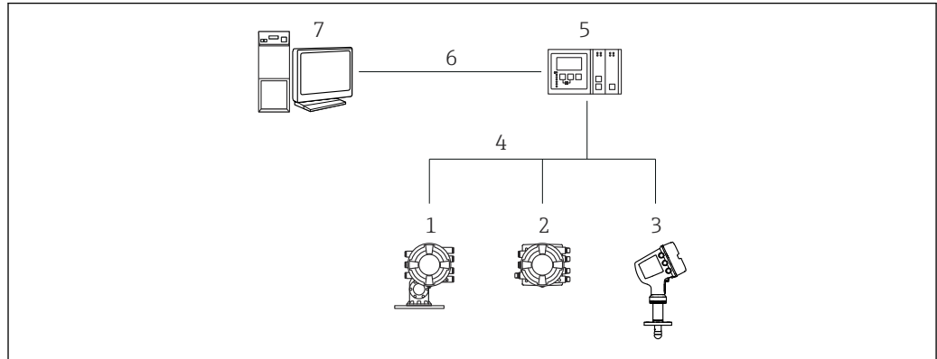
34 Anschluss von Tankstandmessgeräten an FieldCare über den Tankvision Tank Scanner NXA820
