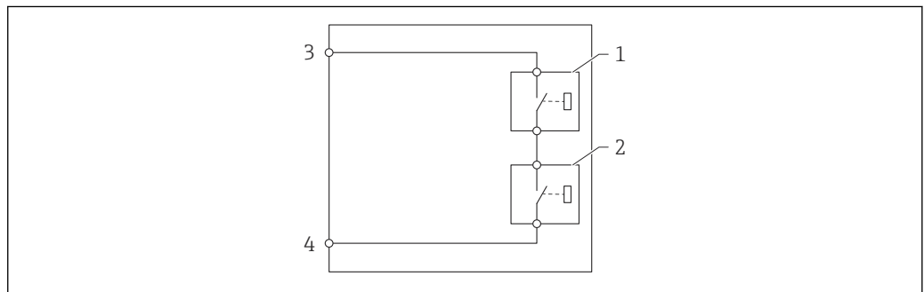
88 Die zwei Relais des Digitalausgangs
