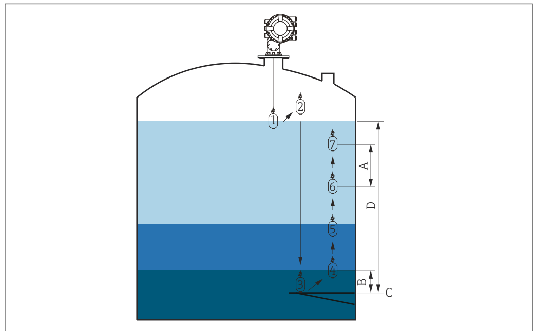
50 Bewegungsabfolge Tankprofil-Messung (die Zahlen zeigen die Abfolge der Verdrängerbewegung an)
