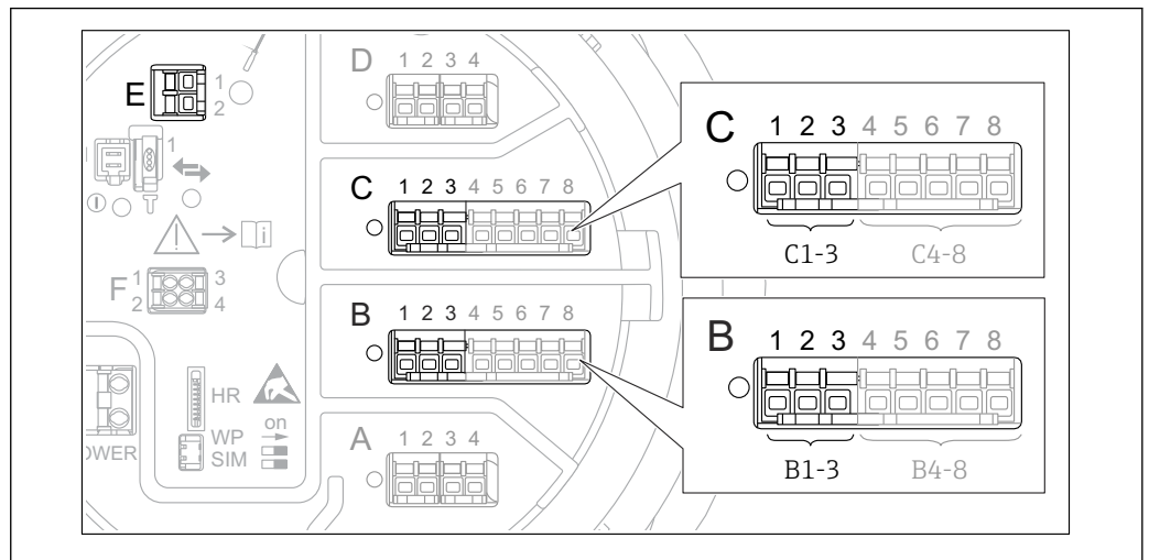
53 Mögliche Anschlüsse für HART-Schleifen
