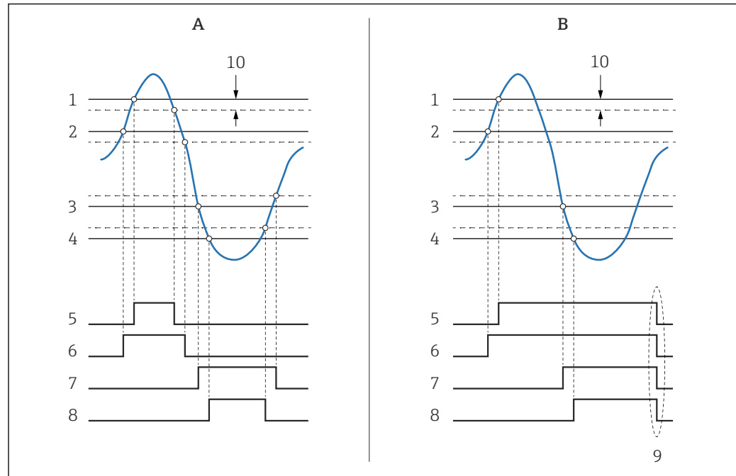
64 Prinzip der Grenzwertauswertung
