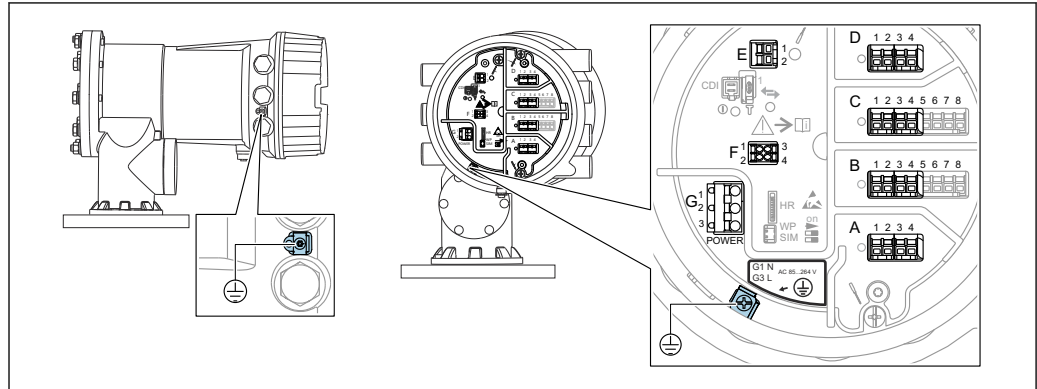
12 Anschlussklemmenraum (typisches Beispiel) und Erdungsklemmen
