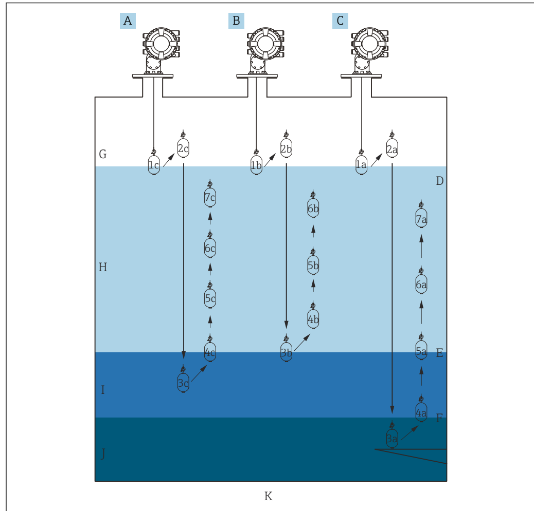
49 Übersicht über die Profildichte (1a, 2a, 3a ... zeigen die Abfolge der Verdrängerbewegung an)
