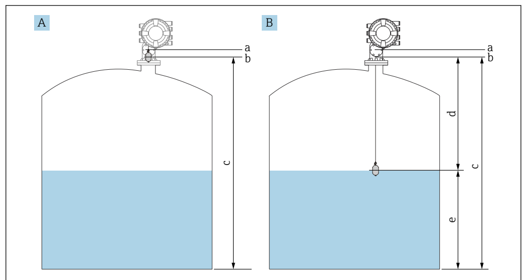
47 Einstellen des Füllstands bei Leerabgleich (NMS83)
