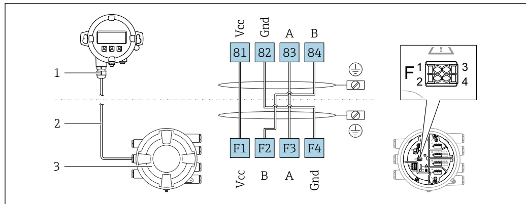
14 Anschluss des abgesetzten Anzeige- und Bedienmoduls DKX001 an das Tankstandmessgerät (NMR8x, NMS8x oder NRF8x)
