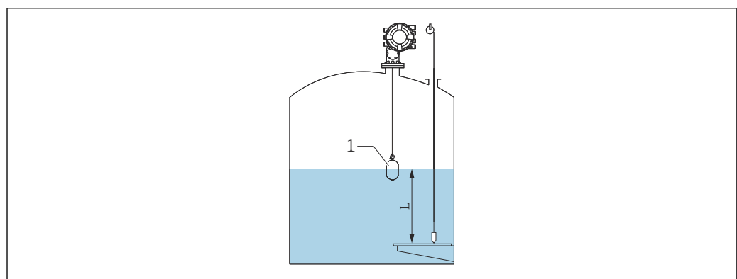
44 Füllstand für offenen Tank mit Flüssigkeit einstellen
