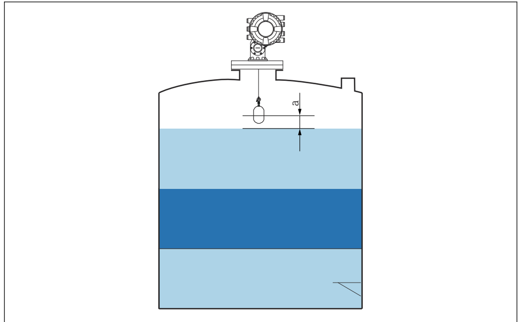
83 a: Offset Standby Distanz
