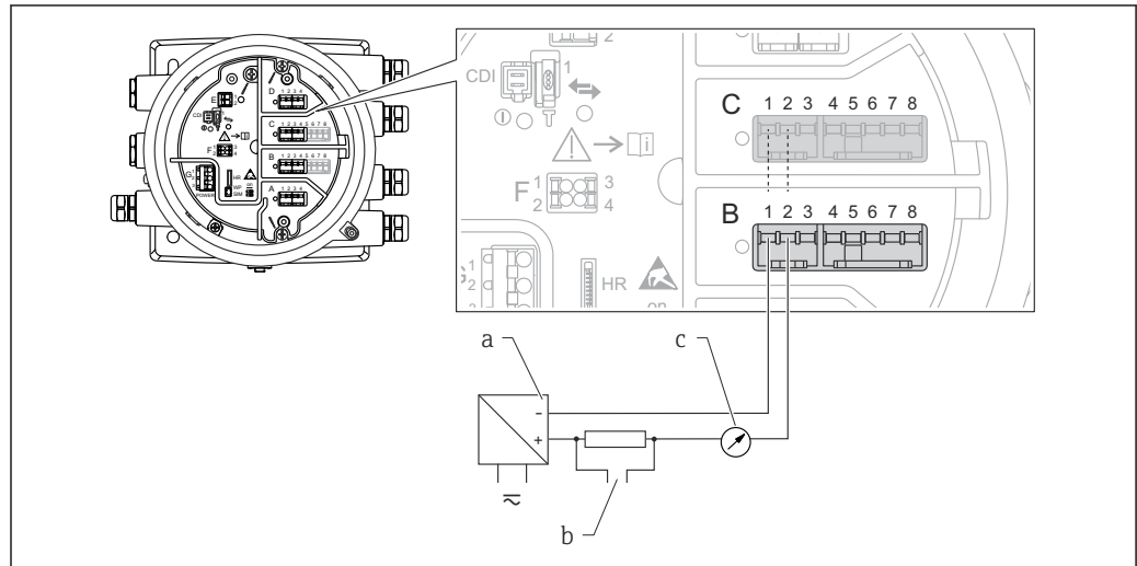
16 Passive Nutzung des Analog I/O-Moduls im Ausgangsmodus
