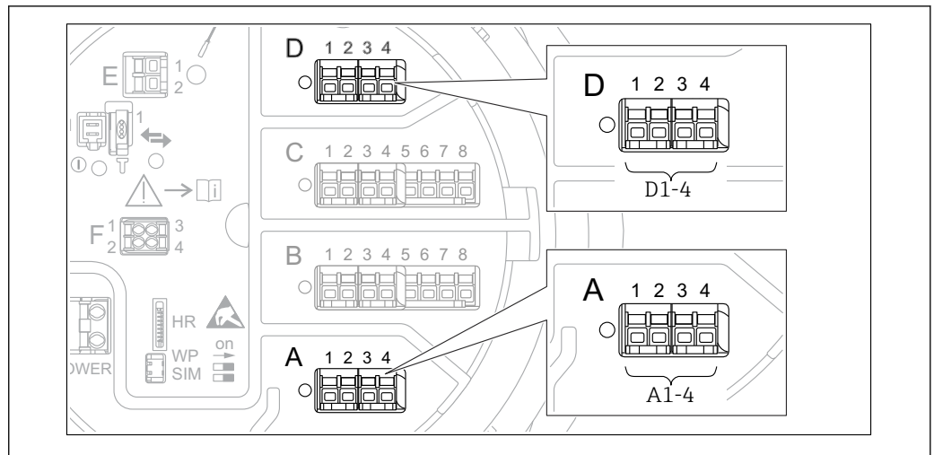
15 Bezeichnung der "Modbus"-, "V1"- oder "WM550"-Module (Beispiele); diese Module können je nach Geräteausführung auch in den Slots B oder C sitzen.
