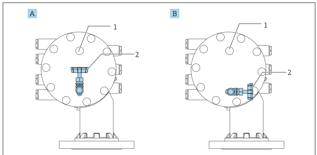
80 Reinigungsdüse und Überdruckventil
