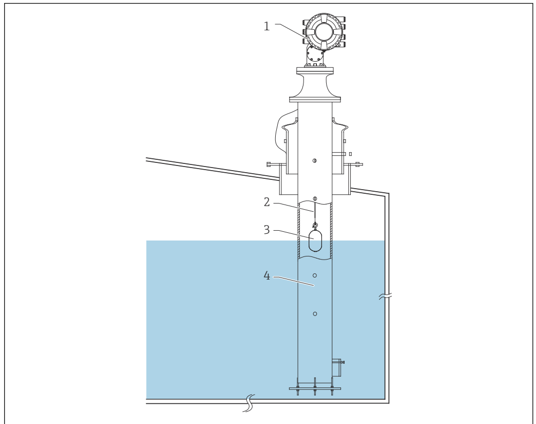
4 Typische Tankmontage 1
