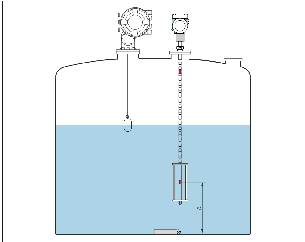
54 Prothermo NMT53x: Position des unteren Temperaturelements
