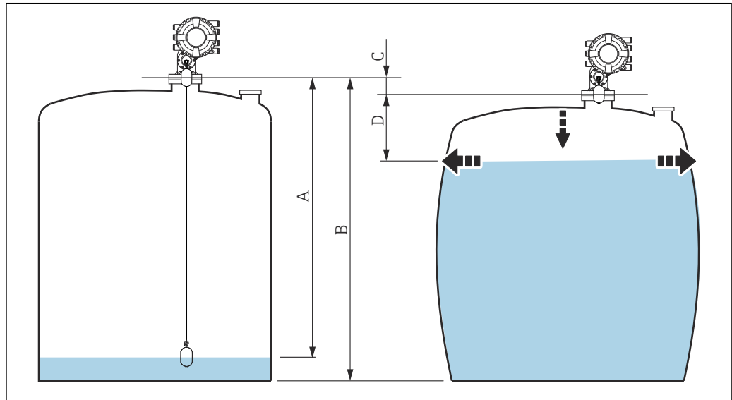
61 Korrektur der hydrostatischen Tankdeformation (HyTD)
