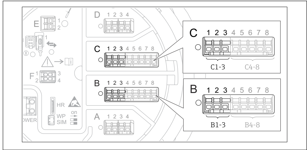
85 Klemmen für das Untermenü "Analog I/O" ("B1-3" bzw. "C1-3")
