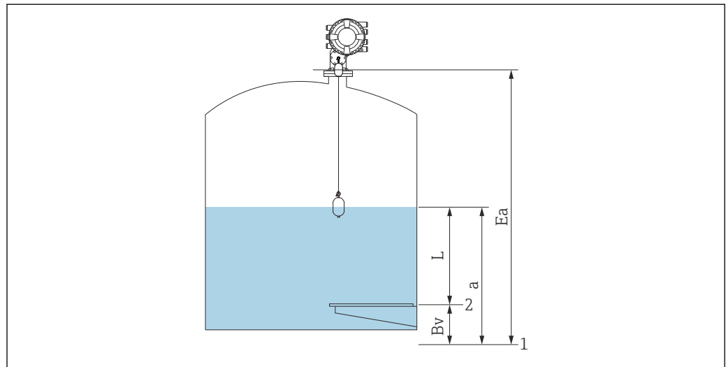
46 Geschlossener Tank für NMS83
