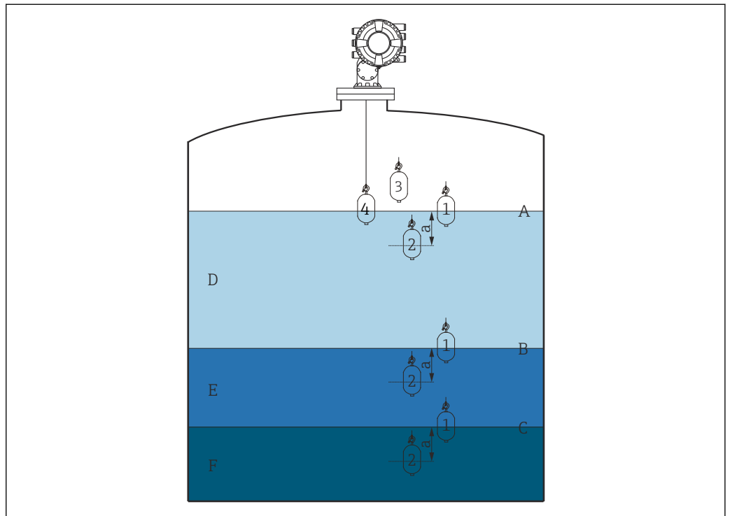
48 Punktdichte (die Zahlen zeigen die Abfolge der Verdrängerbewegung an)
