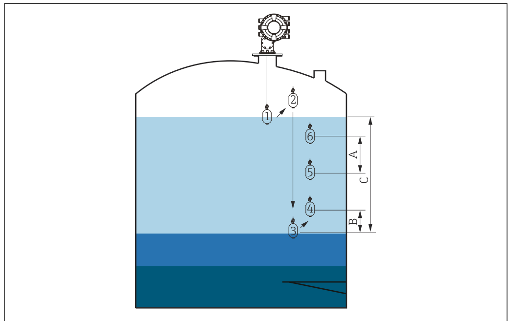
51 Bewegungsabfolge Trennschichtprofil-Messung (die Zahlen zeigen die Abfolge der Verdrängerbewegung an)
