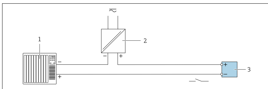
18 Пример подключения для релейного выхода (пассивного)
