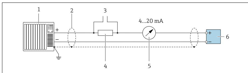
20 Пример подключения токового выхода 4–20 мА HART (активного)
