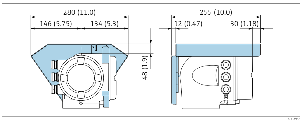
12 Защитный козырек от погодных явлений для прибора Proline 500; единицы измерения – мм (дюймы)
